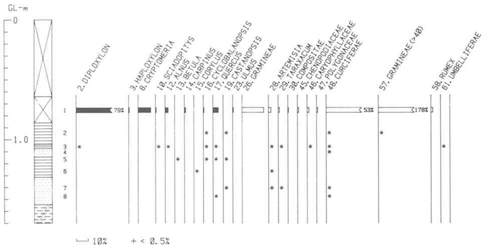
第28図 花粉ダイヤグラム
