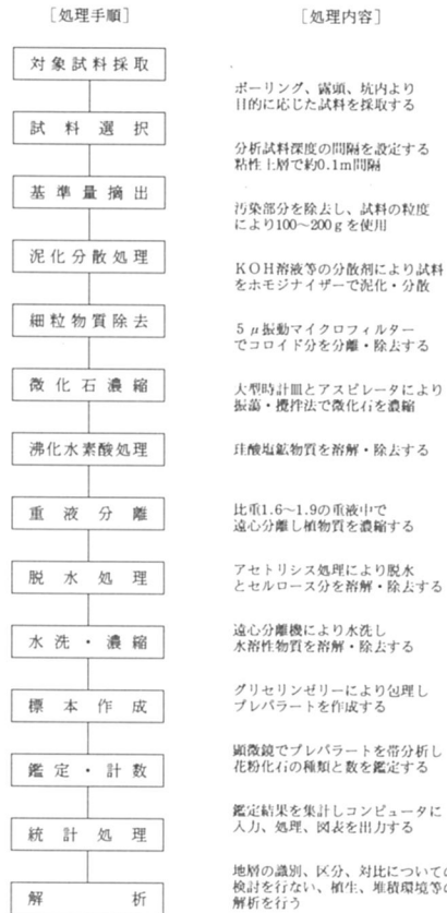
第27図 花粉分析フロー
