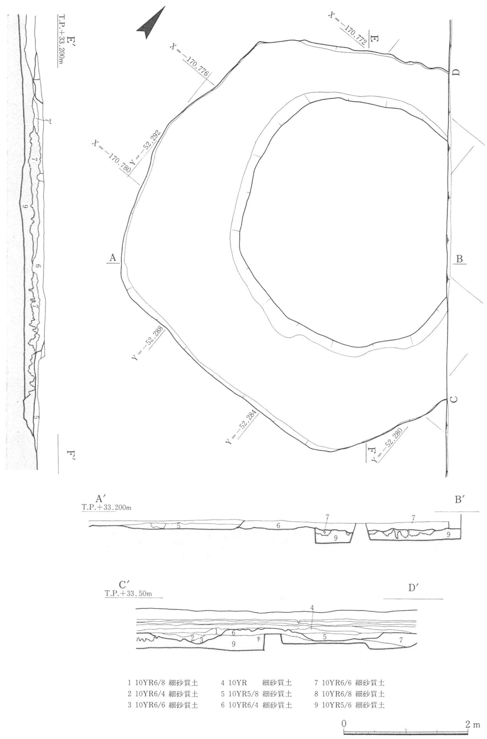
図版四十二 三三五—OG平・断面図
