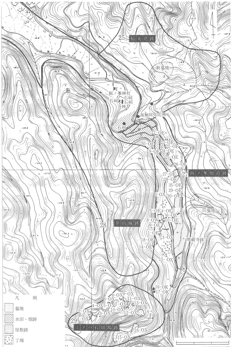
第57図 飯ノ峯畑遺跡遺構配置図
