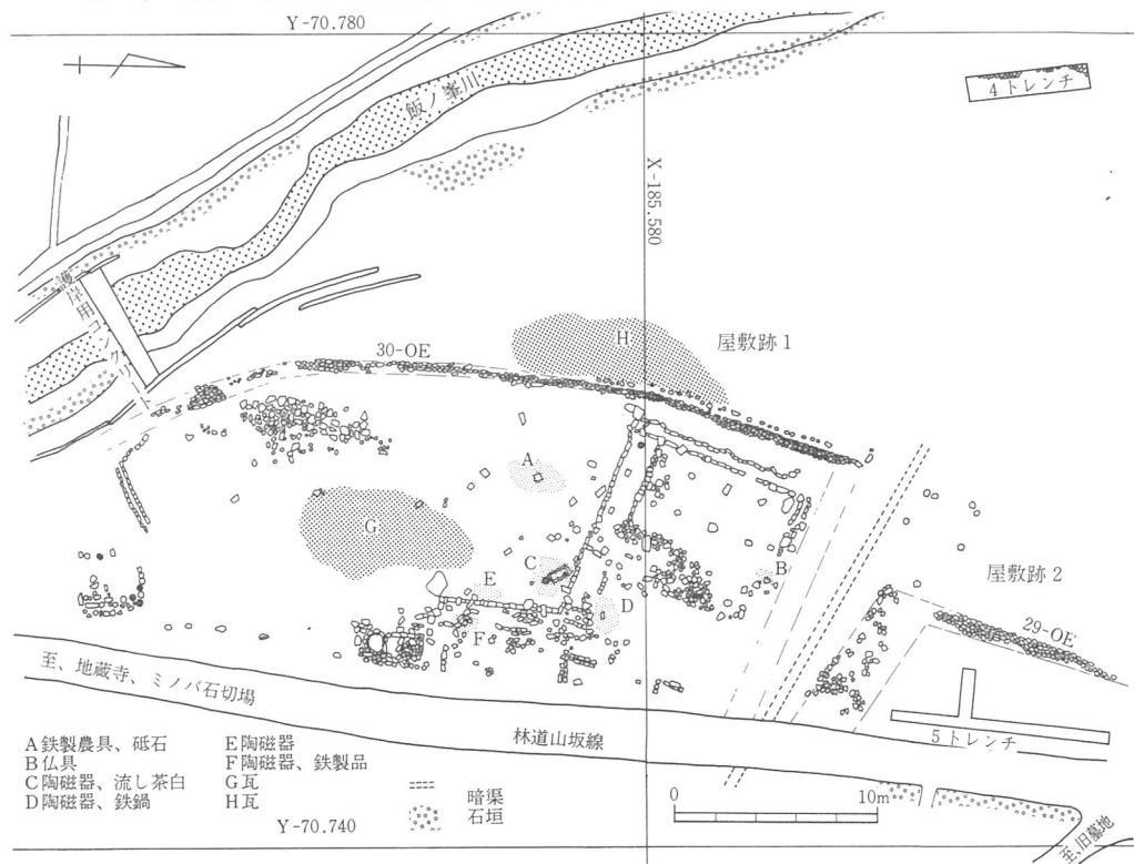
第58図 屋敷跡平面図
