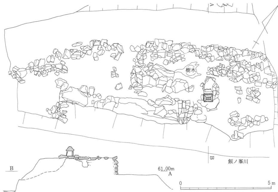
第53図 石祠4基壇実測図
