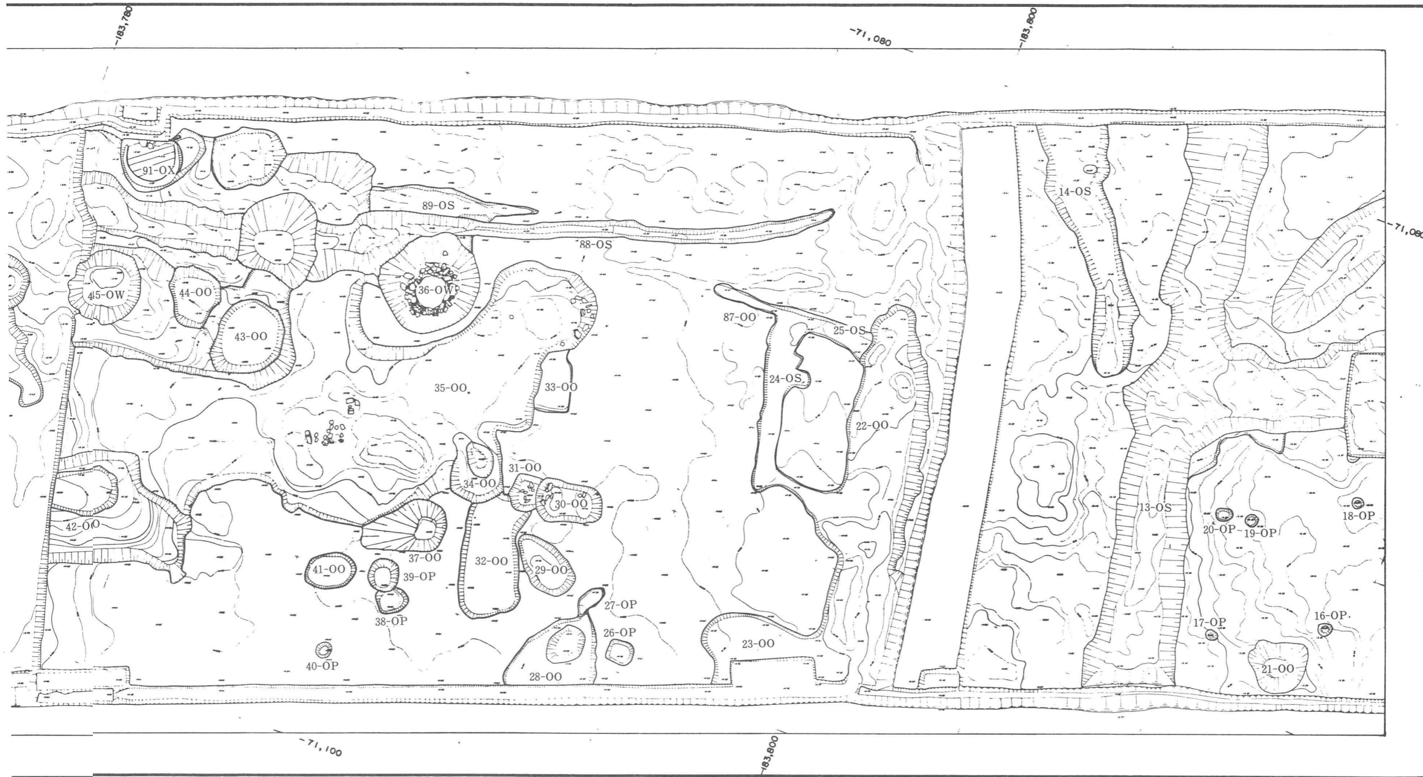
第8图 II区平面图3 (1:100)
