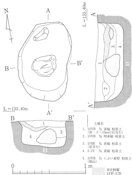
第7図 88-00実測図 (1/30)
