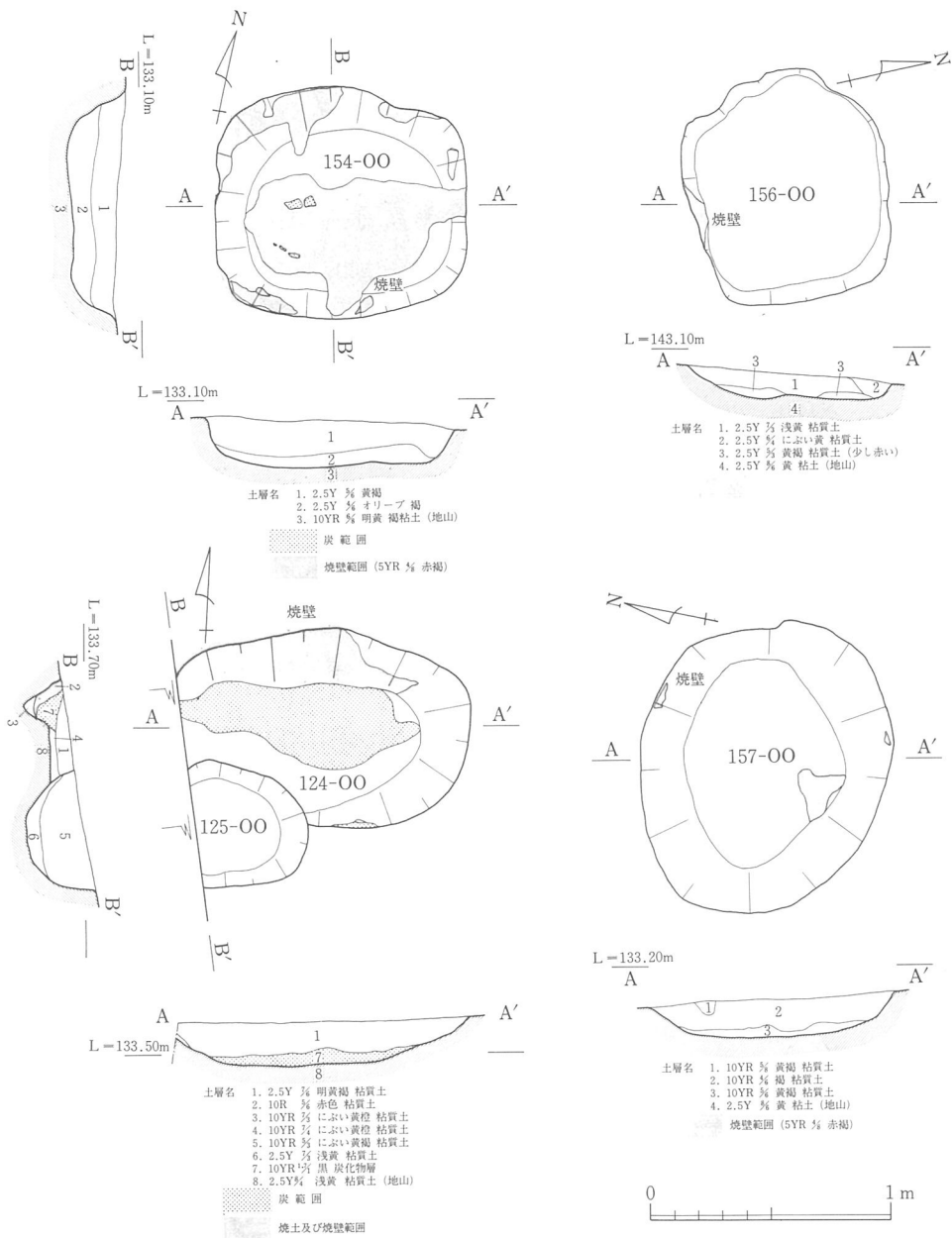
第8図 124-00, 125-00, 154-00, 156-00, 157-00実測図 (1/30)
