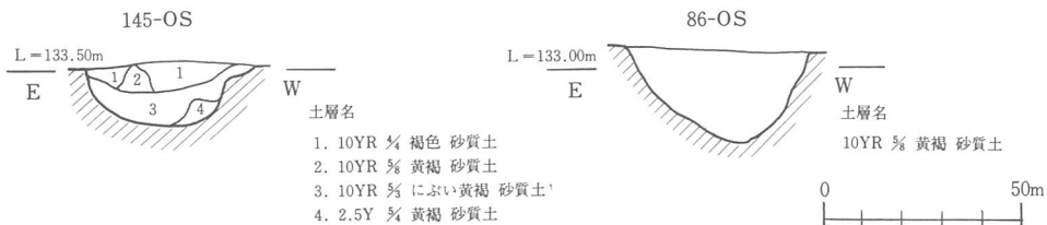
第5図 86-O S, 145-O S断面実測図 (1/20)
