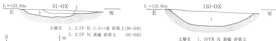
第10図 91-OX, 150-OX断面実測図 (1/40)
