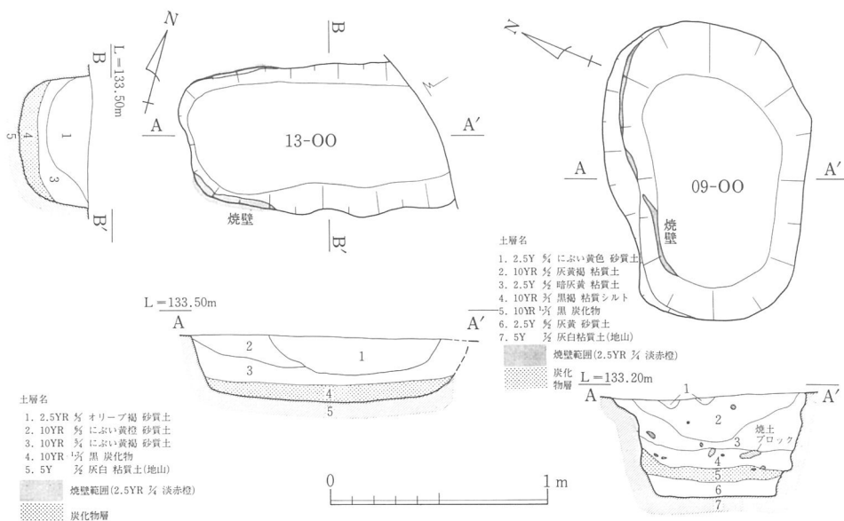
第6図 09-00, 13-00実測図 (1/30)
