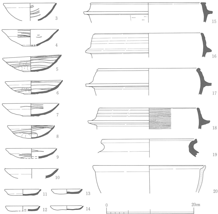
第12図 出土遺物実測図 (1/4)
