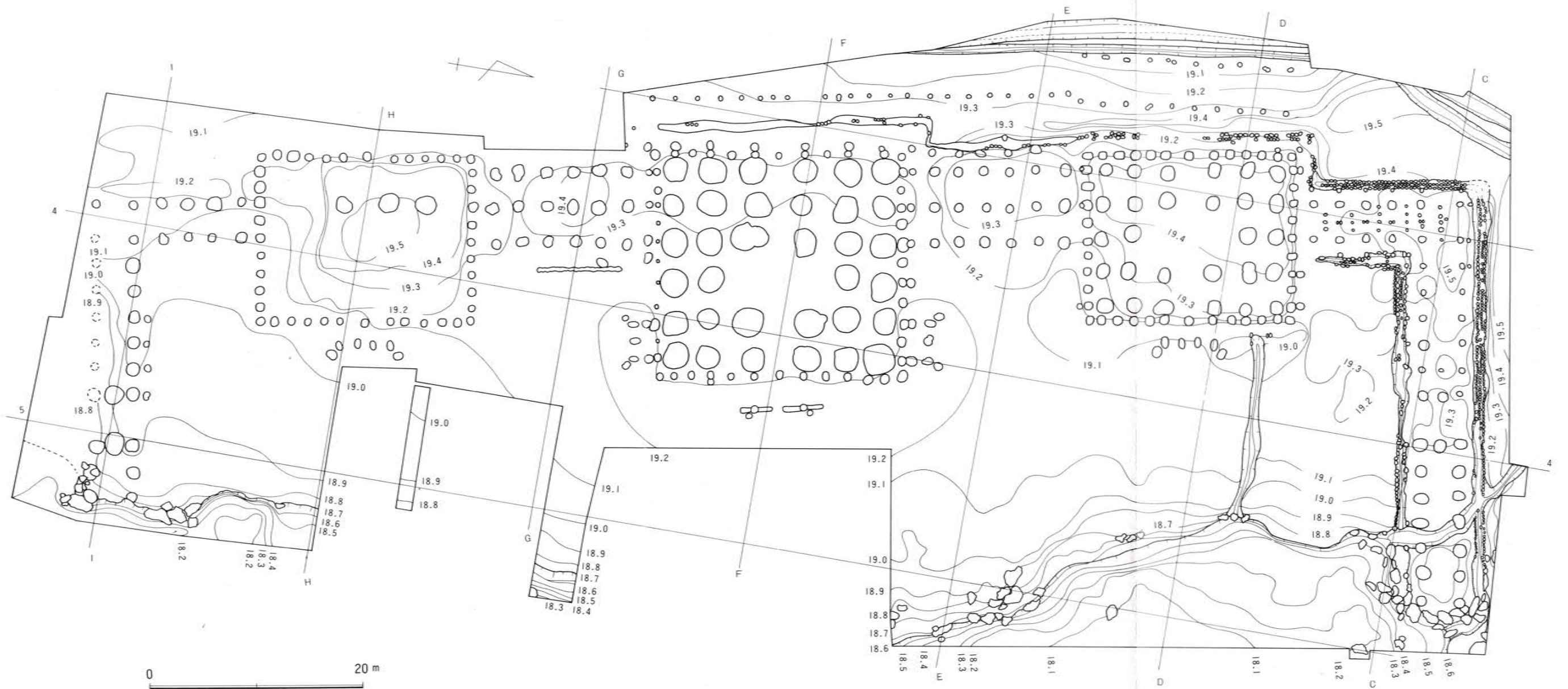
图3 遺構面地形測量図
