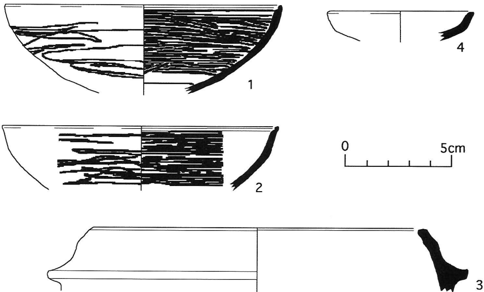
図22 出土遺物実測図。1・2:瓦器碗, 3:瓦器釜, 4:土師器皿
