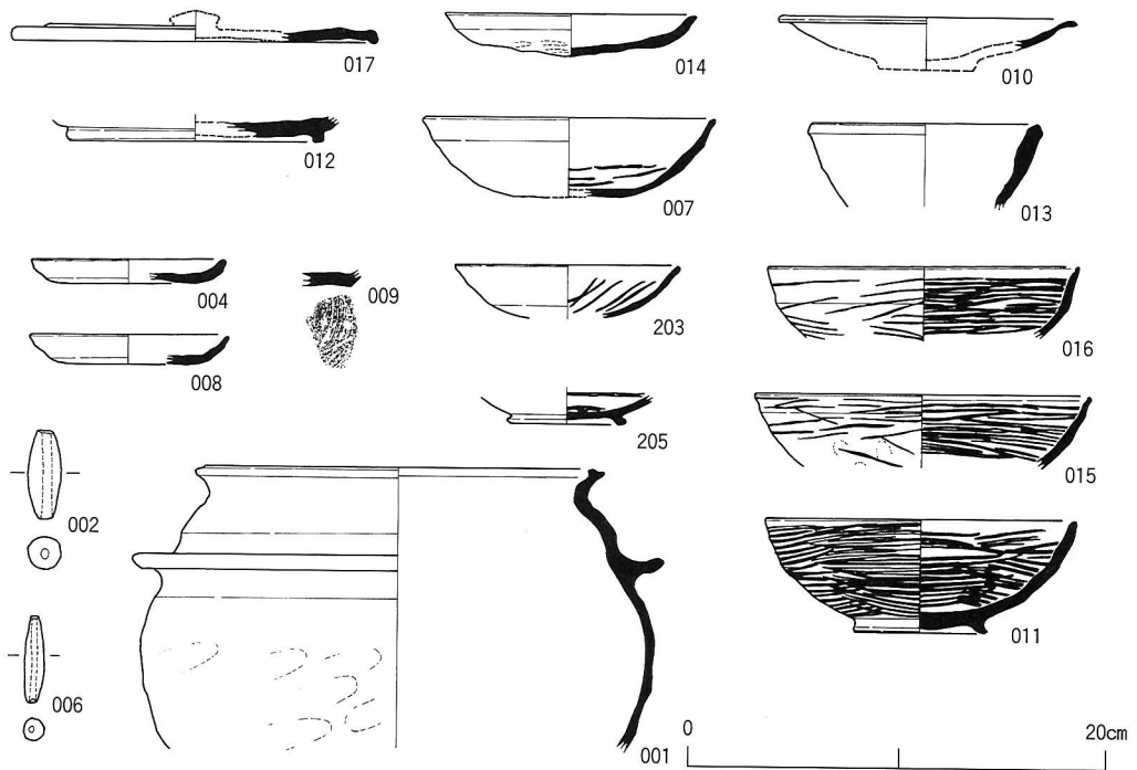
図8 柱穴・掘立柱建物1・3出土遺物実測図
