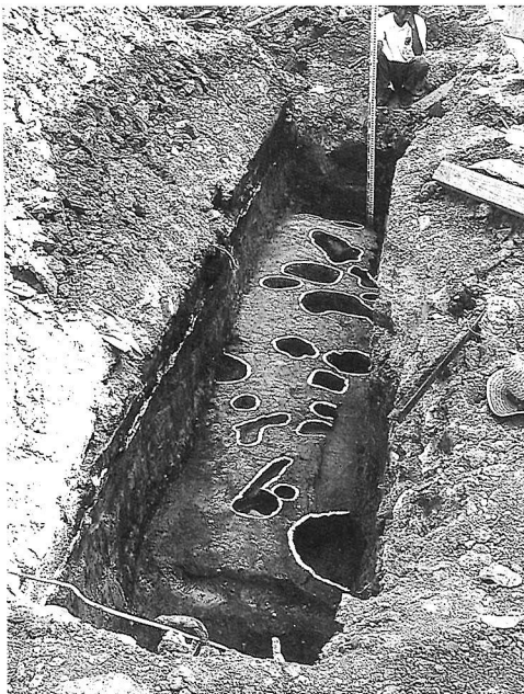
写真2 第3トレンチ、4層上面での中世遺構検出状況。北から南を撮影。手前中央のピットには根石が残る。4層の上面は本トレンチの南端部で低くなる。
