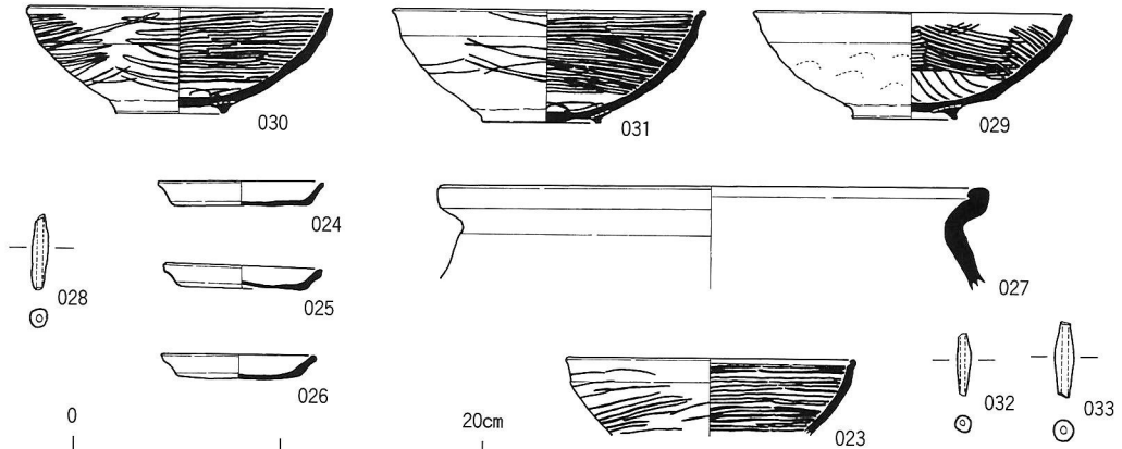
図11 土壇1・6・12・14出土遺物実測図
