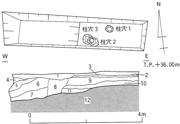
図17 B地区地山上面遺構平面図・北壁断面図
