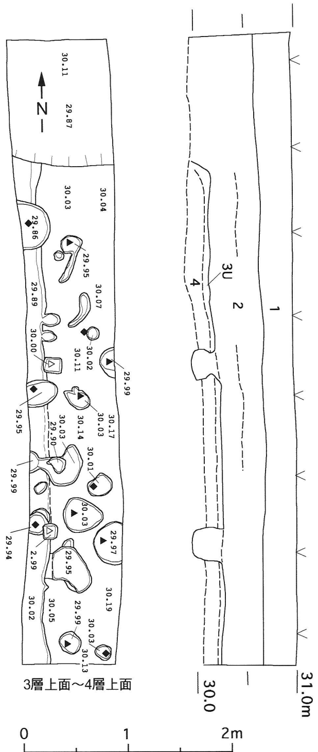
図20 第3トレンチの堆積層断面と遺構平面図
