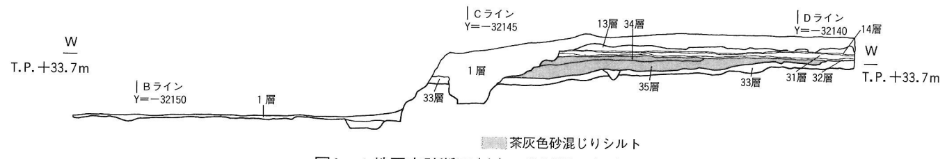
図4 A地区南壁断面(上) 北壁断面(下)
