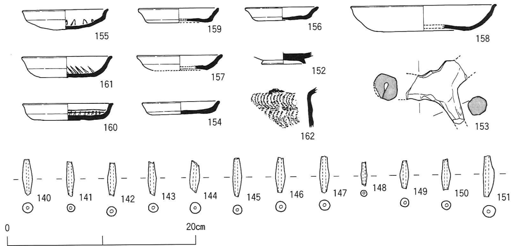
图16 第28层出土遗物实测图
