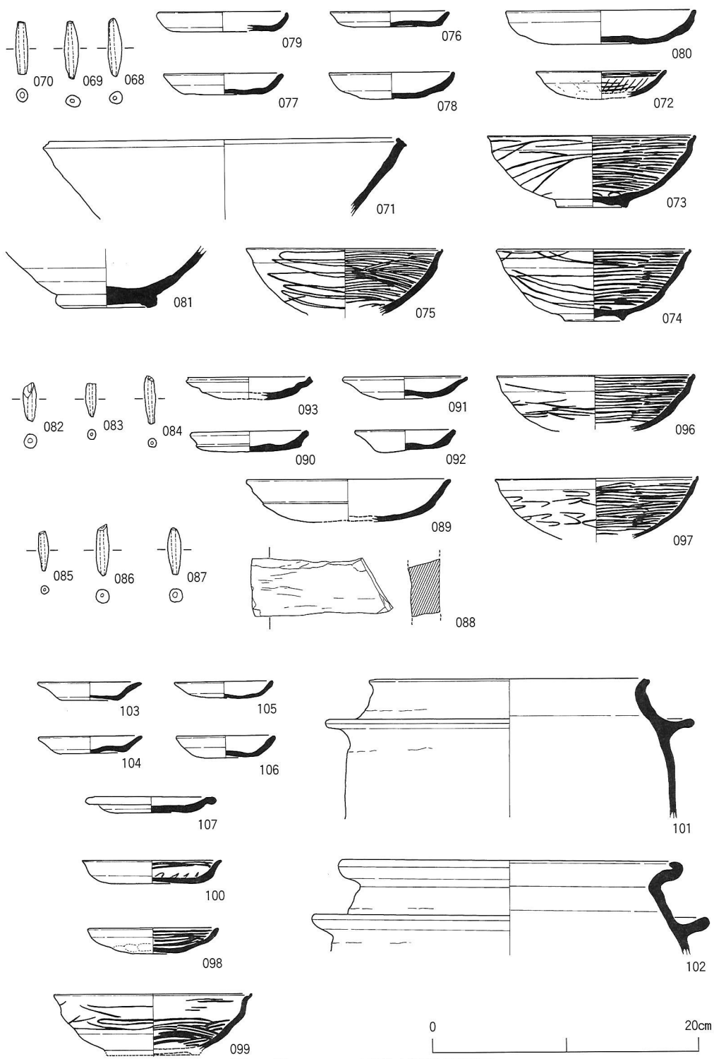
图9 溝29・35・36出土遺物実測図
