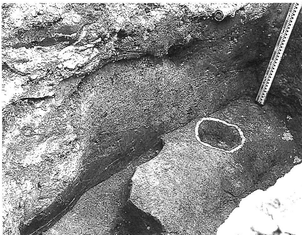
写真3 第2トレンチの堆積層断面(東壁)と4層上面での中世遺構検出状況。北西から南東を撮影。西落ちの段差が見られ、高い面でピットが検出された。写真手前の落ち込みは4層中の同時異相部分を掘削した跡で遺構ではない。
