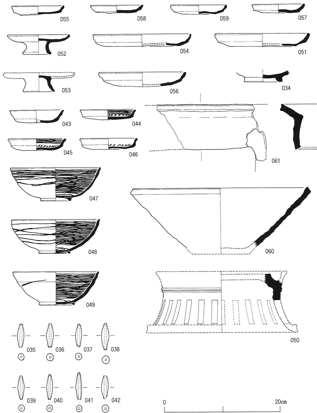
图12 土壤15出土遗物实测图
