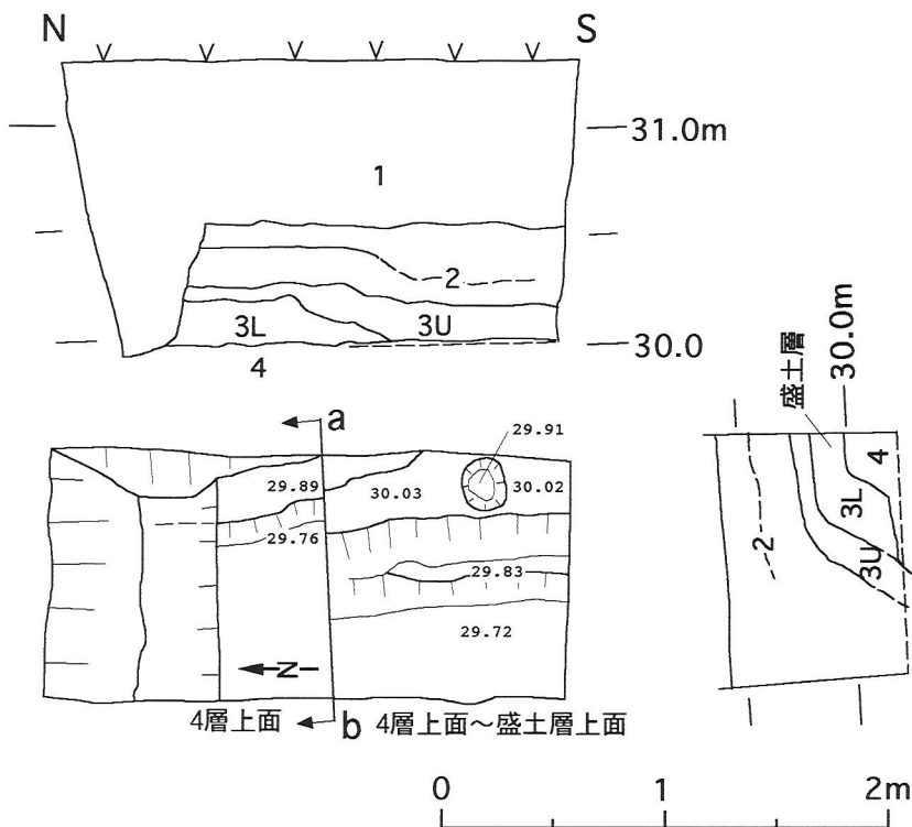
図21 第2トレンチの堆積層断面と遺構平面図
