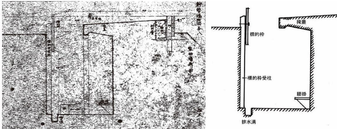
図 44. 射撃場附図第八 監的壕断面(左)と本断面の堀内(2017)による部分トレース図(右)
