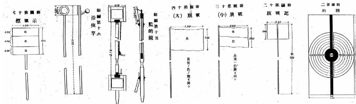
図 49. 『歩兵射撃教範』の射撃用具附図
