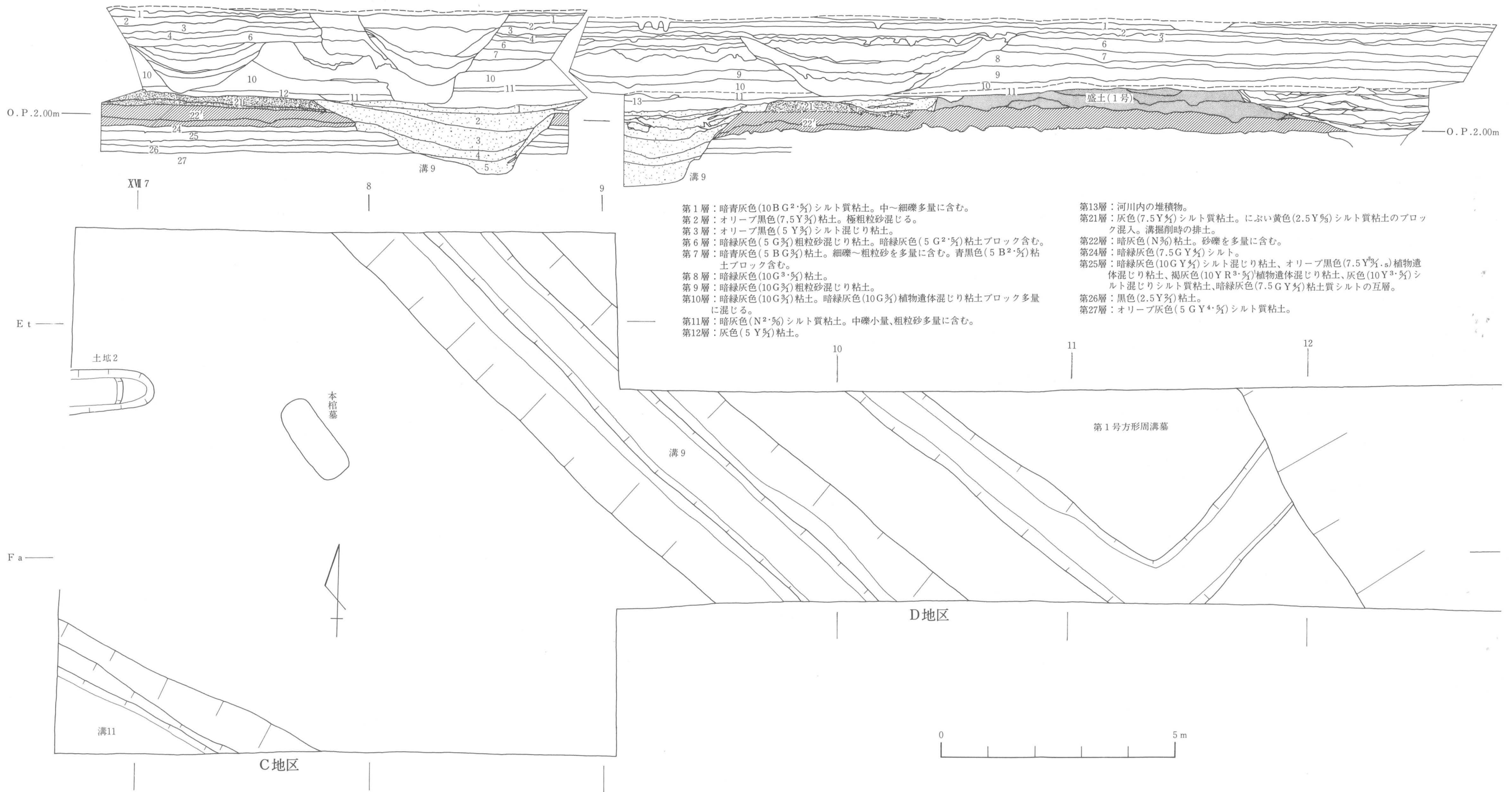
付図2. C・D地区遺構図・上層(1/100)
