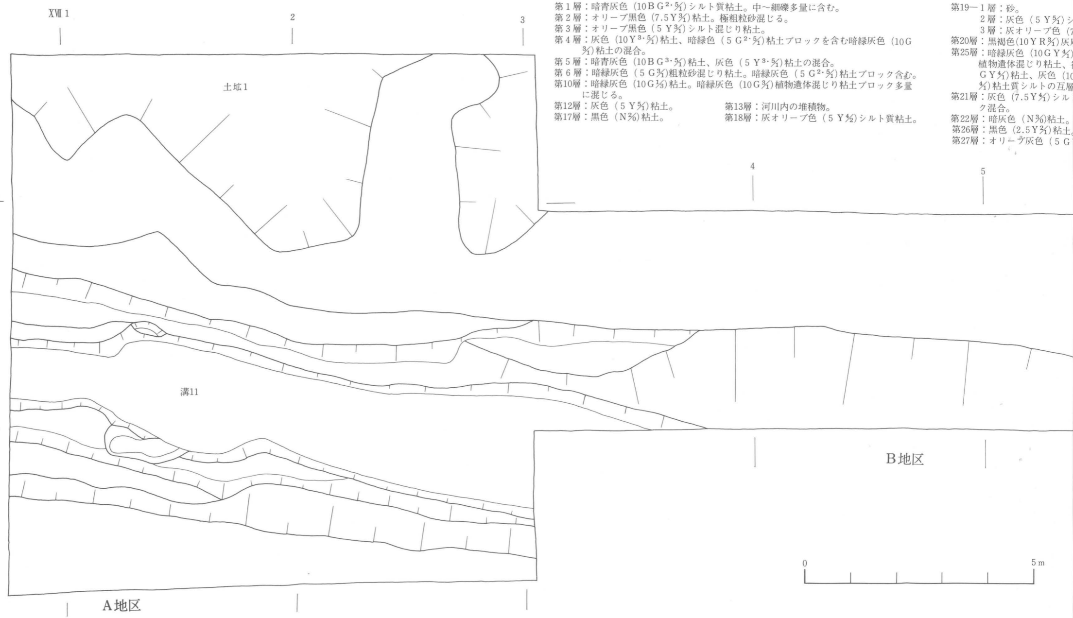
付図1. A・B地区遺構図・上層(1/100)
