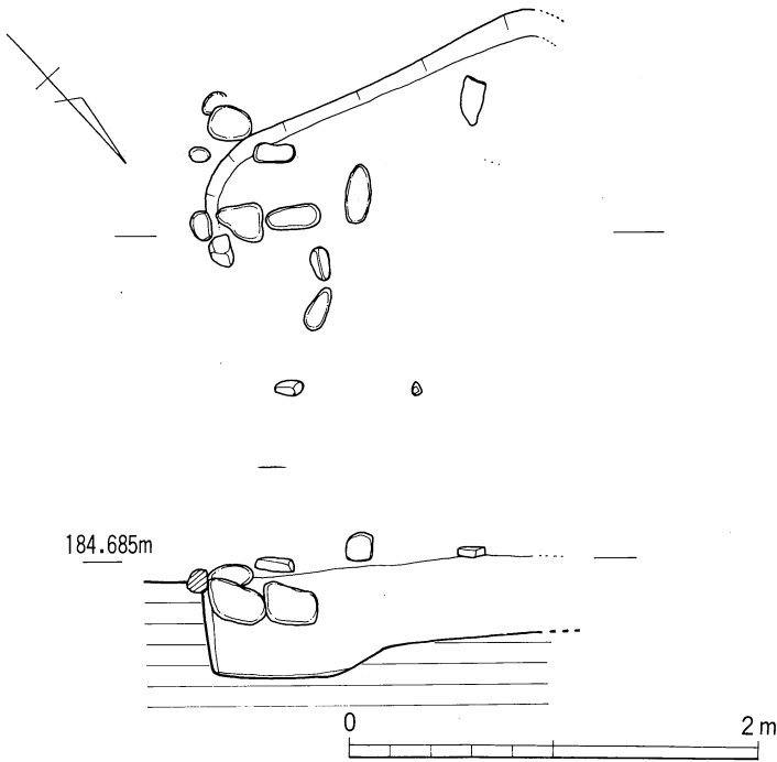
第22図 配石遺構実測図(1/40)
