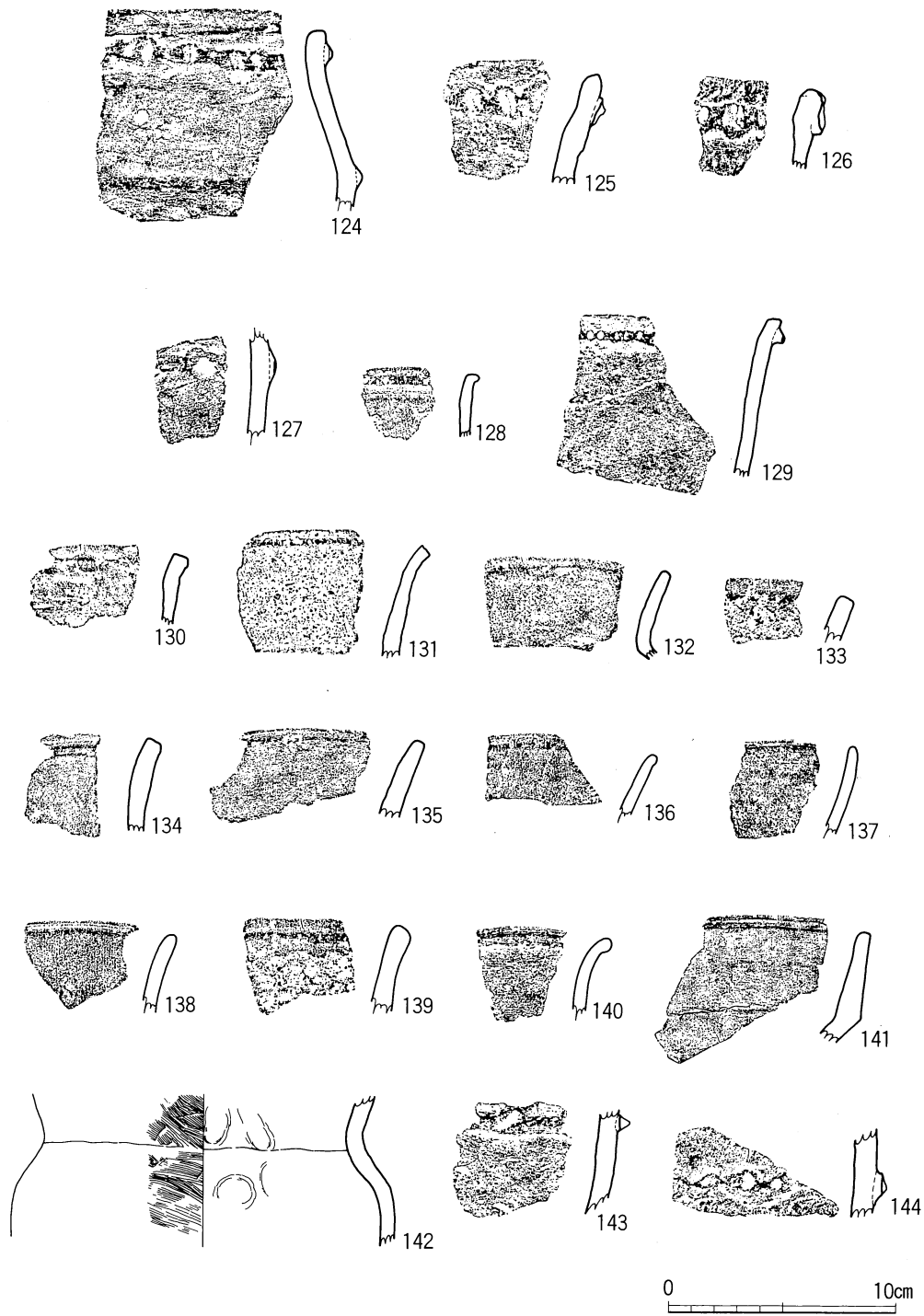
第31图 C区出土遗物实测图
