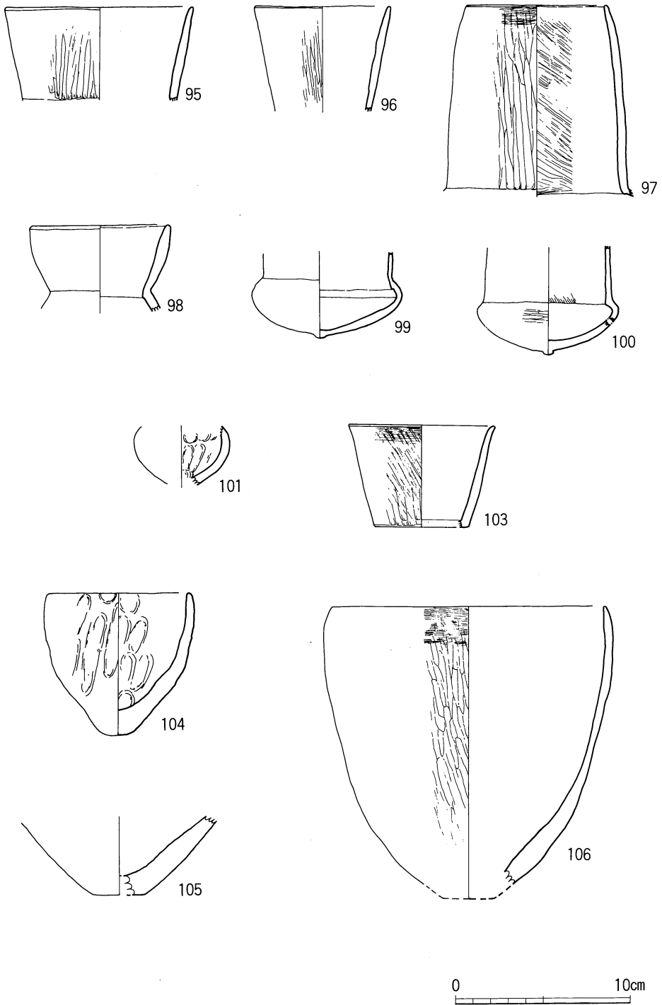
第26图 BK区出土遗物实测图(1/3)
