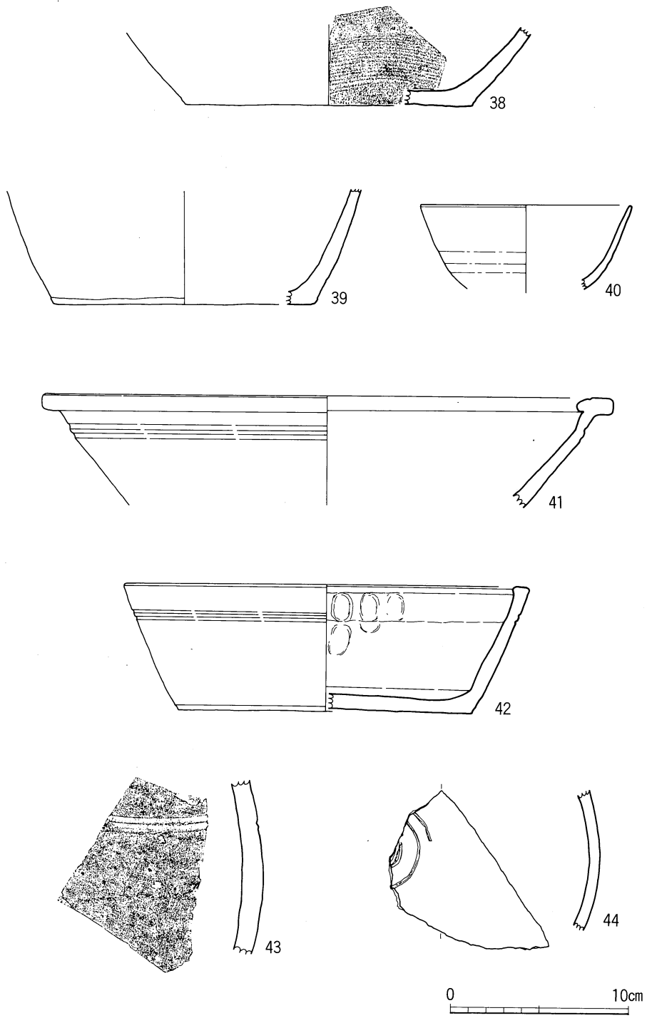
第12图 A区出土遗物实测图(1/3)
