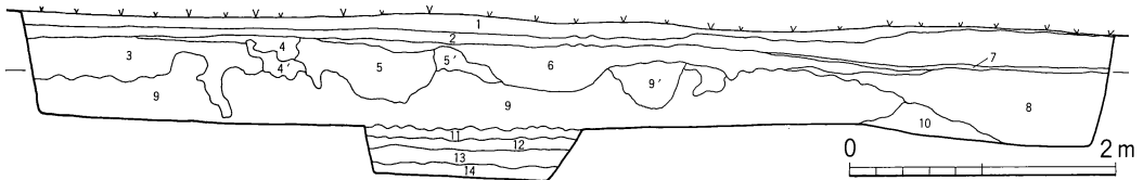
第4図 A区土層断面図
