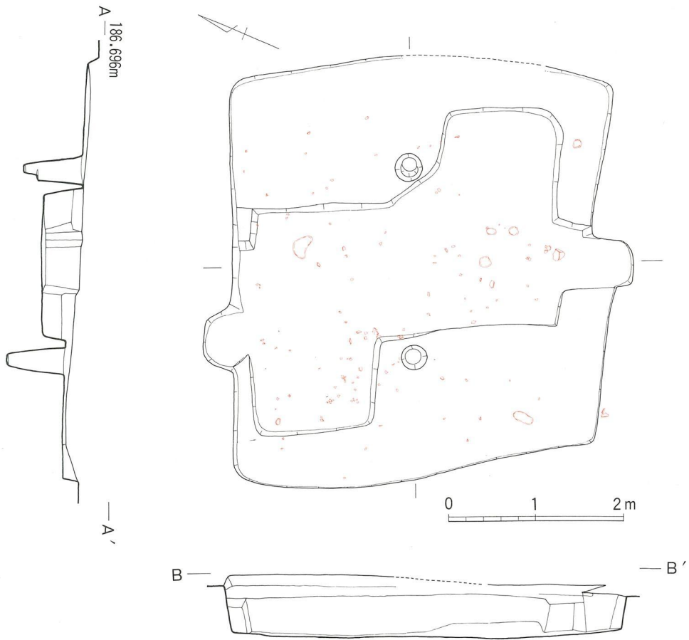
第28图 2号竖穴住居实测图
