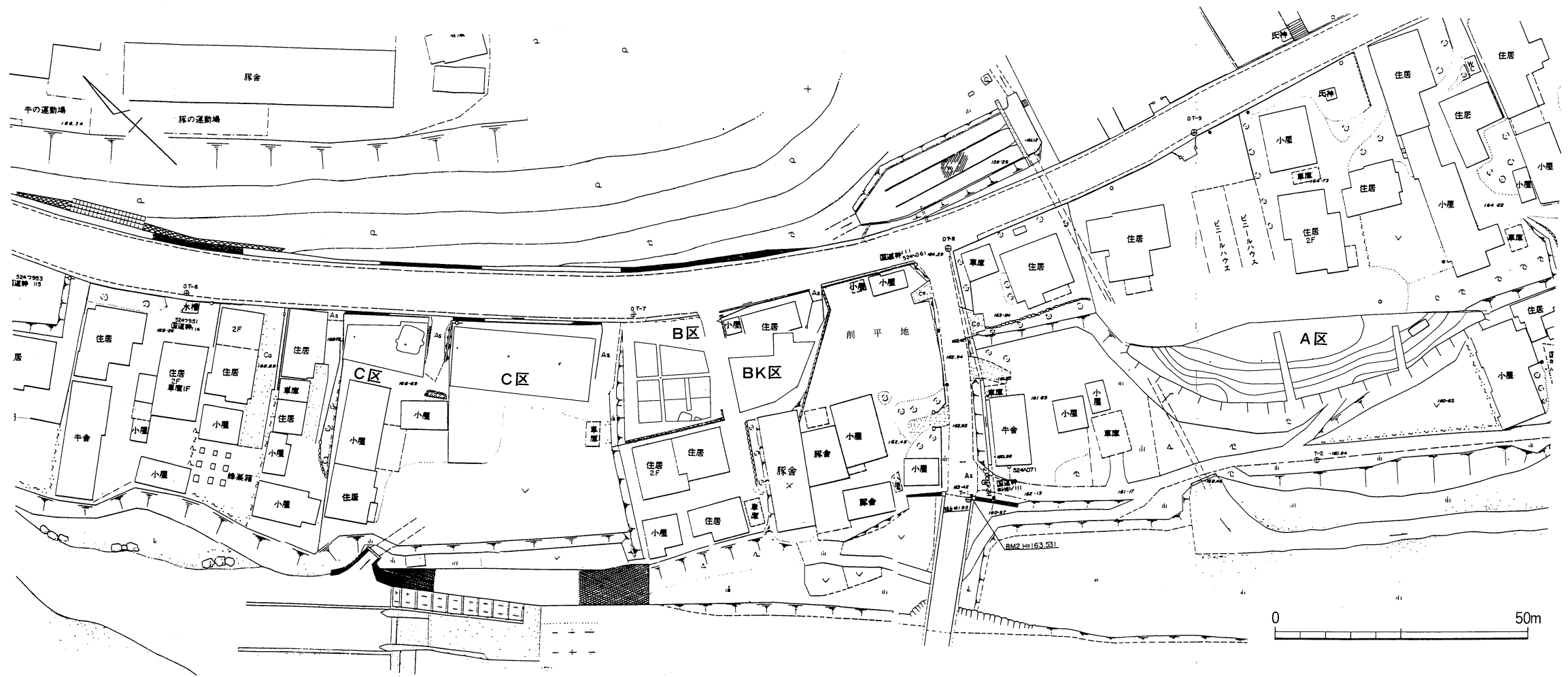
第1図 様屋敷遺跡発掘調査区(A・B・C・BK区) (1/500)
