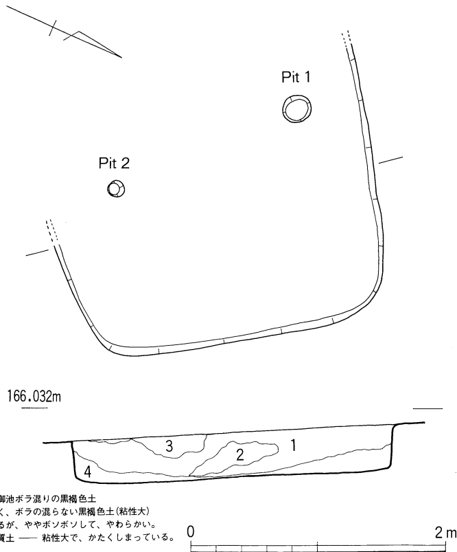
第16図 1号竪穴住居実測図
