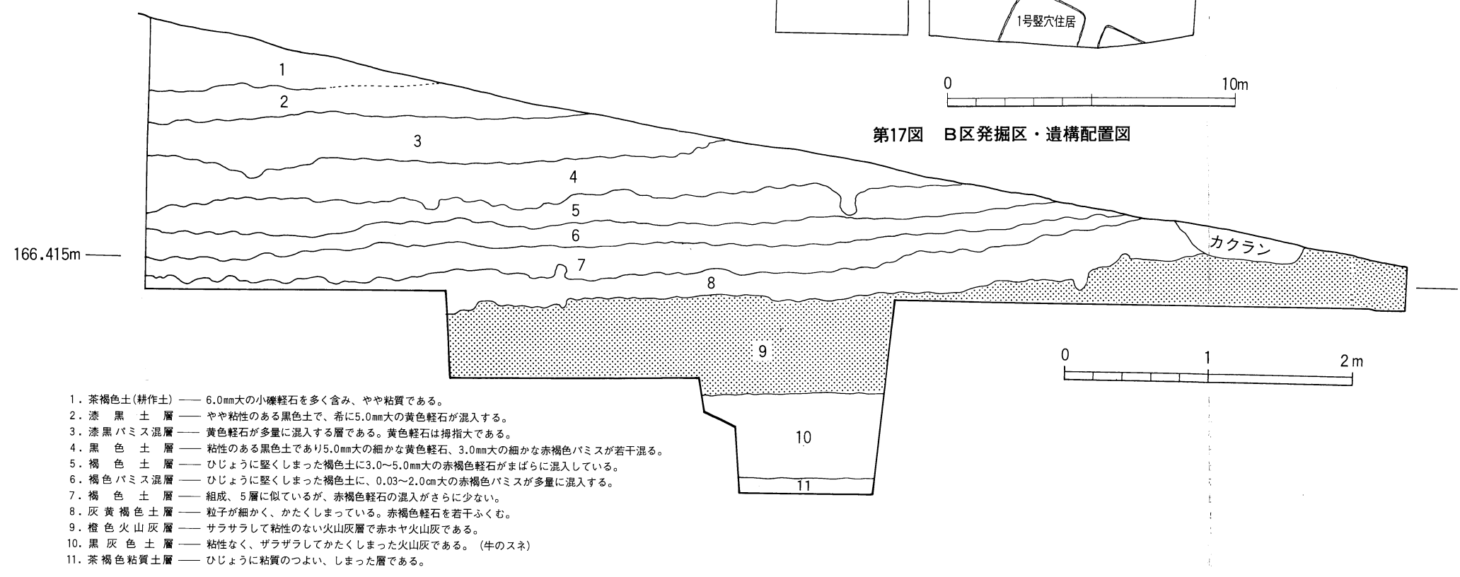
第18図 様屋敷遺跡(B区)基本土層断面図
