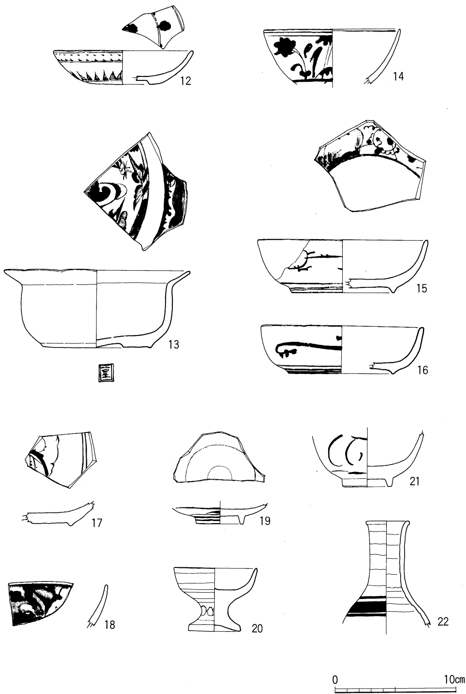
第9图 A区出土遗物实测图(1/3)
