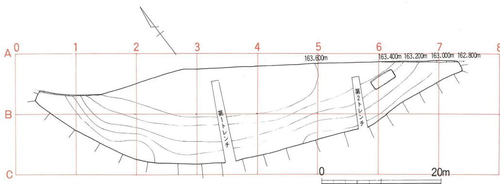
第2図 A区発掘区
