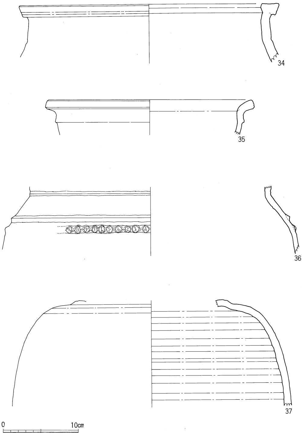
第11图 A区出土遗物实测图(1/3)
