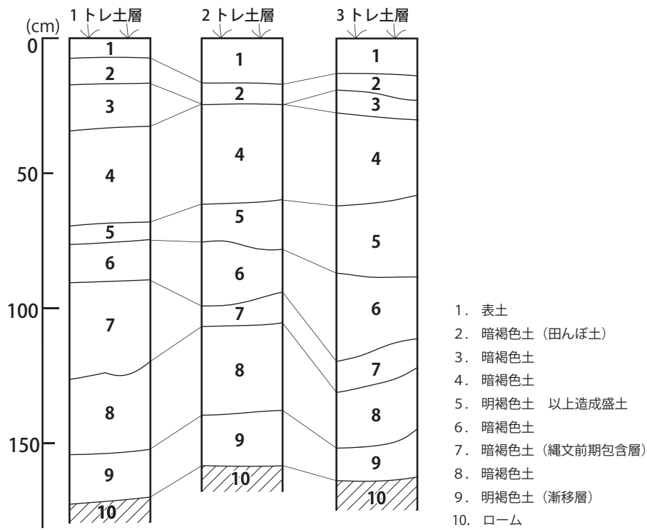
第7図 土層図 (1/20)
