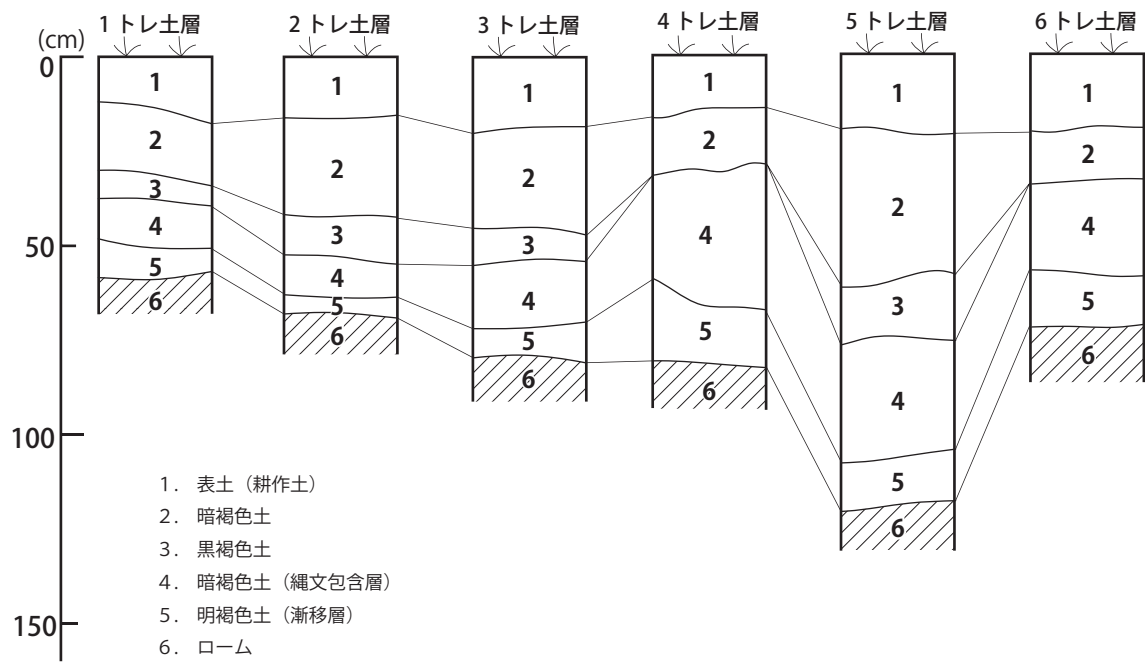
第3図 トレンチ配置図 (1/300)・土層図 (1/20)
