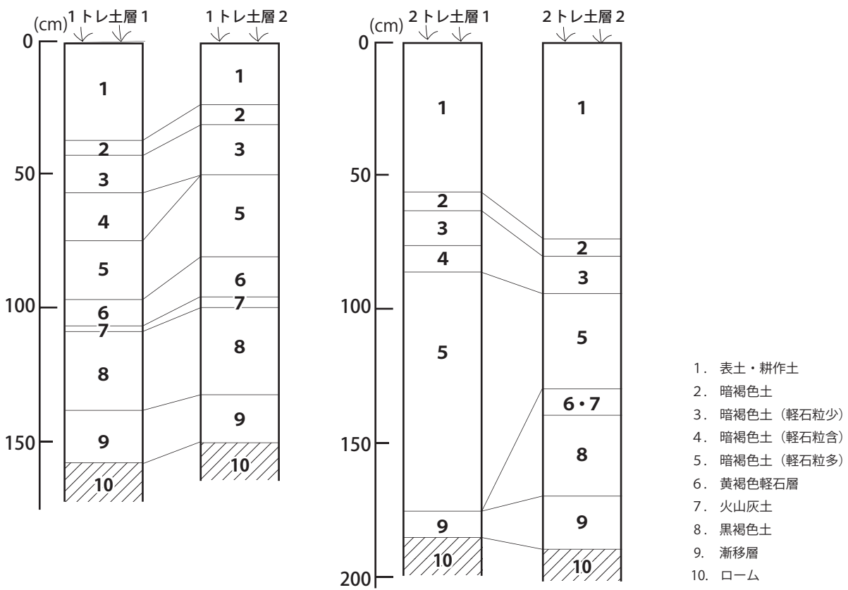
第12図 トレンチ配置図 (1/200)・土層図 (1/20)
