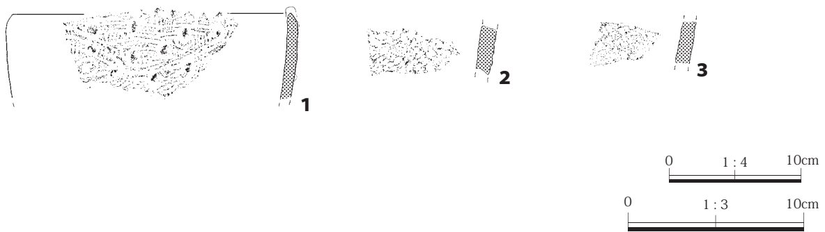
第8図 洞口遺跡出土遺物実測図 (1/4・1/3)
