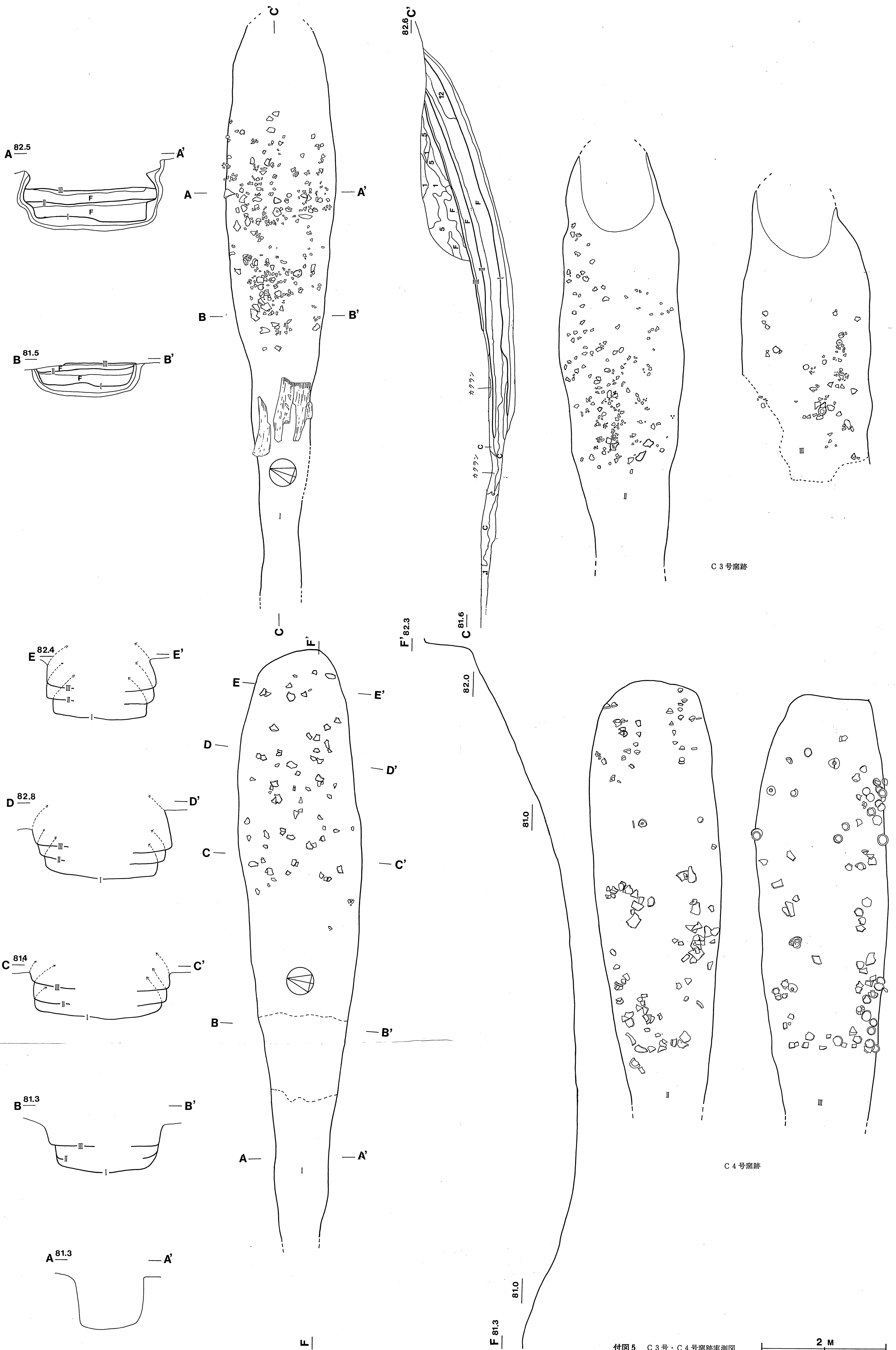
付図5 C3号・C4号窯跡実測図
