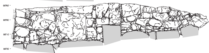
図 28 玄門立柱構造の大型横穴式石室の変遷 (母神山・大野原古墳群)
