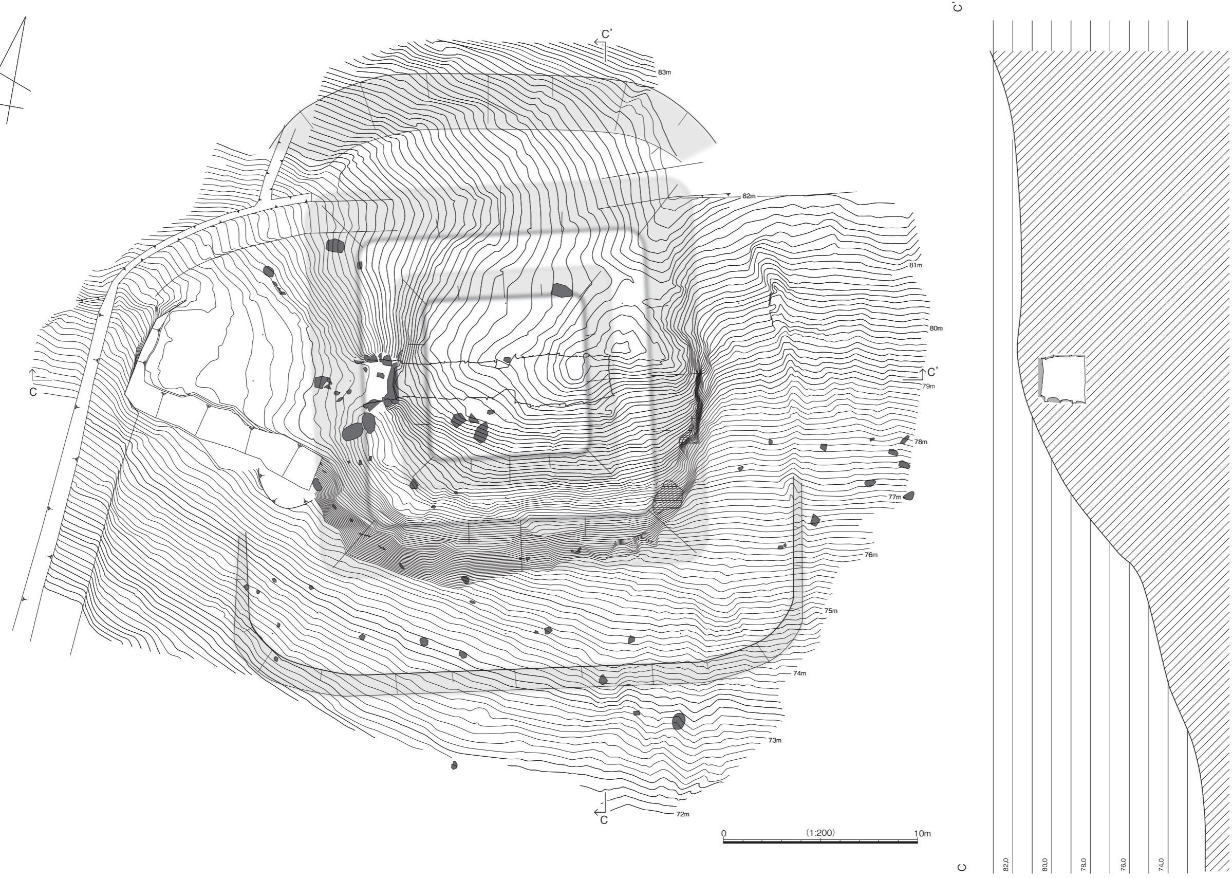
図 18 穴葉師（綾織塚）古墳墳丘測量図
