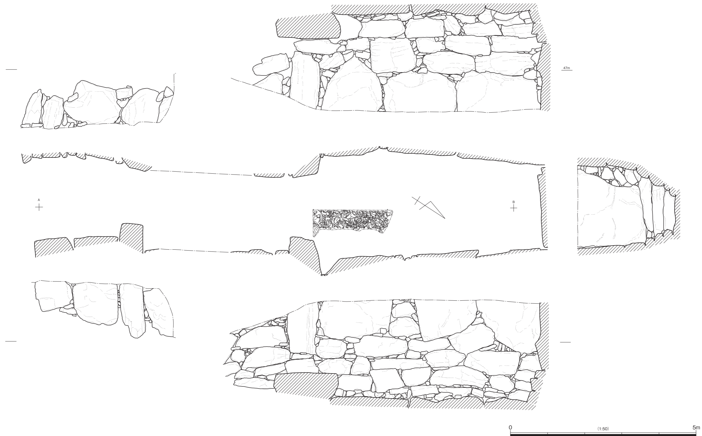
图 15 横穴式石室平面·壁面
