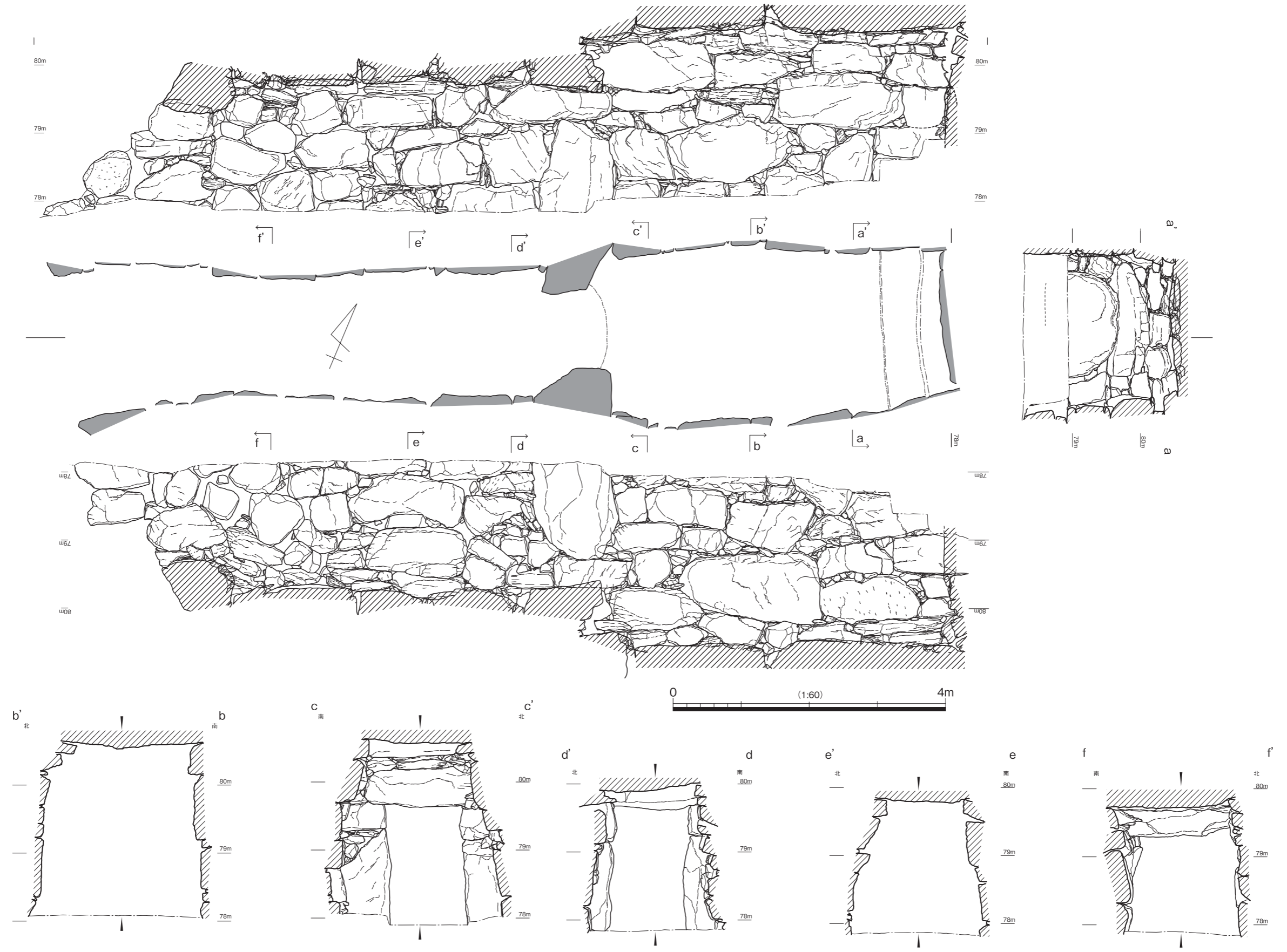
图19 穴薬師（綾織塚）古墳石室平面・壁面
