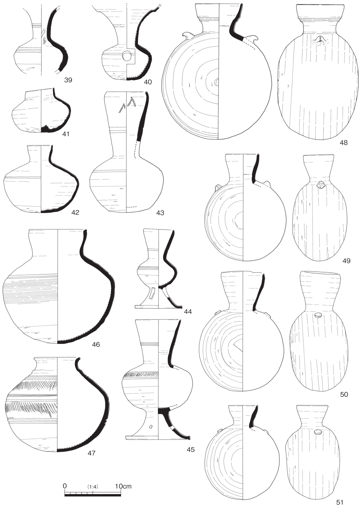
図 23 仏願 1 号墳出土遺物 2
