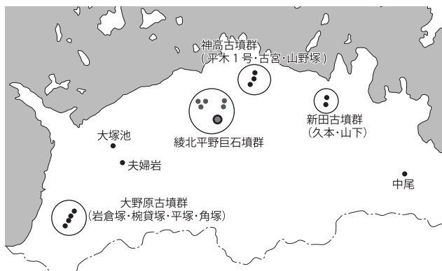
図1 讃岐地域の巨石墳の分布
