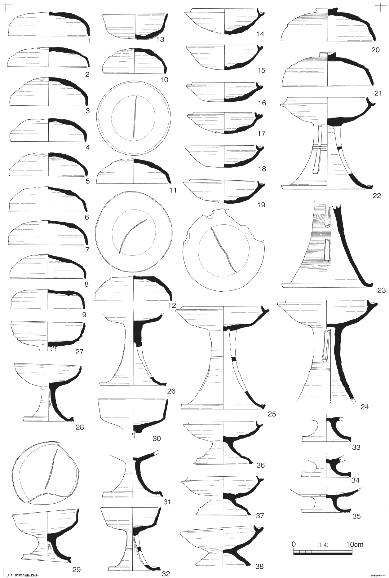
图 22 仏願 1 号墳出土遺物 1
