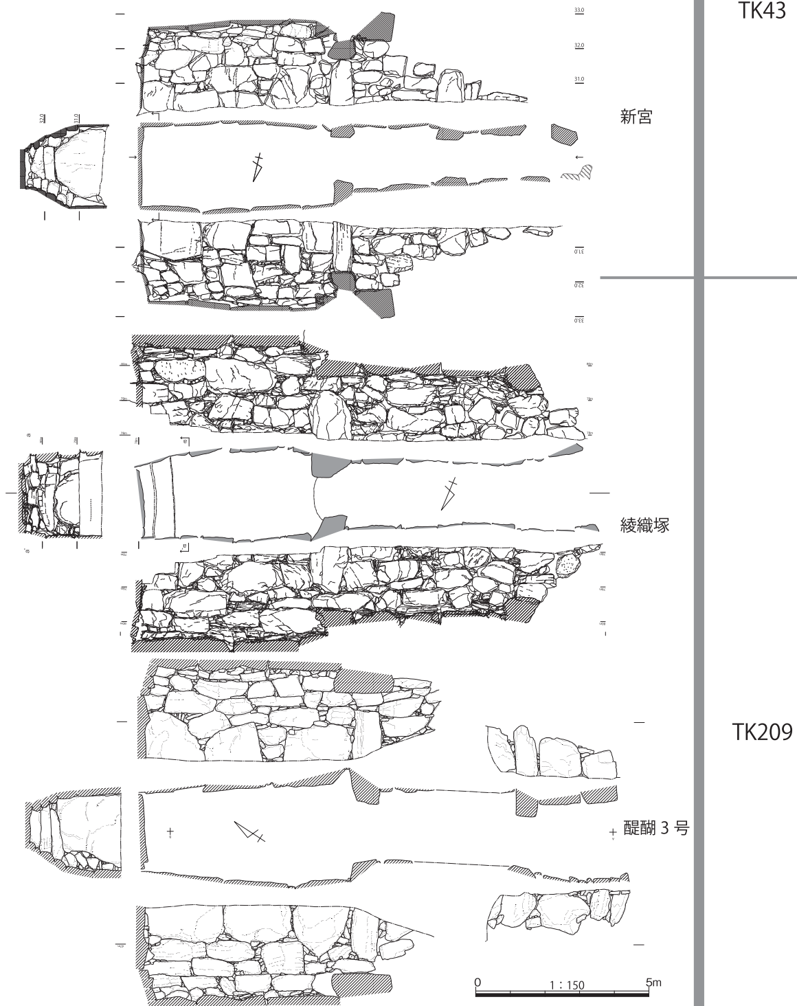
図 29 玄門立柱構造の大型横穴式石室の変遷（綾北古墳群）
