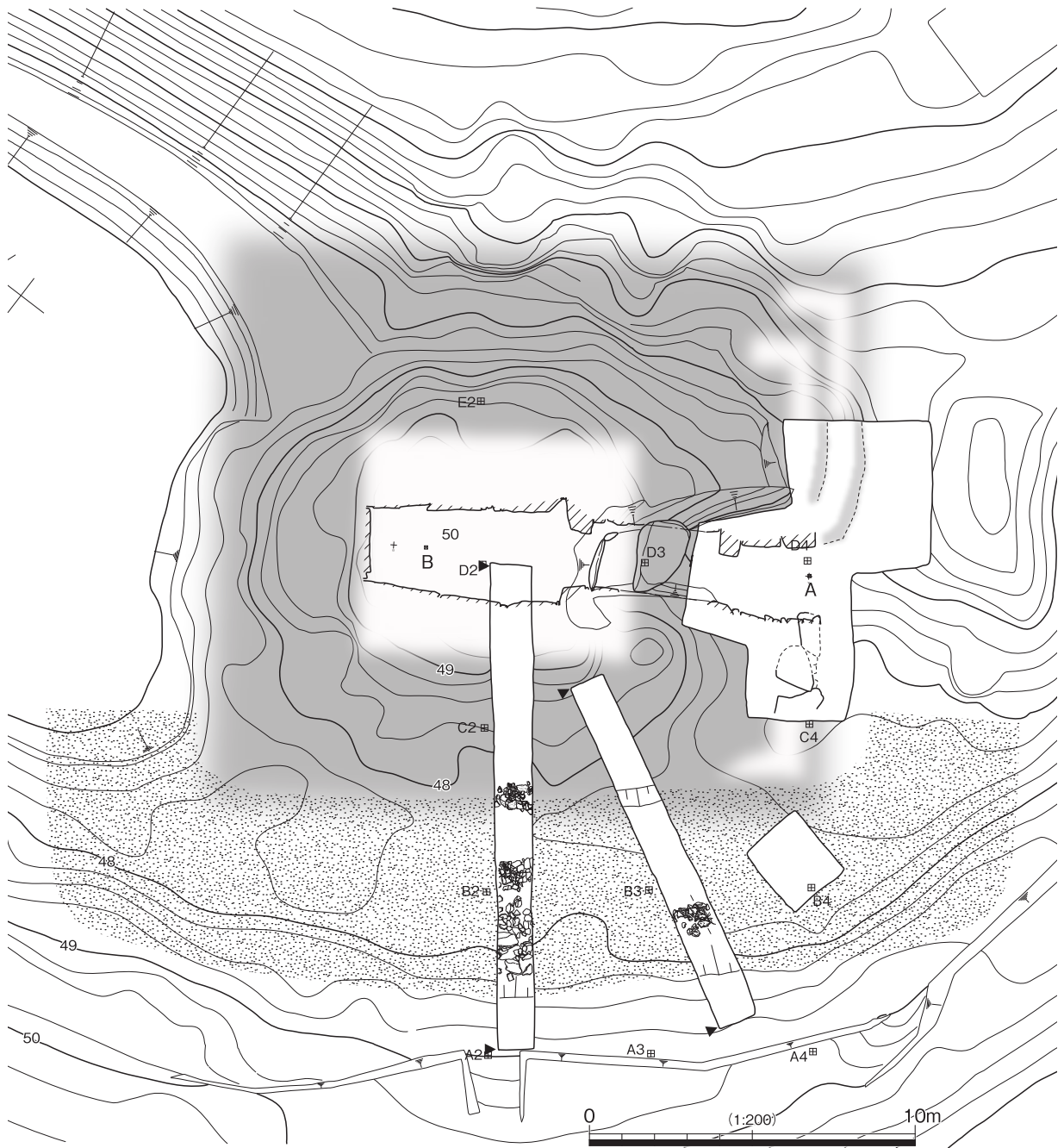
図 14 墳丘復元図
