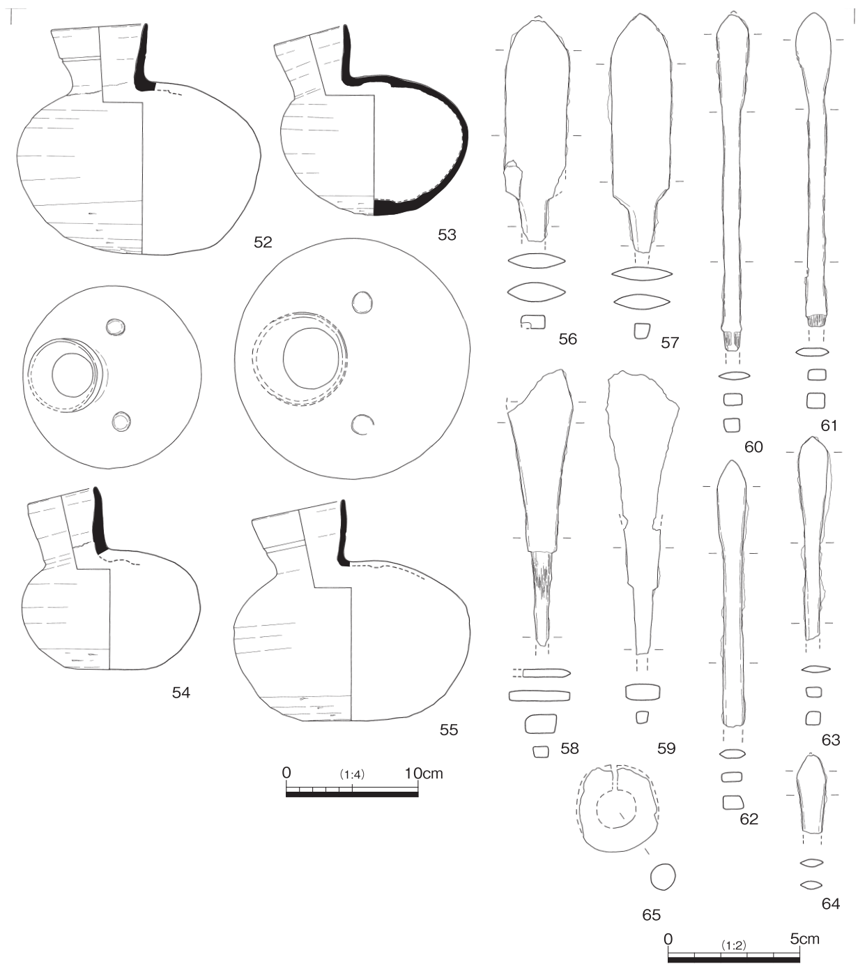
図 24 仏願 1 号墳出土遺物 3
