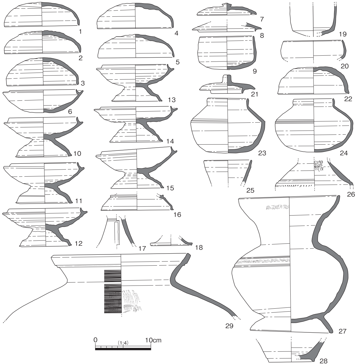
図7 前庭部出土須恵器
