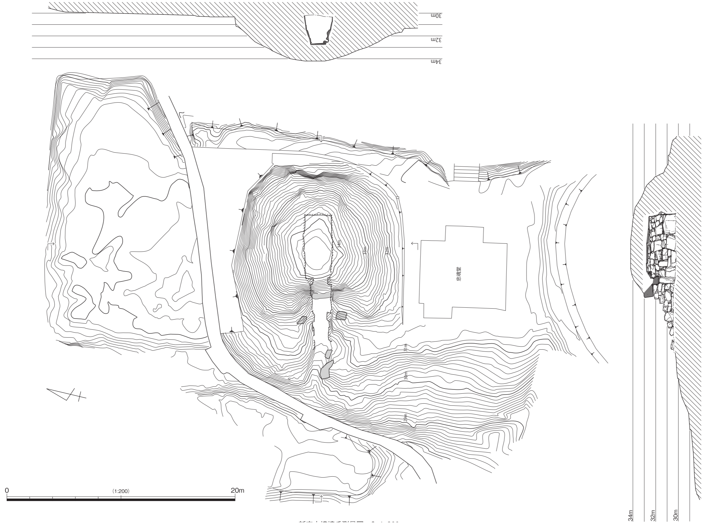
图3 墳丘測量図
