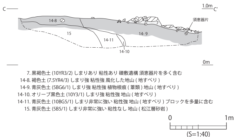
第52図 D区 トレンチ1・2土層図(1:40)
