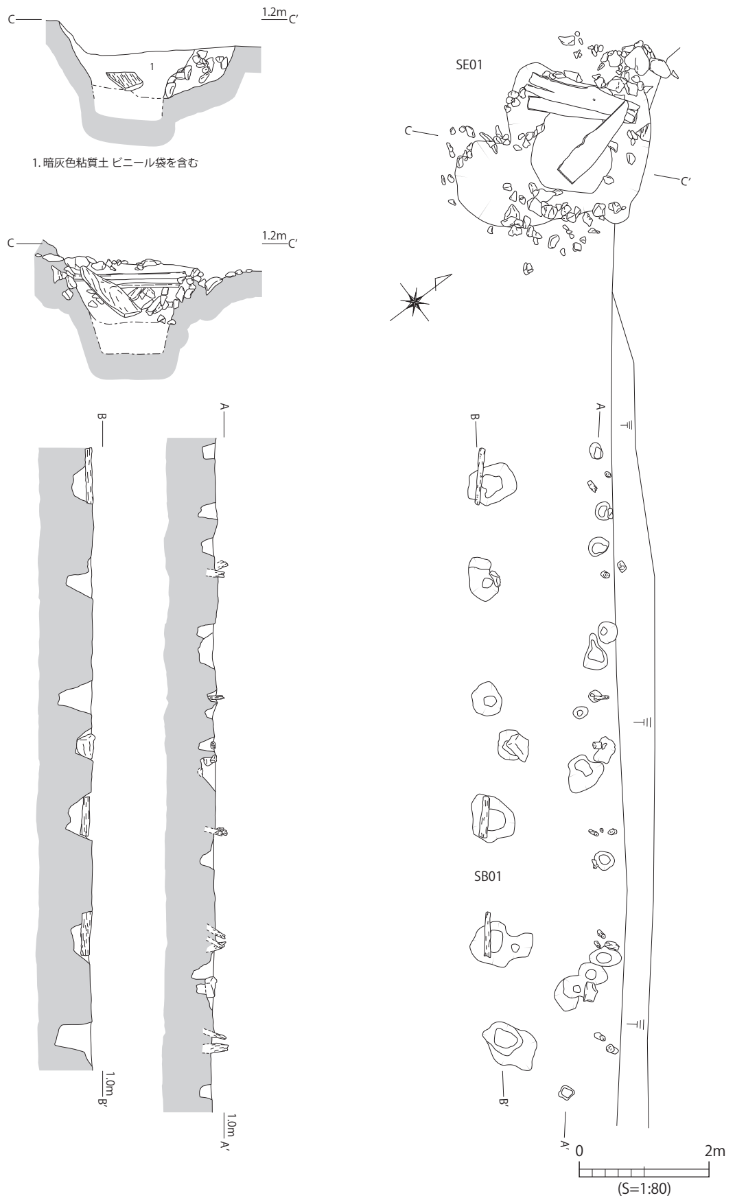
第13図 A-2区 SB01・SE01実測図(1:80)
