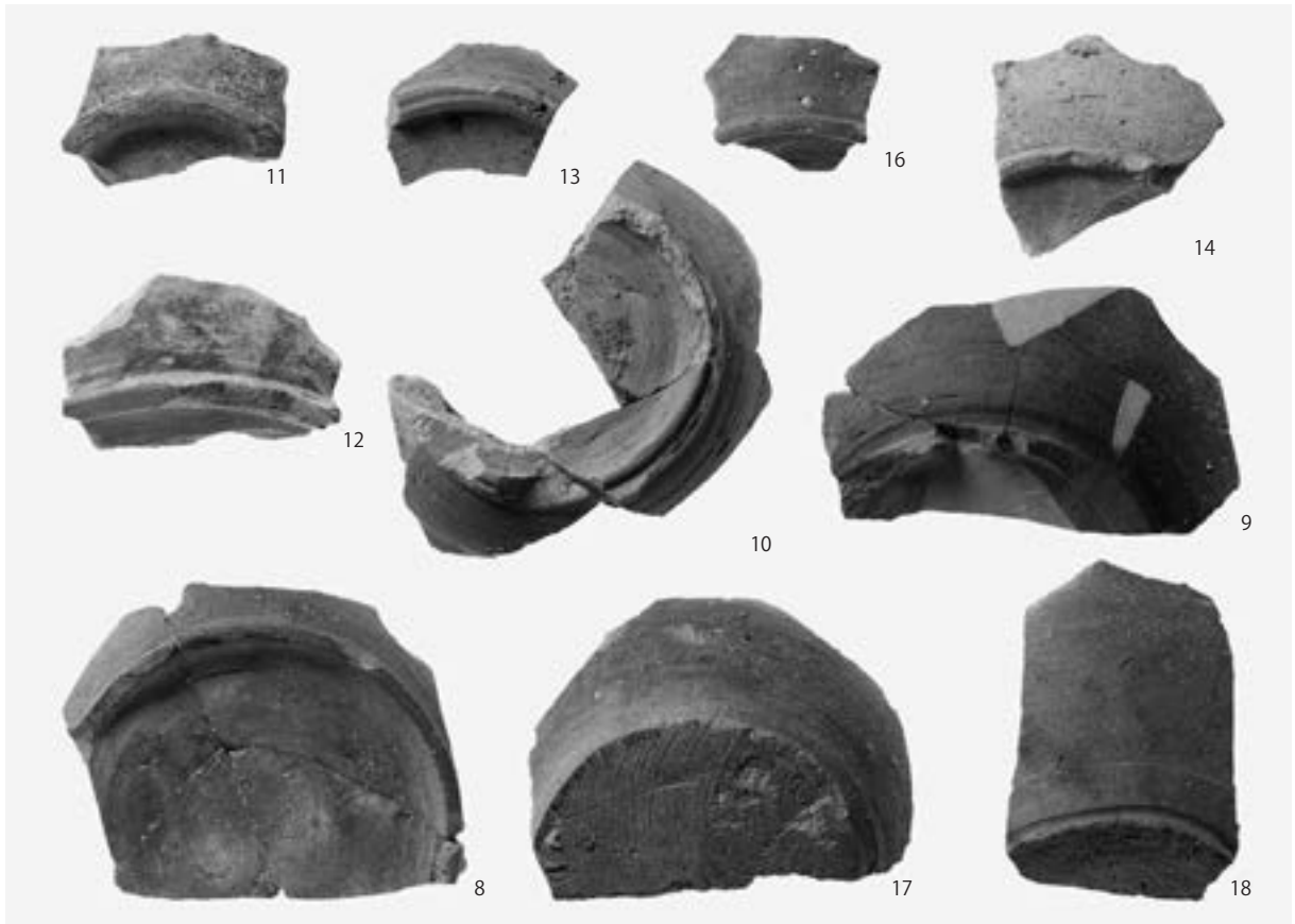
1. C区 礫敷遺構出土須恵器 (第34图)
