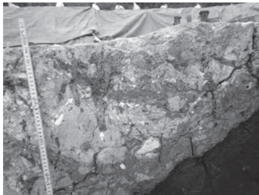
第91図 地すべり堆積物中に発達した生痕化石
