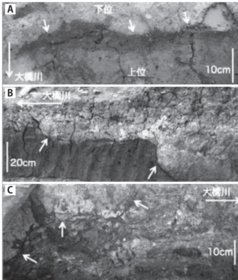
第89図 地すべり堆積物の様子
