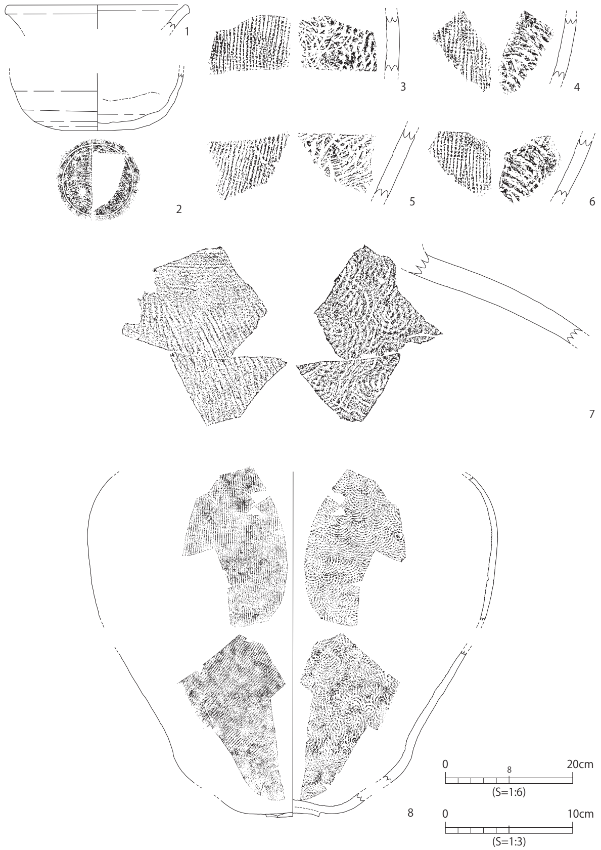
第19図 B区 1号墳出土土器実測図
