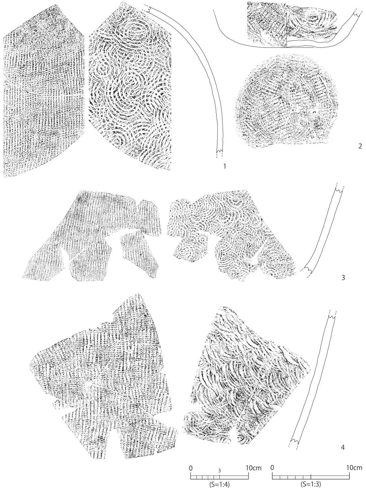
第36図 C区 礫敷遺構出土須恵器実測図5
