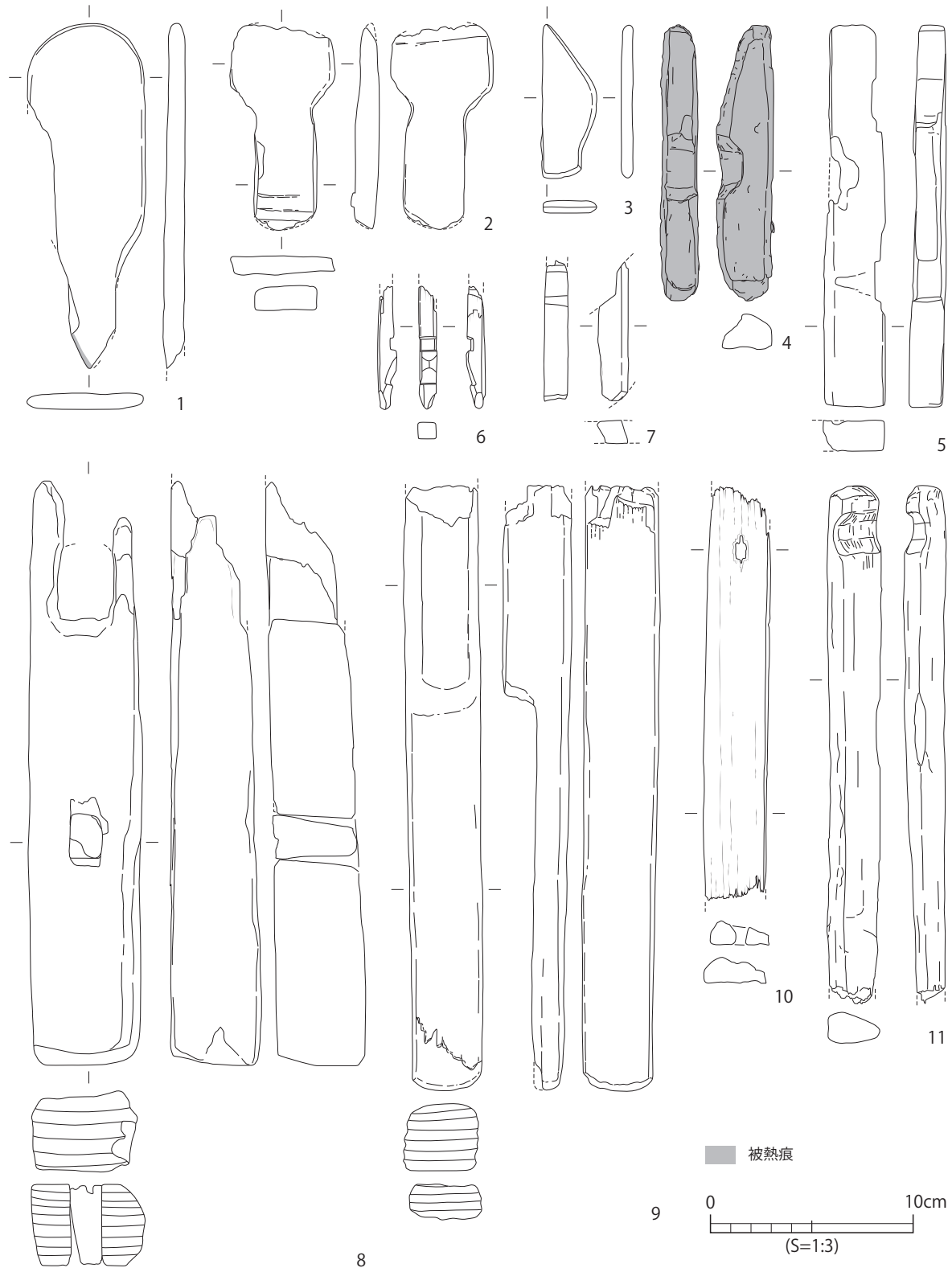
第68図 D区 包含層出土木製品実測図3
