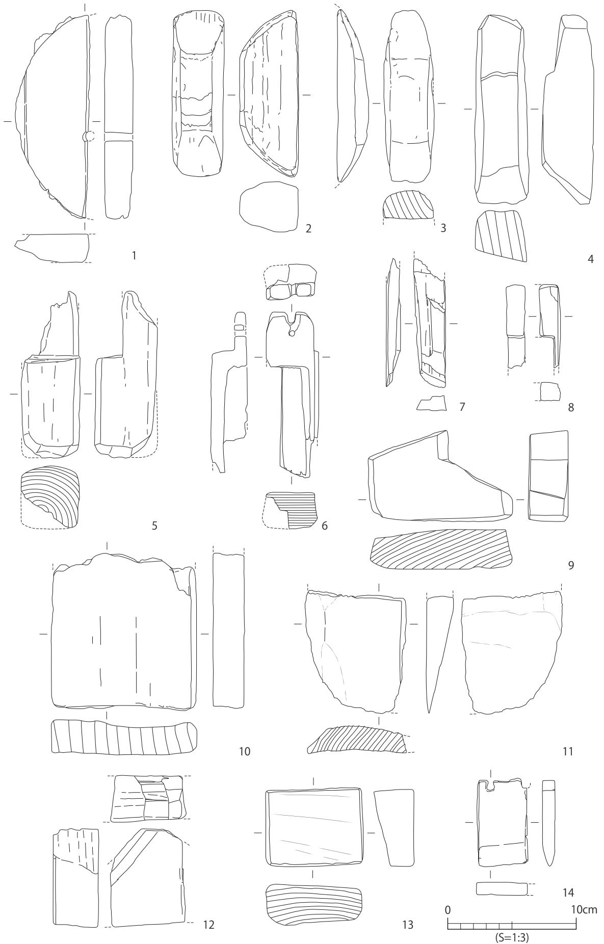
第67図 D区 包含層出土木製品実測図2
