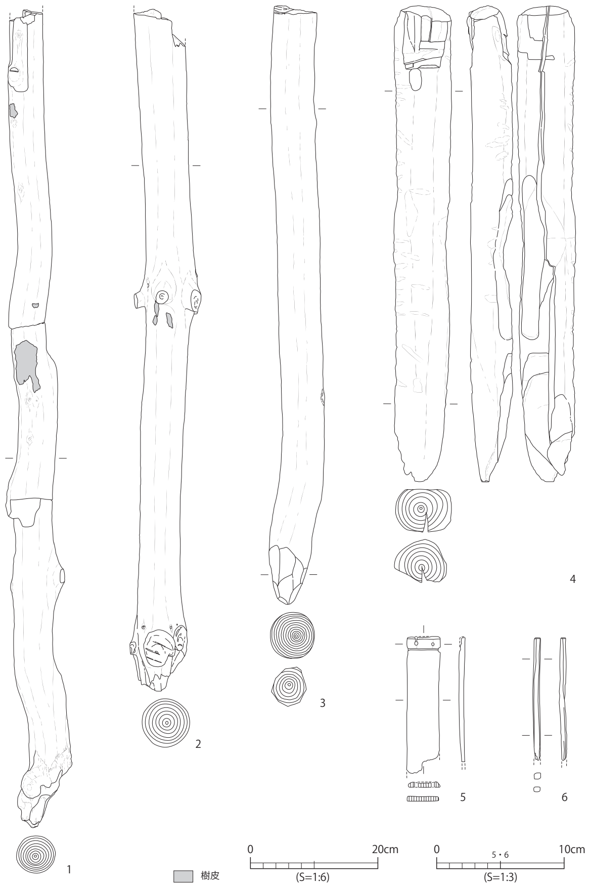
第39図 C区 礫敷遺構出土杭・木製品実測図
