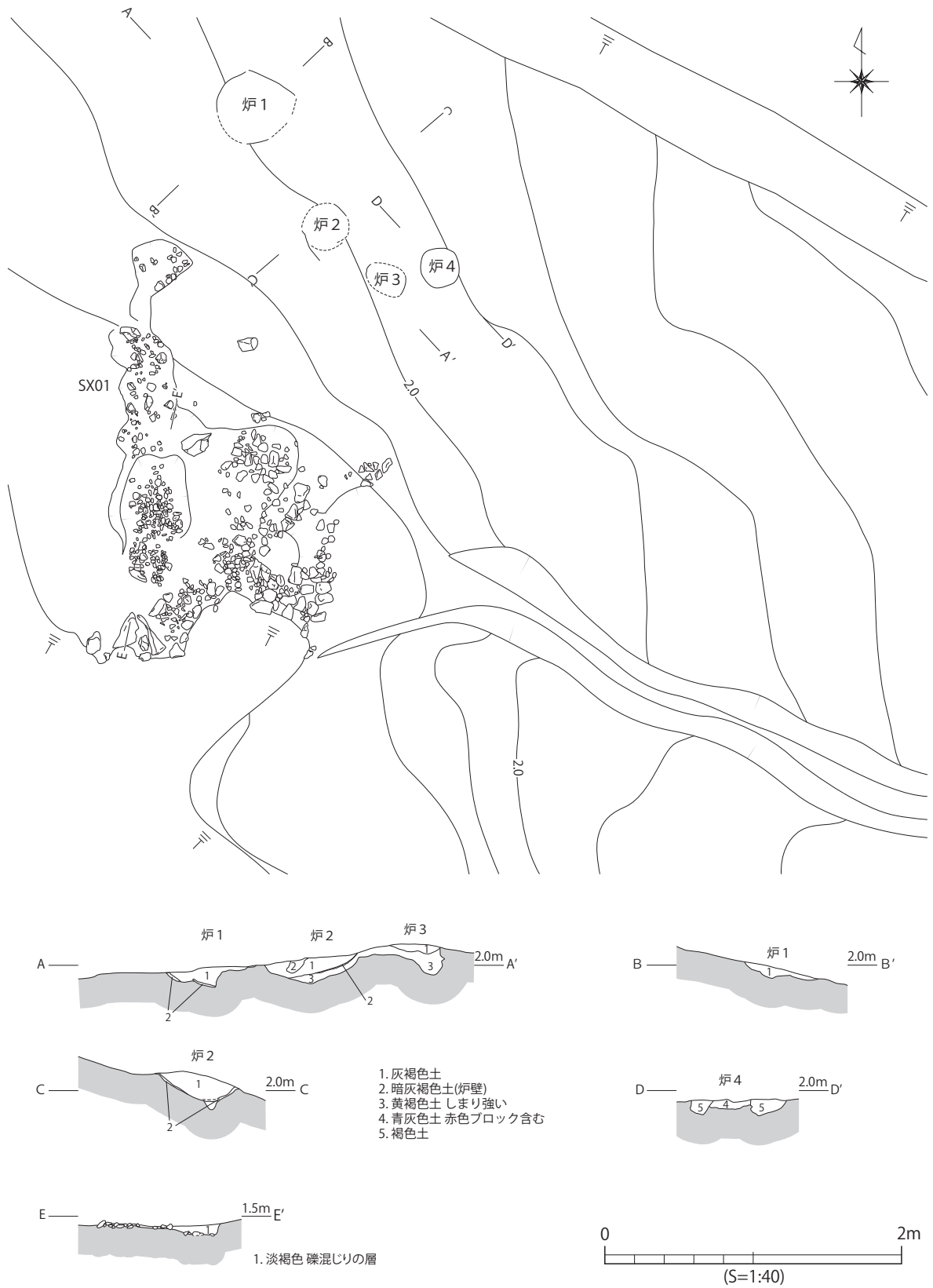
第24図 B区 炉跡実測図(1:40)
