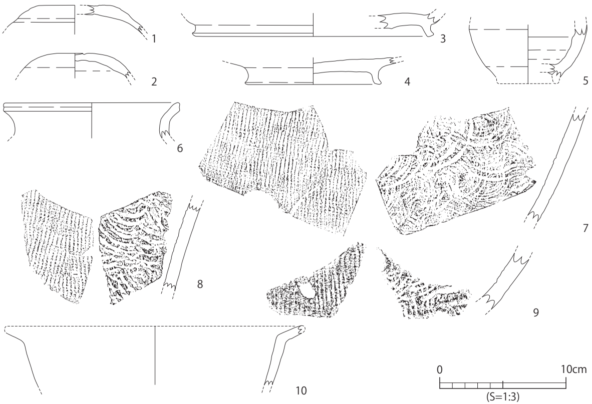
第23図 B区 2号墳出土土器実測図
