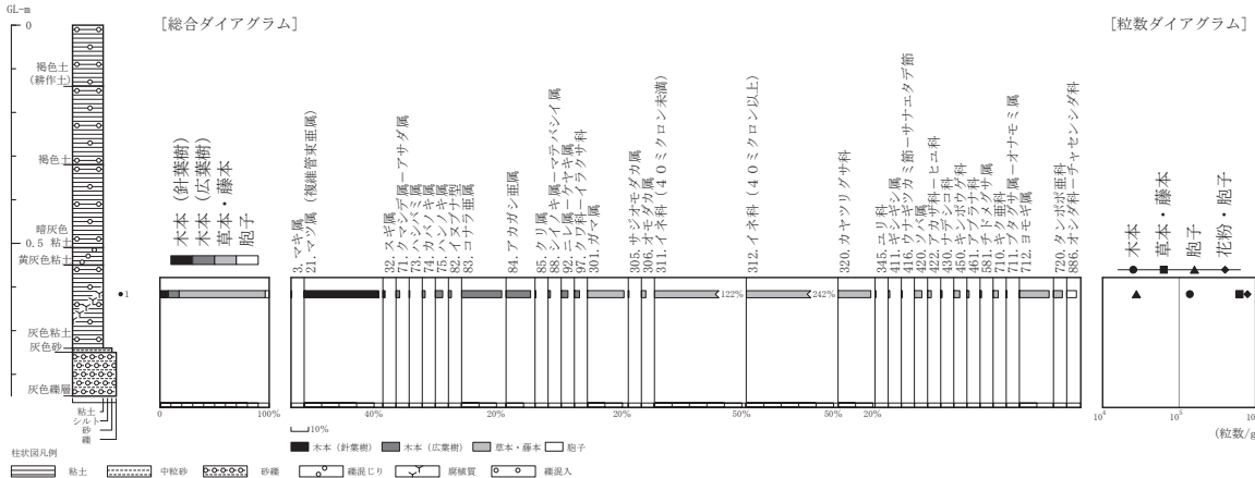
第80図 花粉ダイアグラム (A-2区)
