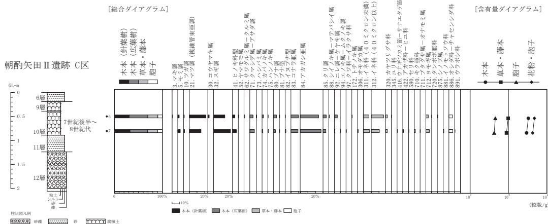
第83図 花粉ダイアグラム (C区)
