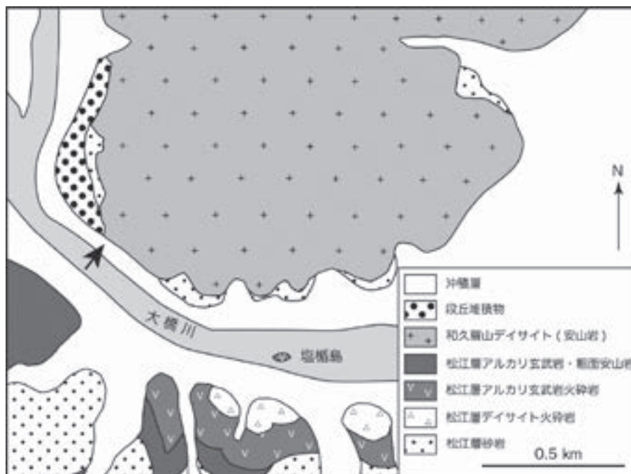
第87図 遺跡周辺の地質（鹿野ほか, 1994）
