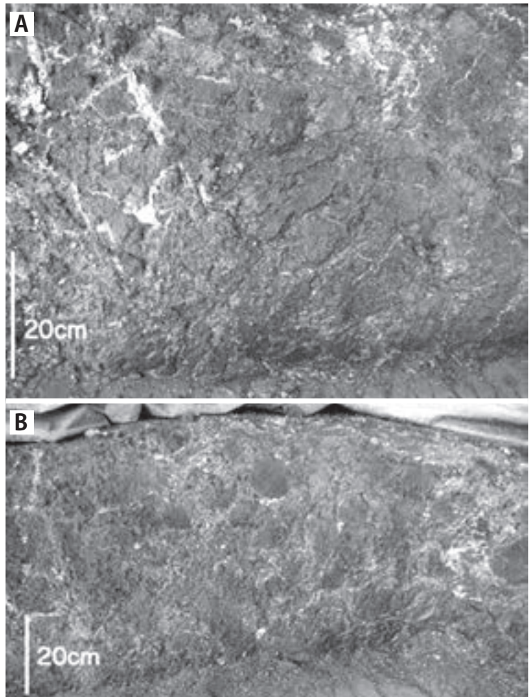
第88図 松江層の玄武岩
