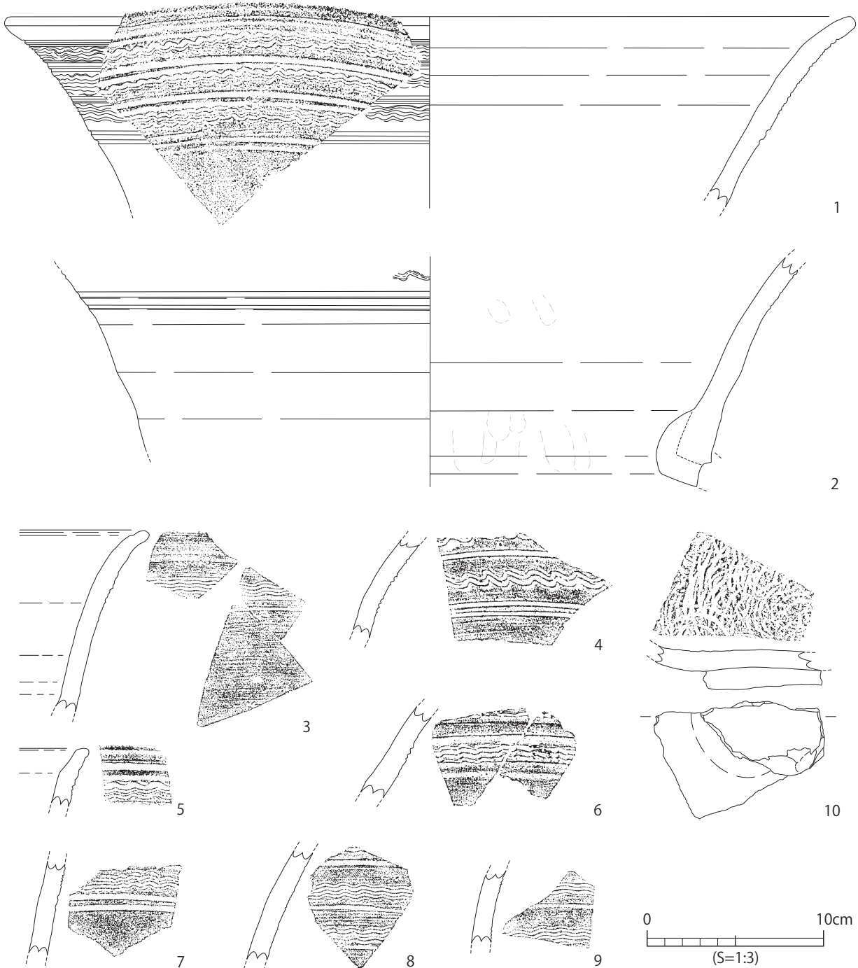
第35図 C区 礫敷遺構出土須恵器実測図4
