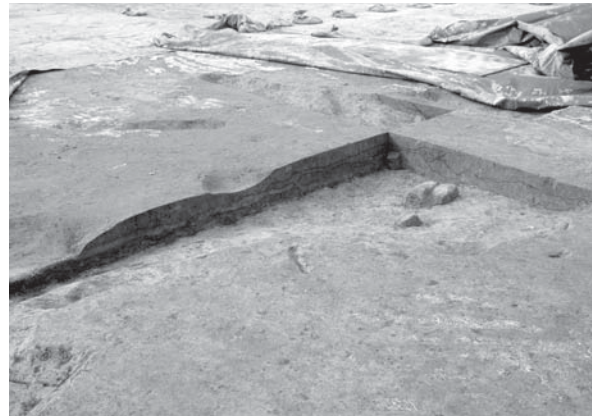
I18区 SDd044 溜まり部 N'-N(M'-Mを含む)土層断面 北から
