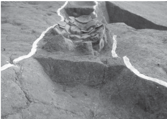
B18区 SDd100 D'-D 土層断面 北から
