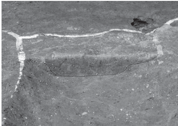
I21 区 SDd001 A-A' 土層断面 南から
