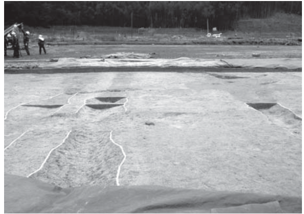
I18区 SDd041 L'-L・042 K'-K・044 J'-J 土層断面 西から
