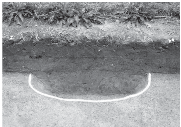
D19区 SKd37 土層断面 西から
