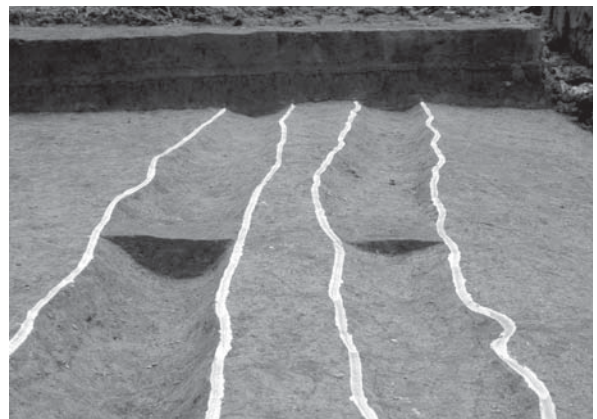
D20区 SDd055(左)・054(右) B'-B 土層断面 北から
