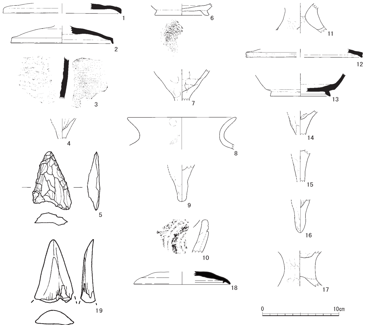
第6図 出土遺物実測図 (5・19:S=1/1、他:S=1/3)
