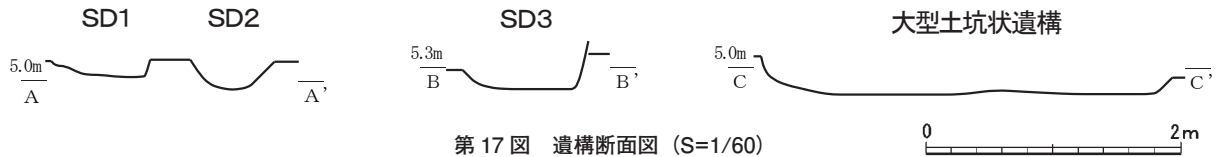
第17図 遺構断面図 (S=1/60)
