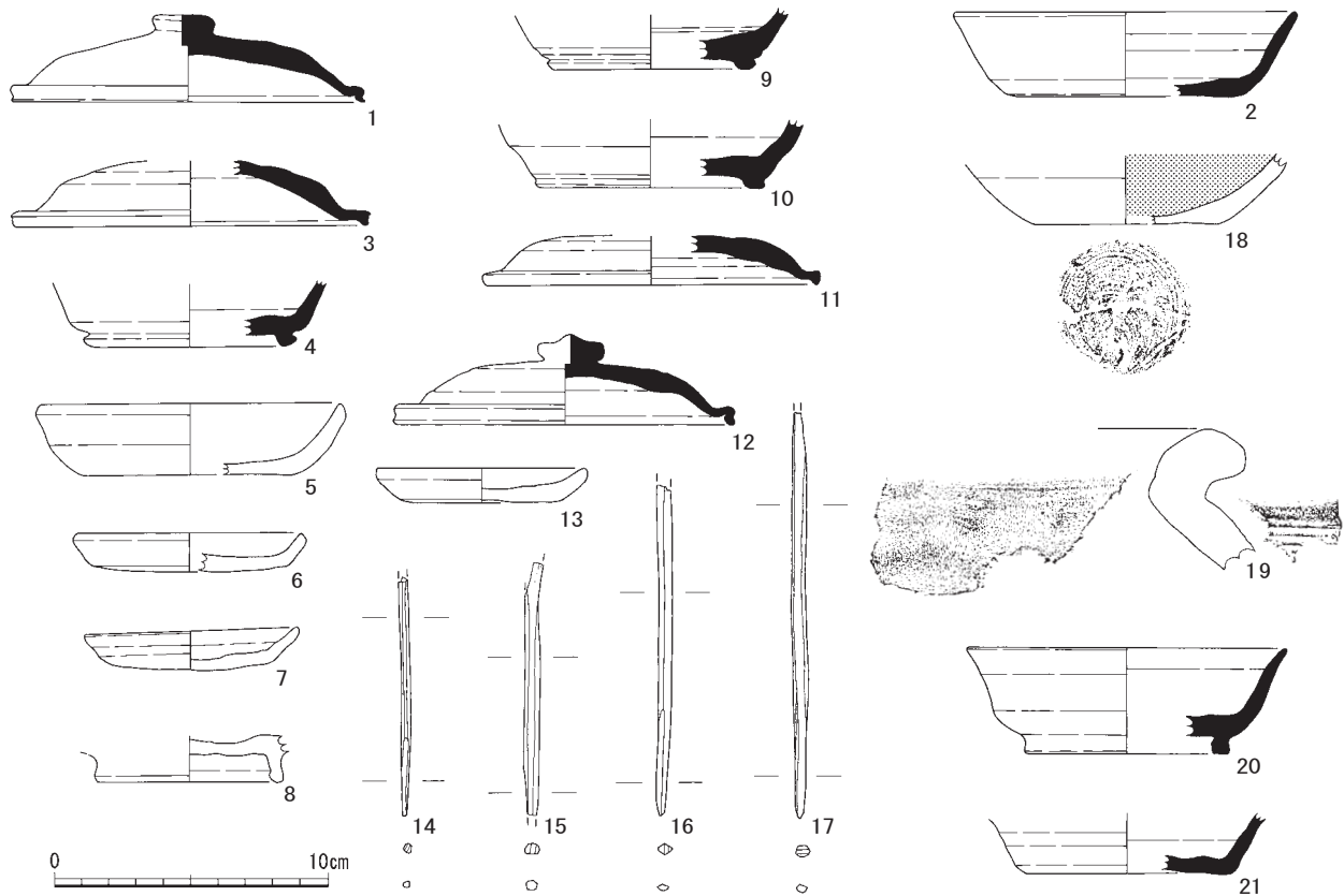
第18図 出土遺物実測図1 (S=1/3)
