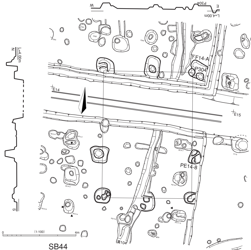
第37図 建物遺構図30
