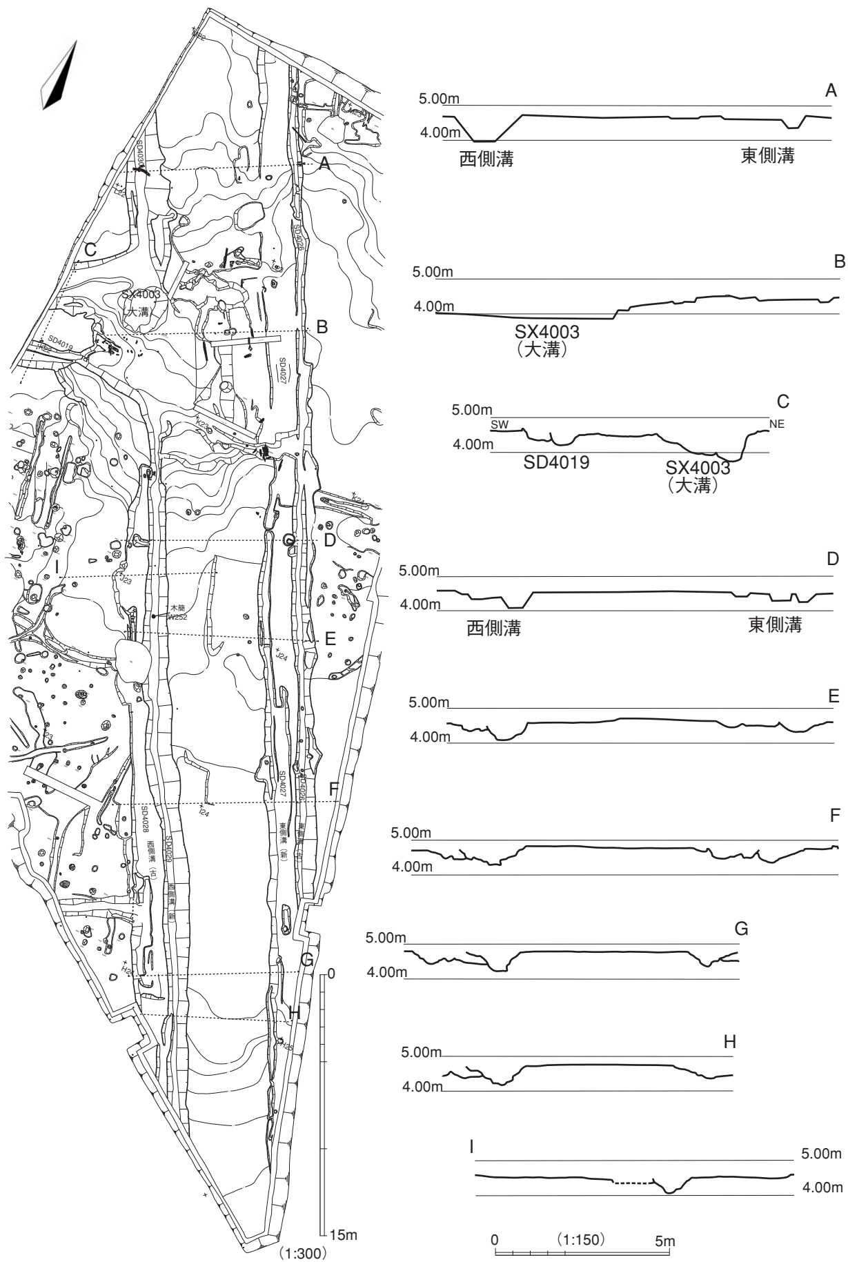
第79図 道路遺構図1
