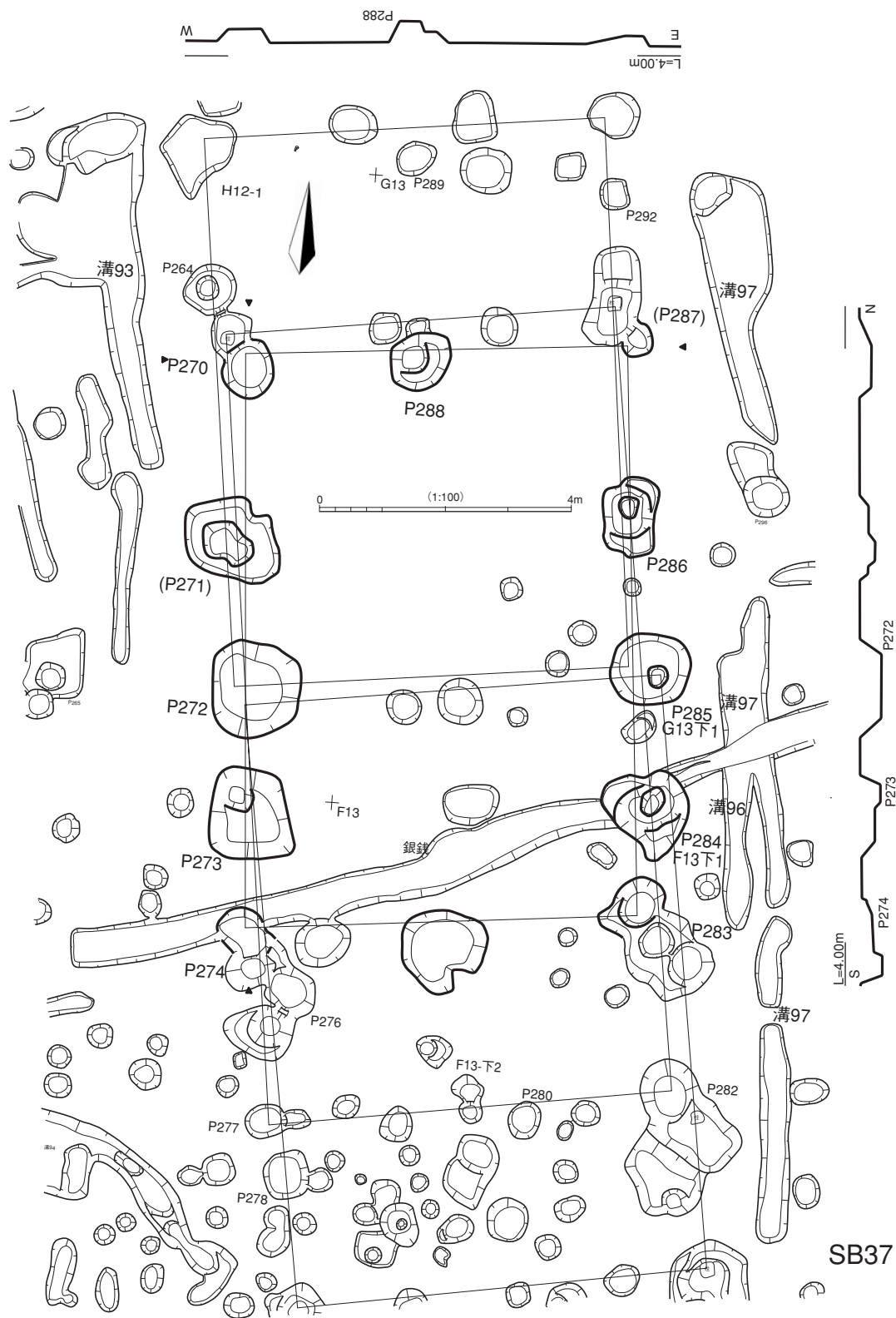
第32図 建物遺構図25
