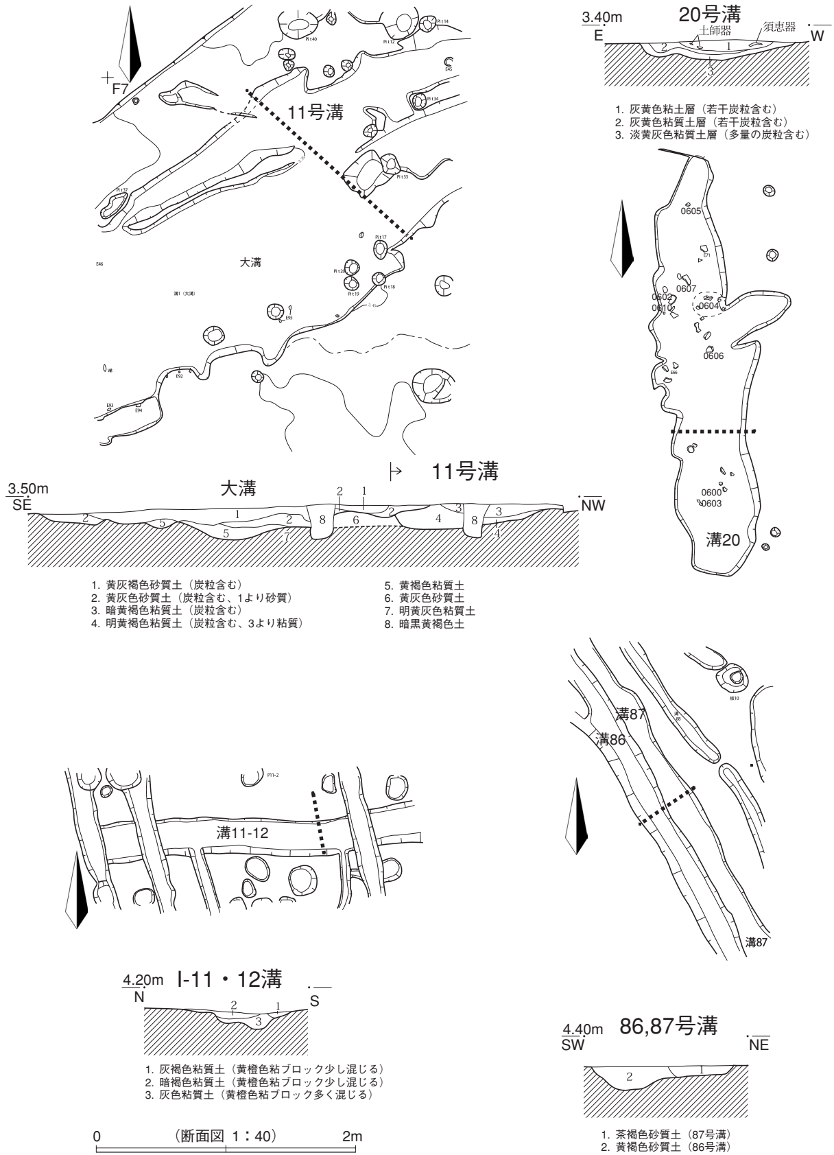
第75図 溝など遺構図1
