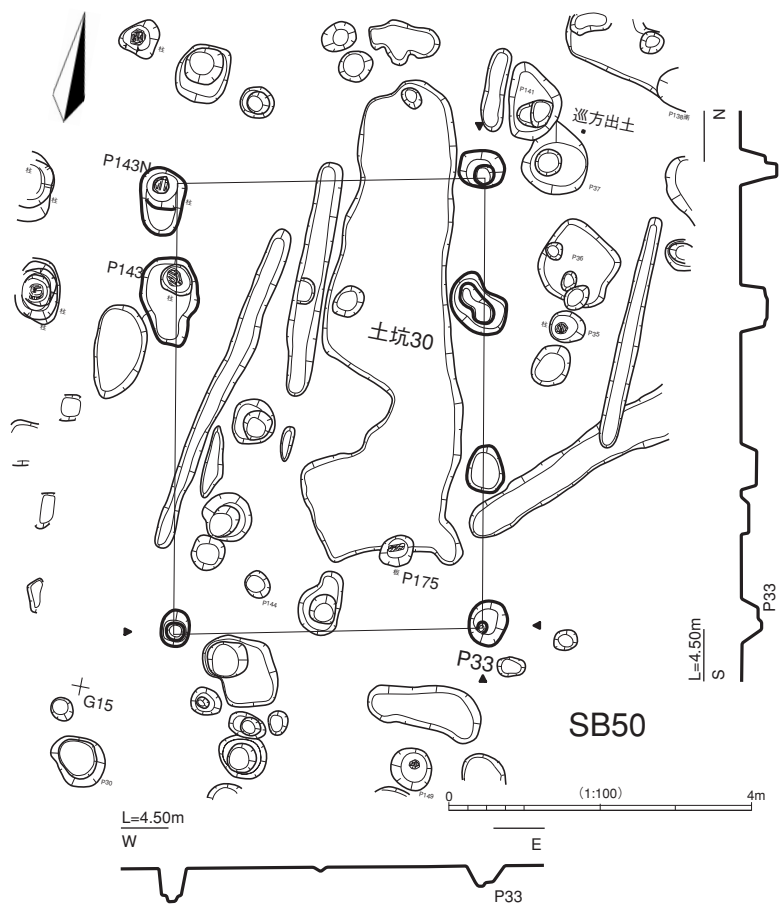
第42図 建物遺構図35
