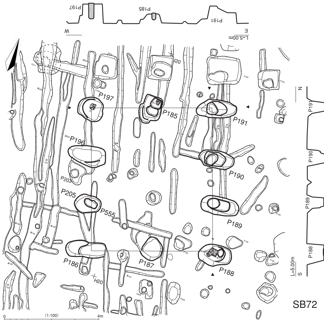
第55図 建物遺構図48
