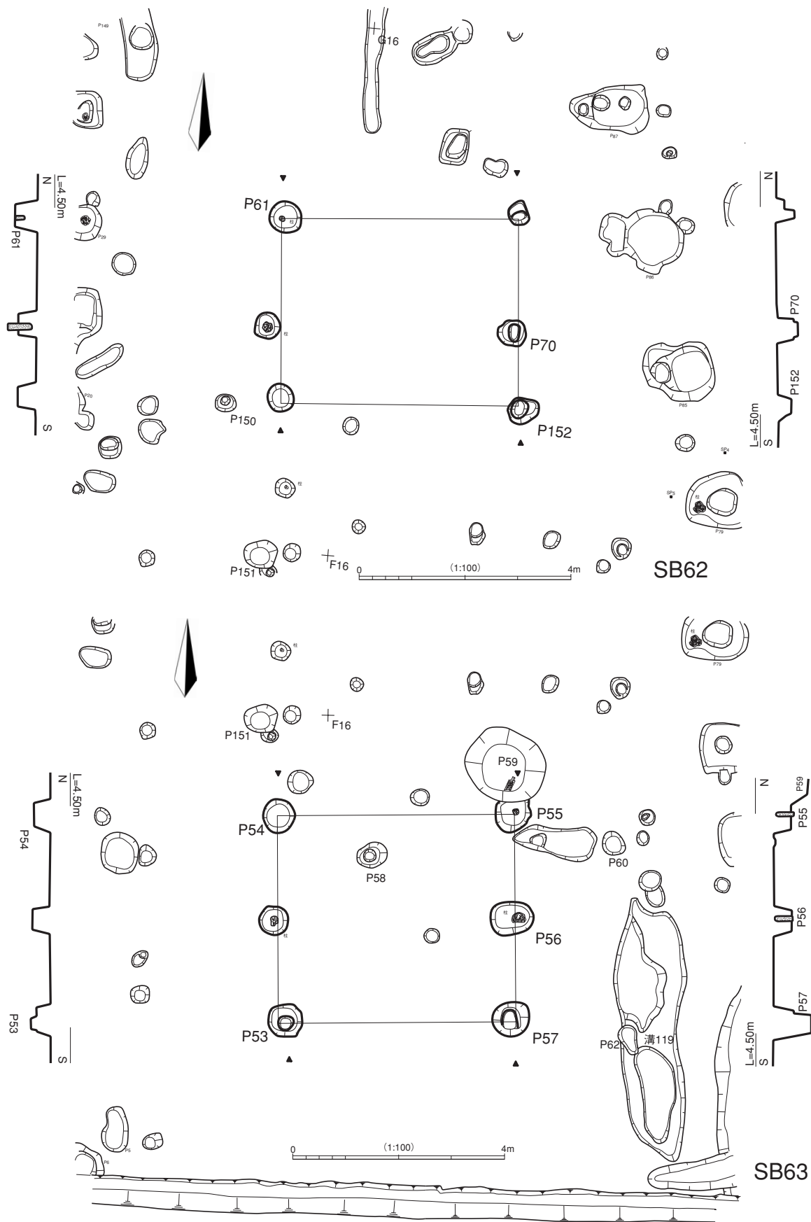
第48図 建物遺構図41
