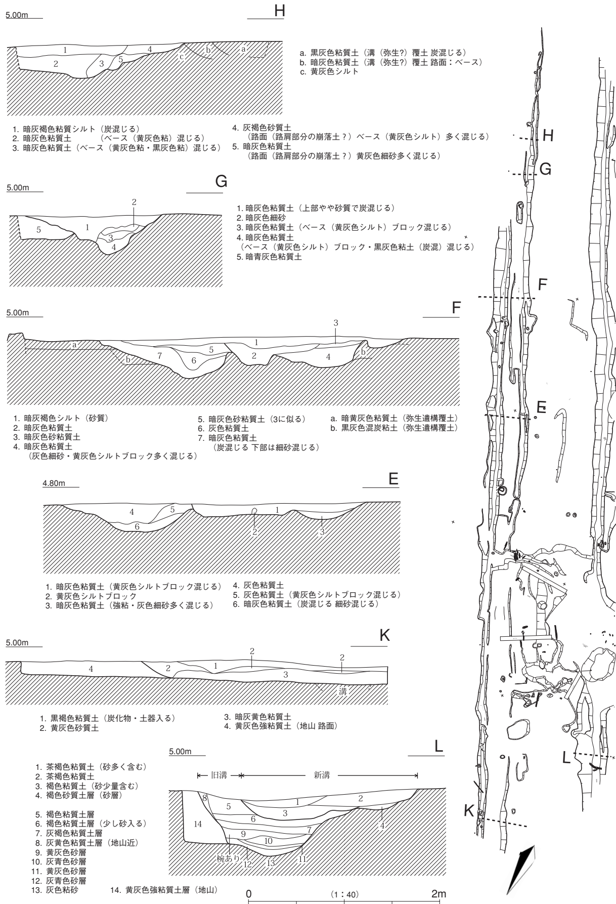
第81図 道路遺構図3
