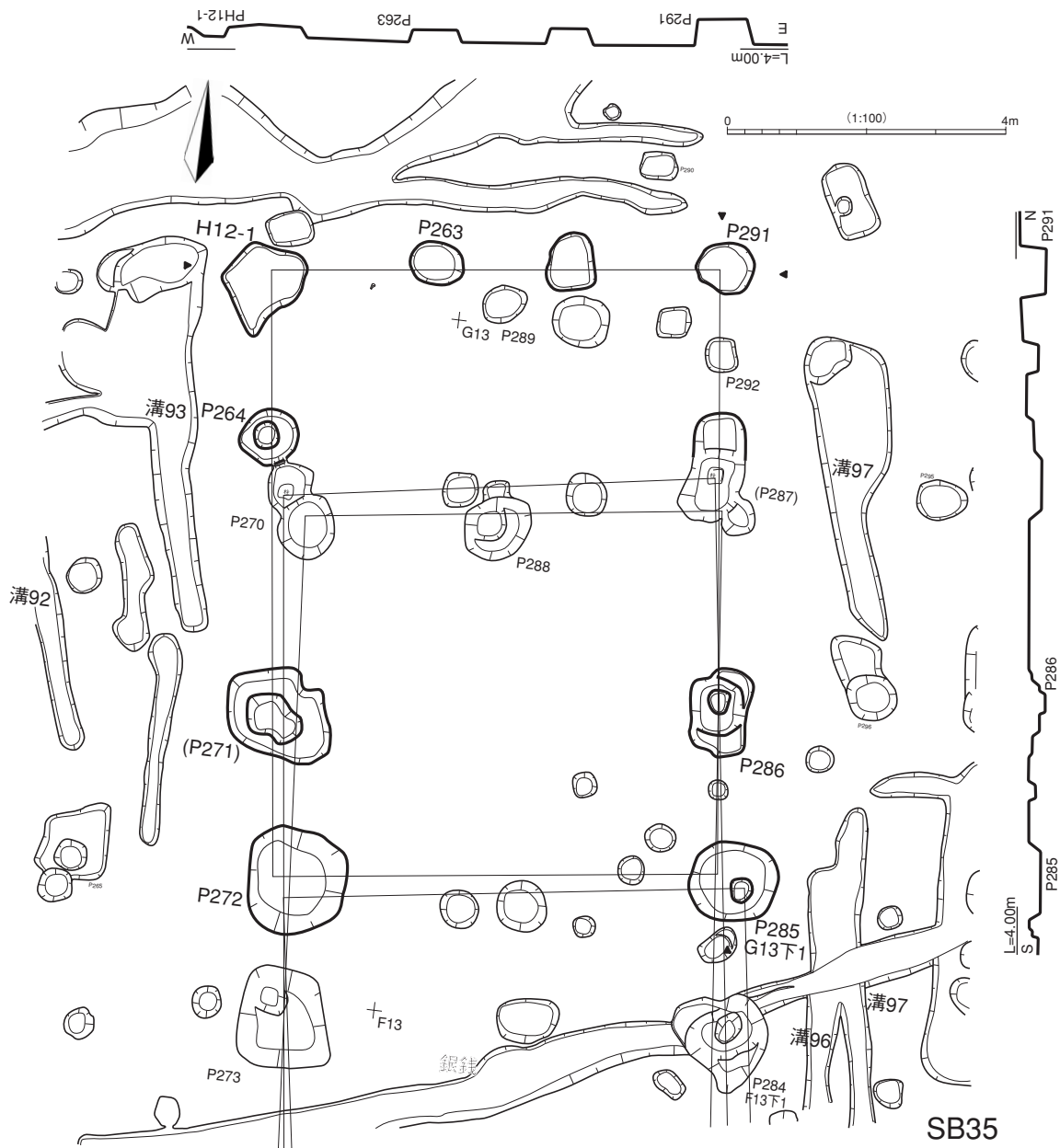
第30図 建物遺構図23
