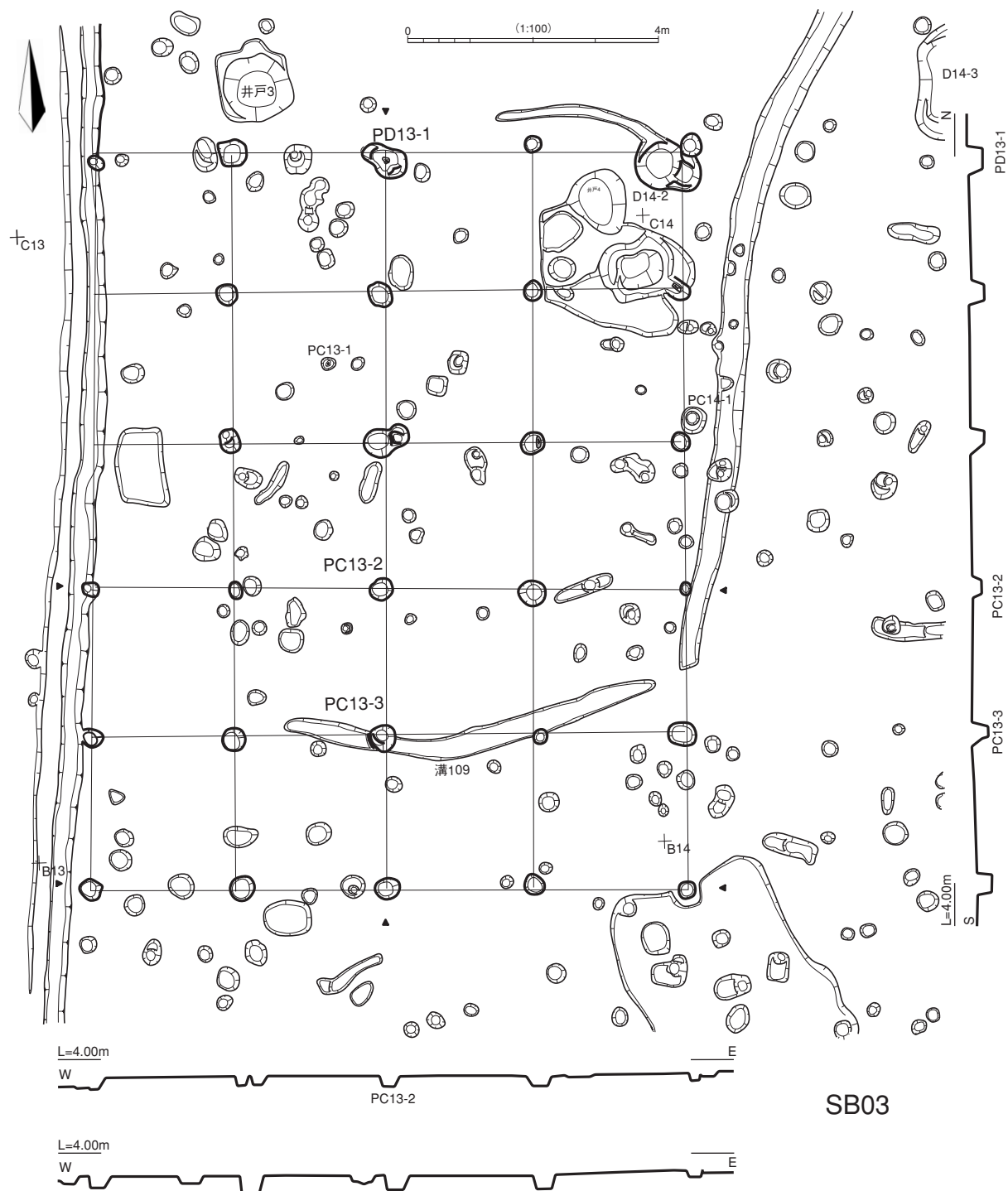
第10図 建物遺構図3
