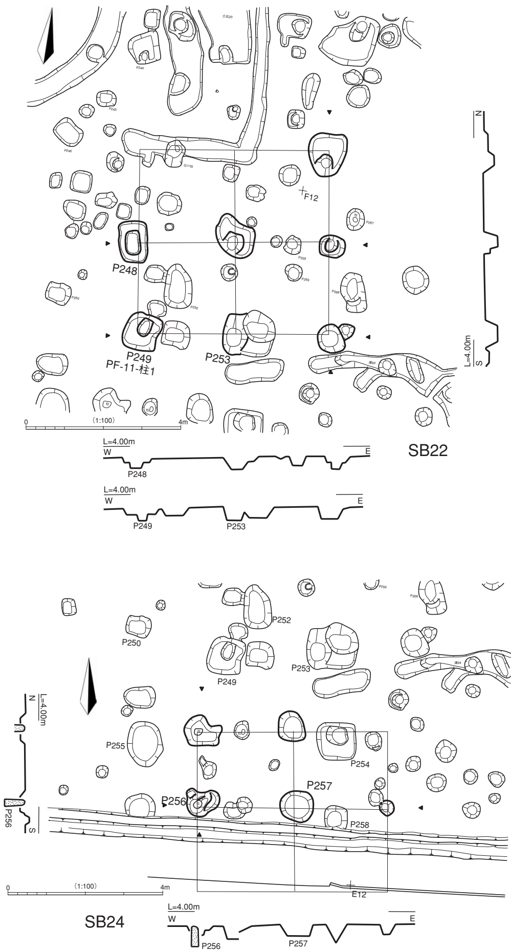
第22図 建物遺構図15
