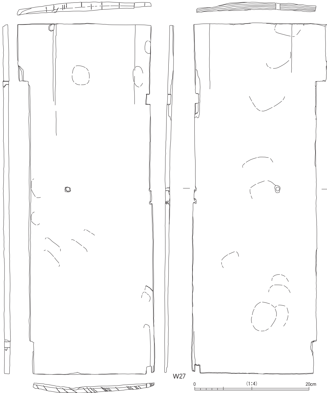
第297図 2000年度出土木製品実測図3 (加賀郡勝示札)
