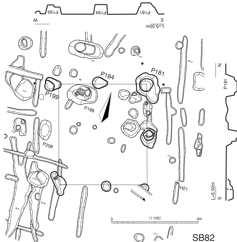
第62図 建物遺構図55
