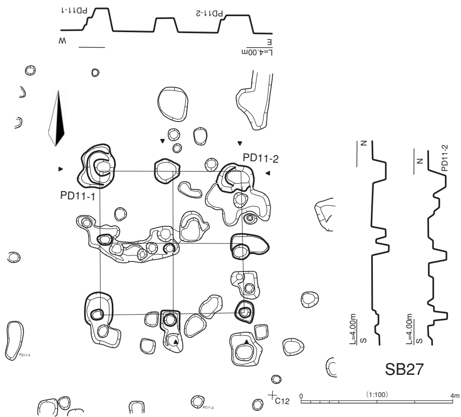
第24図 建物遺構図17
