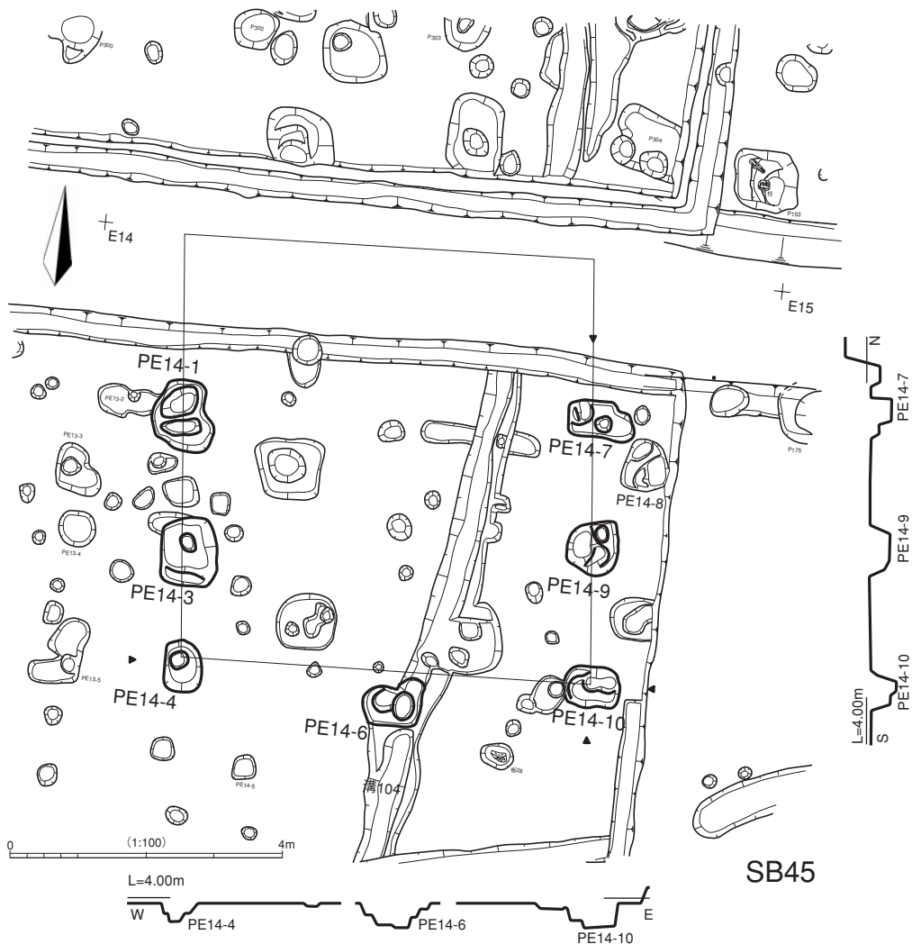
第38図 建物遺構図31
