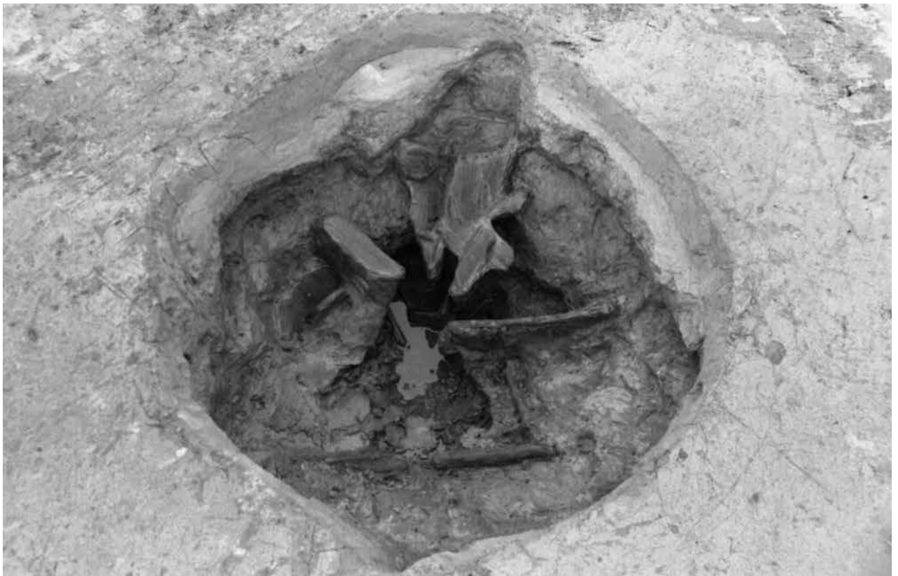
33号土坑（井戸） 木製品など検出状況
