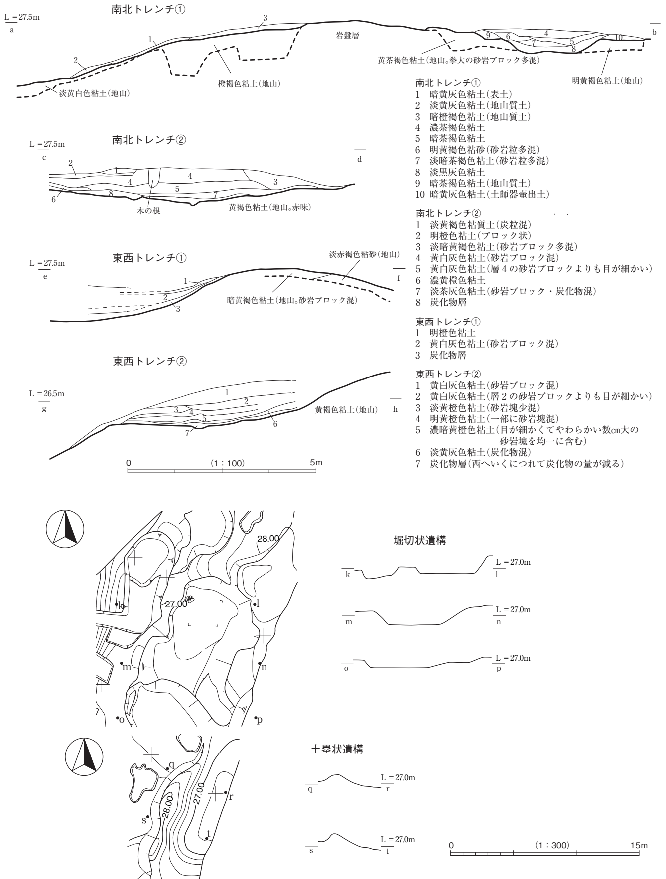
第6図 遺構実測図3 (S = 1/100・300)
