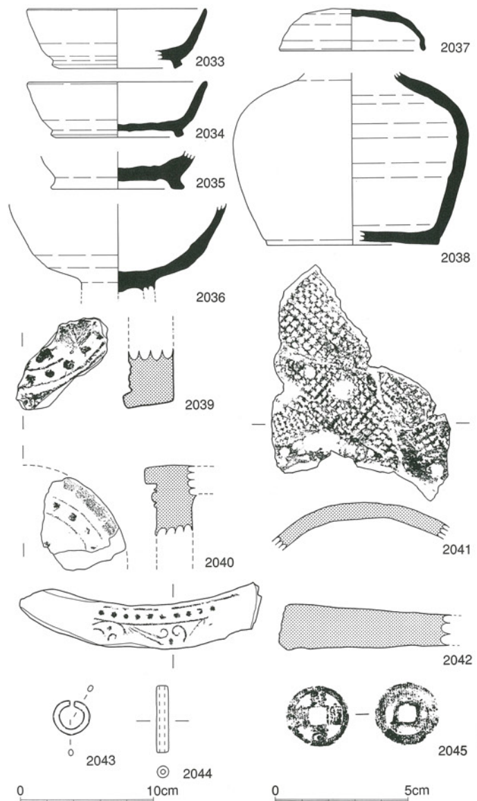
第221図 第6～10調査区遺構外出土遺物実測図(2)
