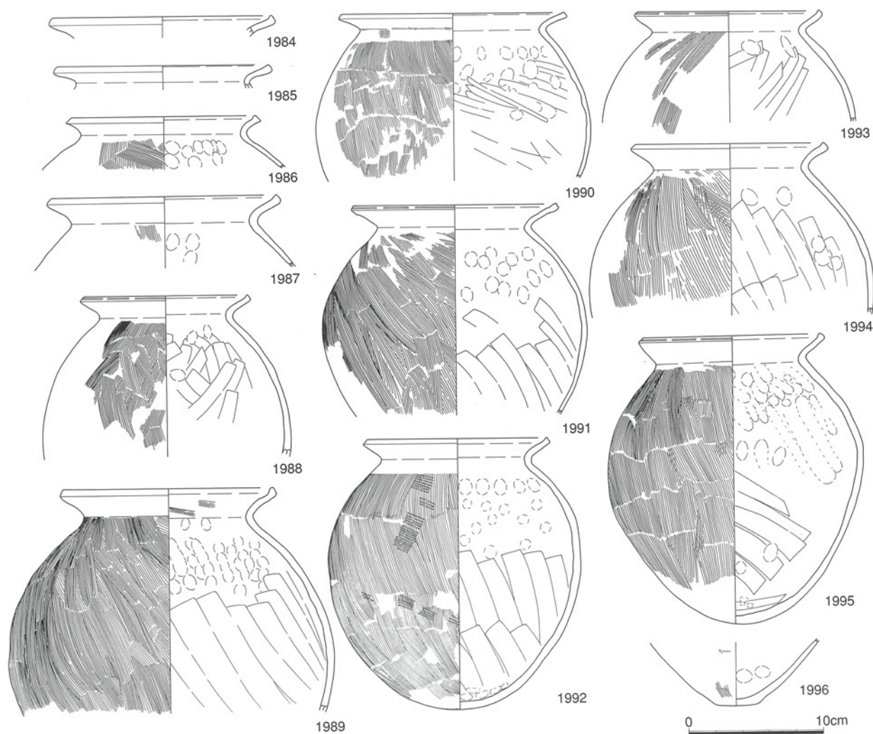
第210図 SK2046出土遺物実測図(2)
