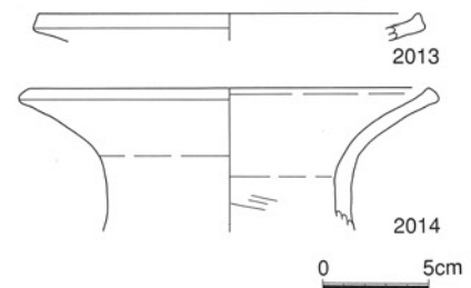
第214図 SX1008出土遺物実測図
