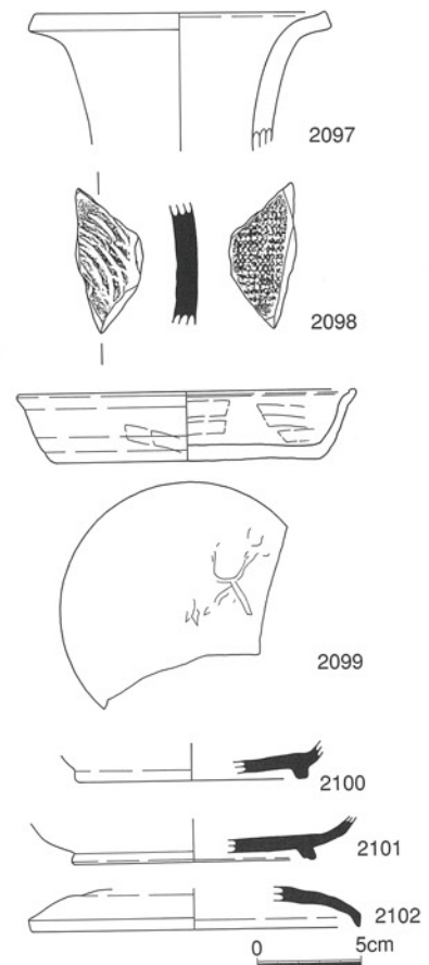
第235図 SK1093出土遺物実測図
