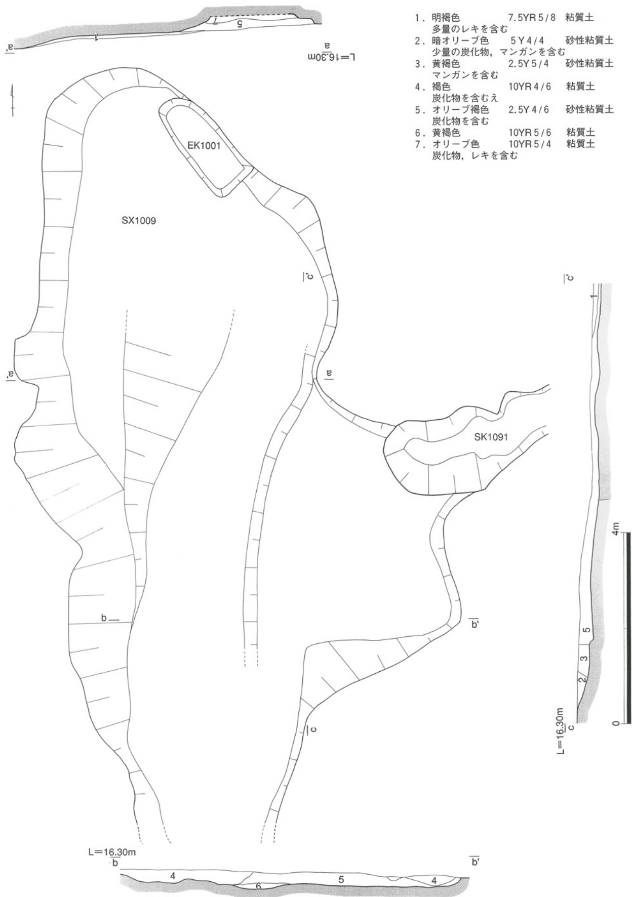
第238図 SX1009実測図
