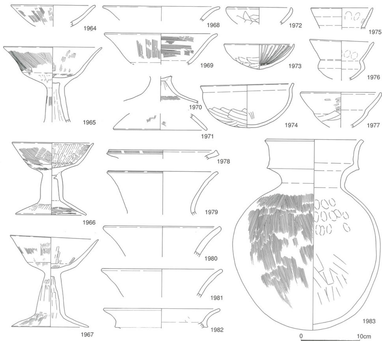
第209図 SK2046出土遺物実測図(1)
