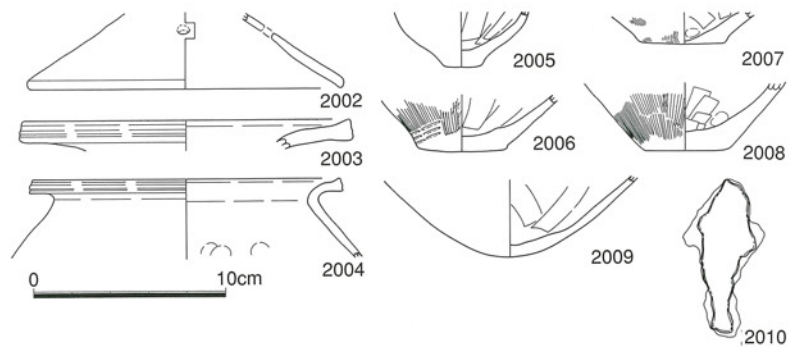
第212図 SX1005出土遺物実測図
