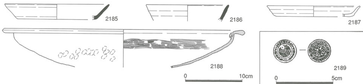
第241図 SK1092, SK1095, SX1010出土遺物実測図
