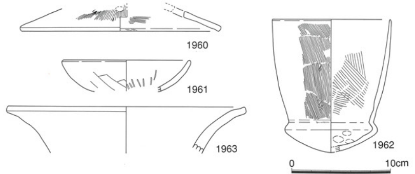
第207図 SK2045出土遺物実測図
