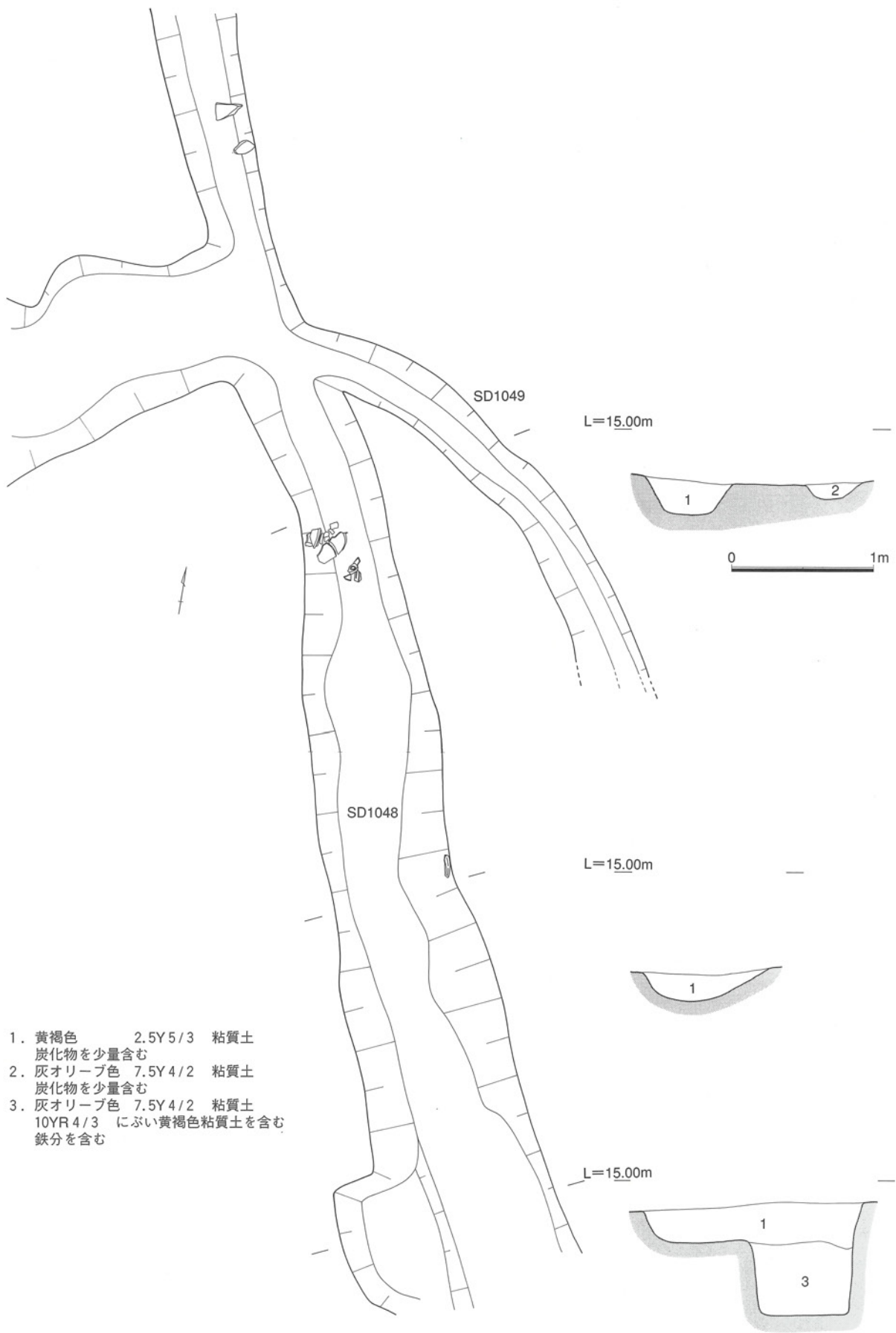
第230図 SD1048, SD1049実測図
