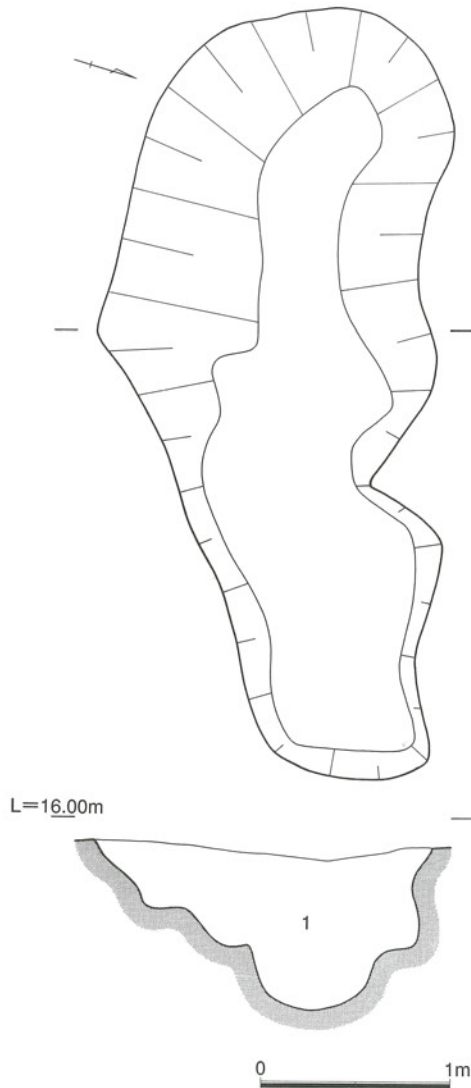
第232図 SK1091実測図
