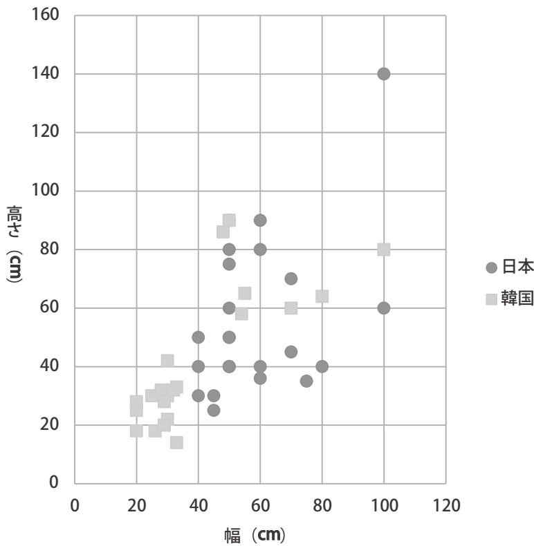
第8図 排水口の規模
