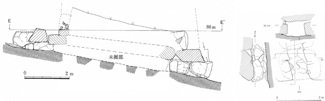
大廻小廻山城跡 一の木戸石壘 通水溝断面図と排水口 (1/100) (岡山市教育委員会 1989 より一部改変・転載)
