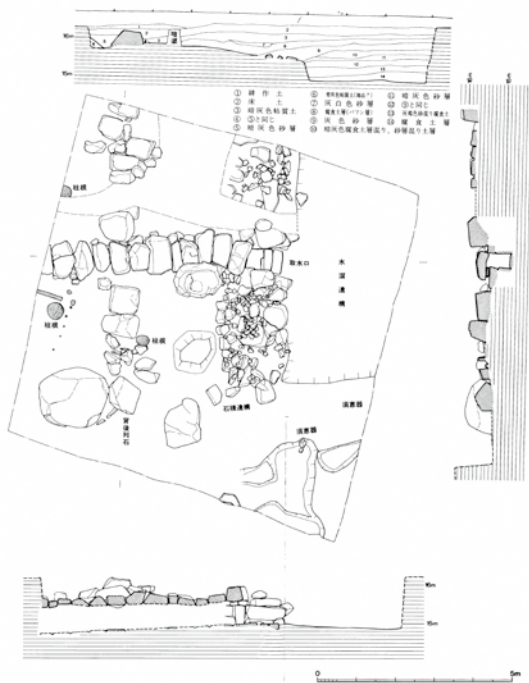
第14図 鹿毛馬神籠石 第1暗渠実測図(1/200) (颯田町教育委員会 1984より転載)
