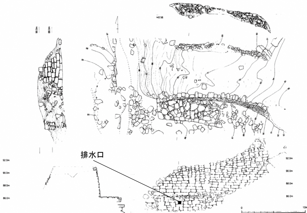
第11図 御所ヶ谷神籠石 中門石塁平面・立面・断面図 (1/400) (行橋市教育委員会 2006 より一部改変・転載)
