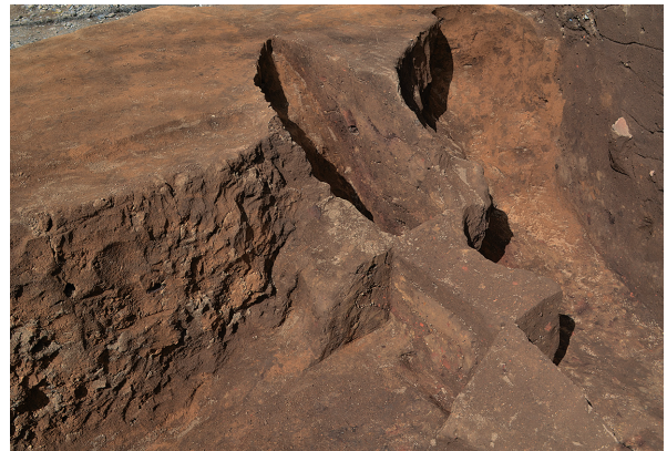
北区第3号竖穴建物跡旧竈土層・新竈袖土層（西から）
