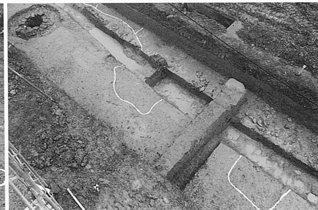
8 I区南 全景 (南東から)
