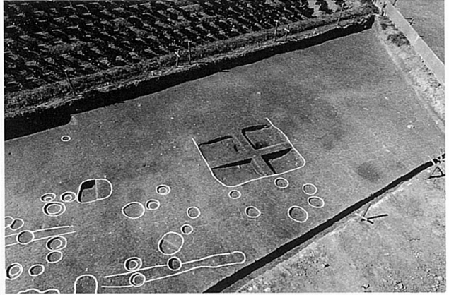
2 Y区 全景 (南東から)
