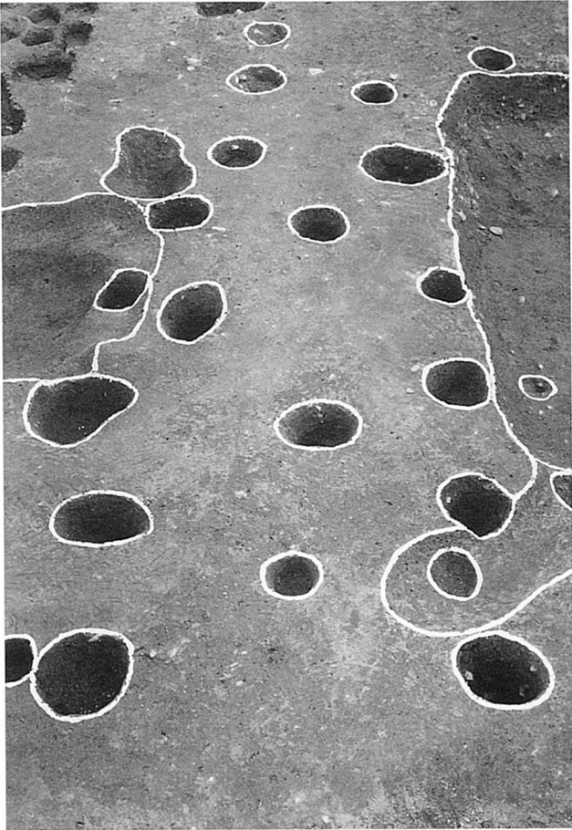
1 T区 掘立柱建物 51 (北西から)
