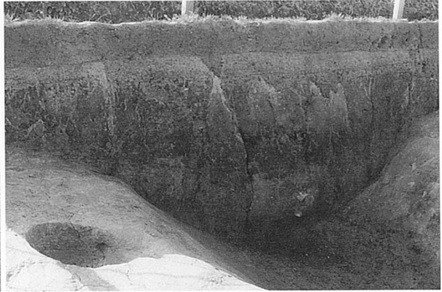
3 Y区 方形周溝墓1 周溝断面 (南西から)
