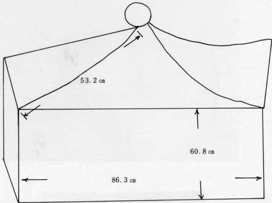
平面図⑩ セメント製寄棟式厨子（1959年製作）
