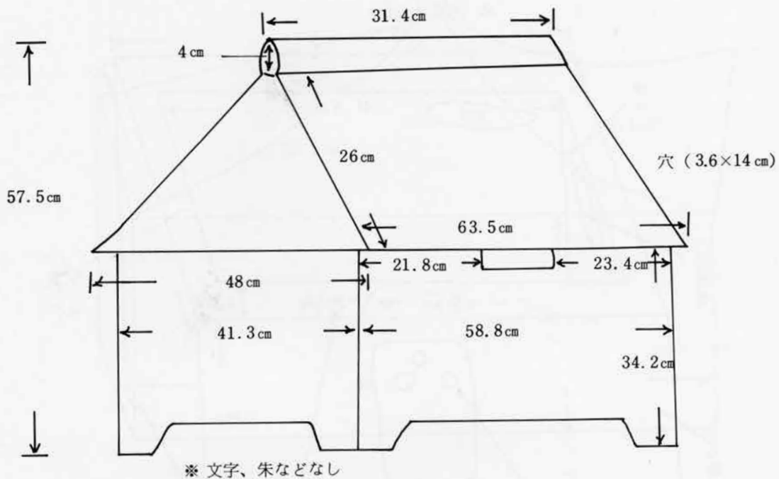
平面図⑧ 素焼寄棟式厨子
