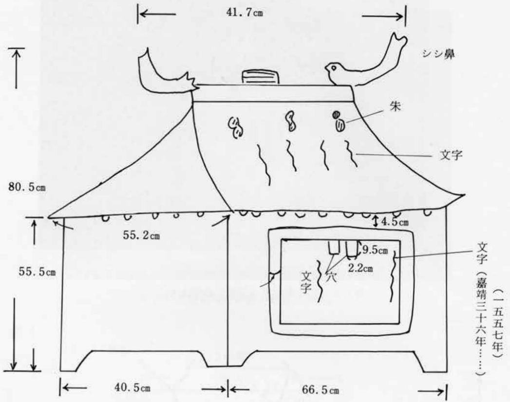
平面図③ 石灰岩製寄棟式厨子
