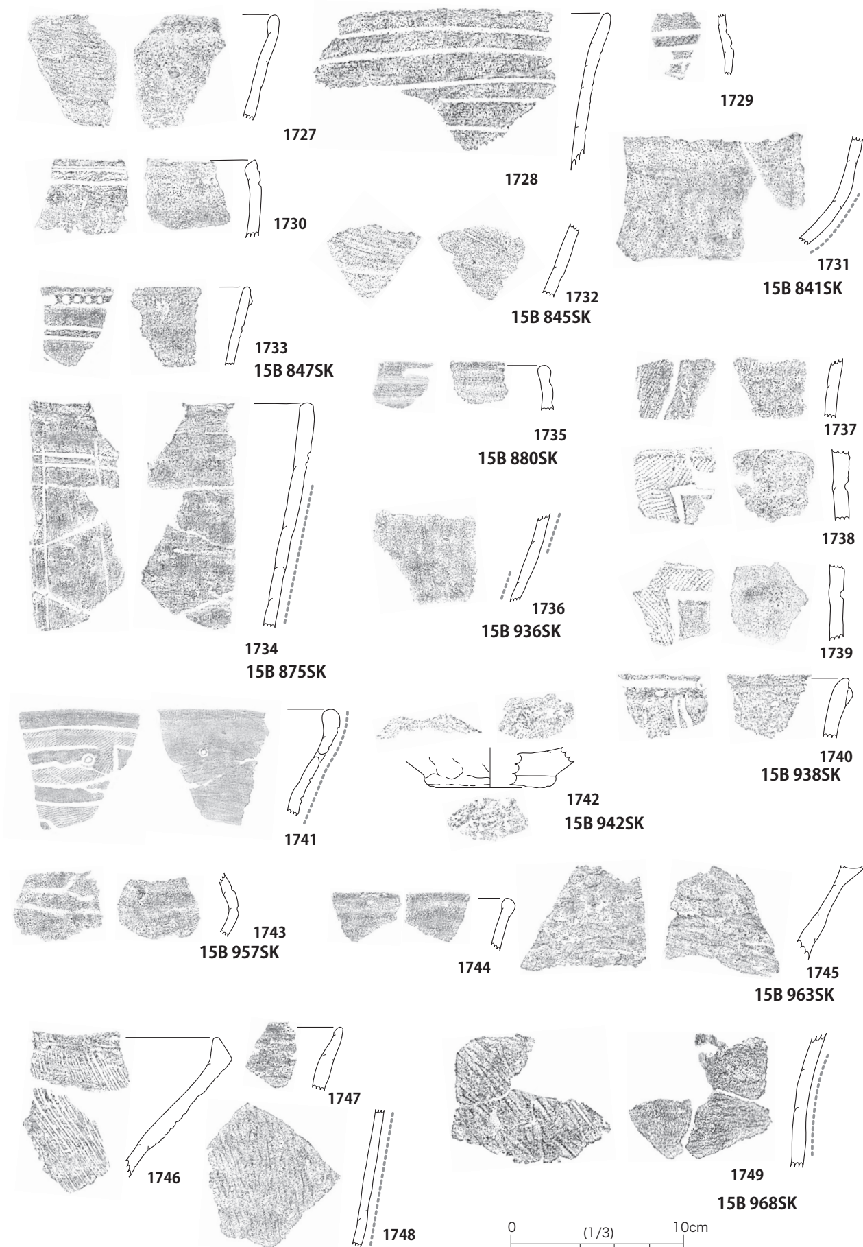
第 186 图 845SK 他出土土器
