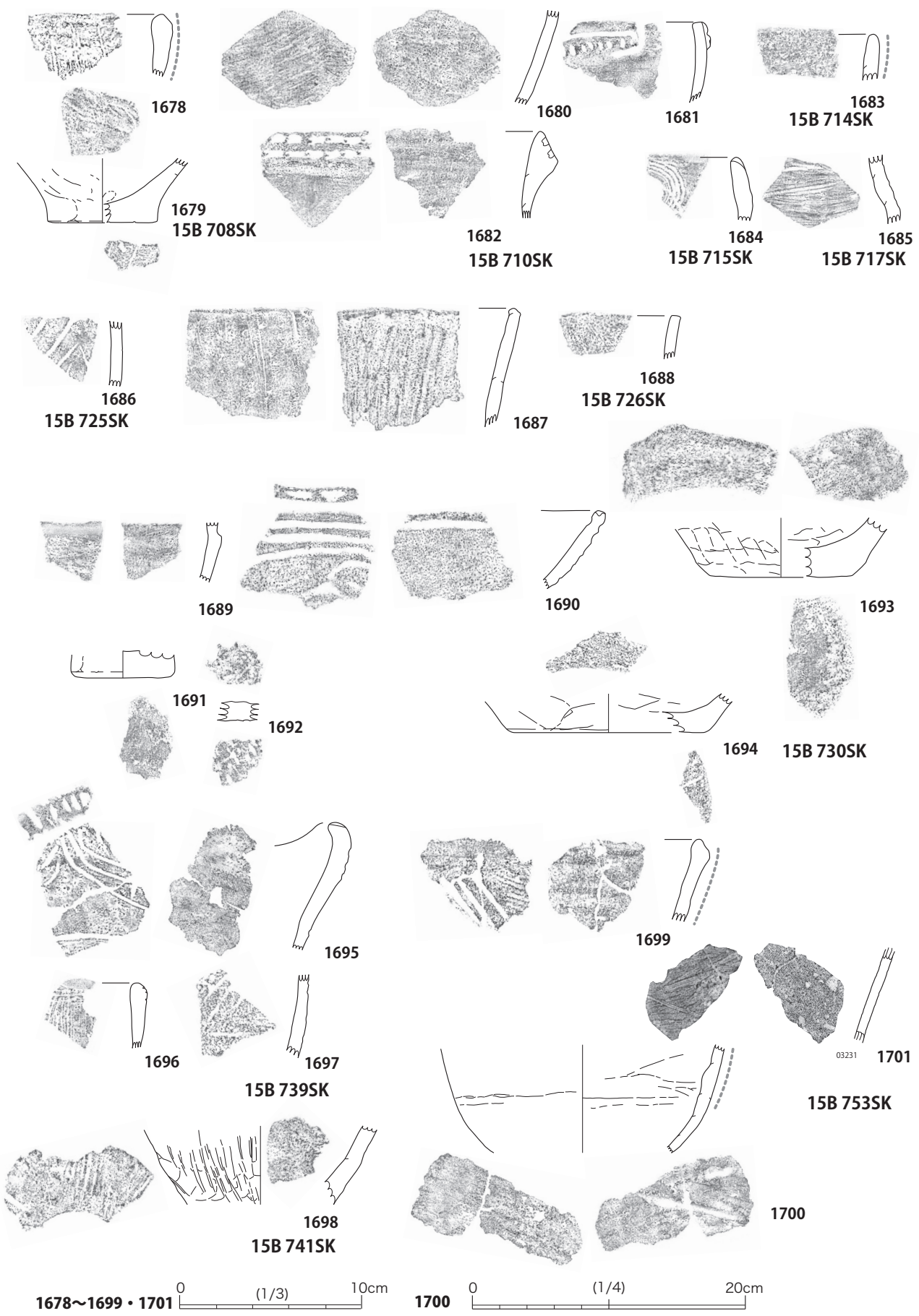
第 184 图 730SK 他出土土器
