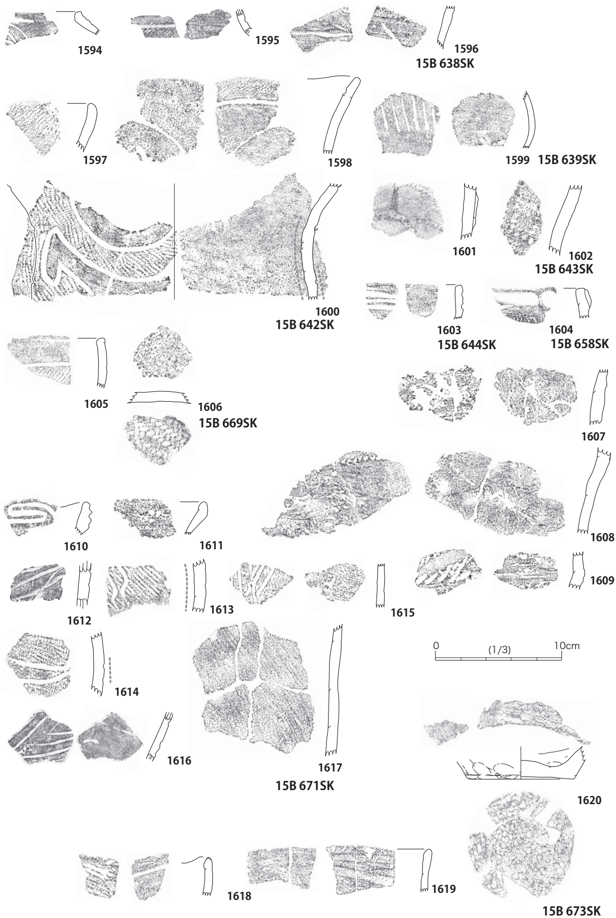
第 181 图 671SK 他出土土器
