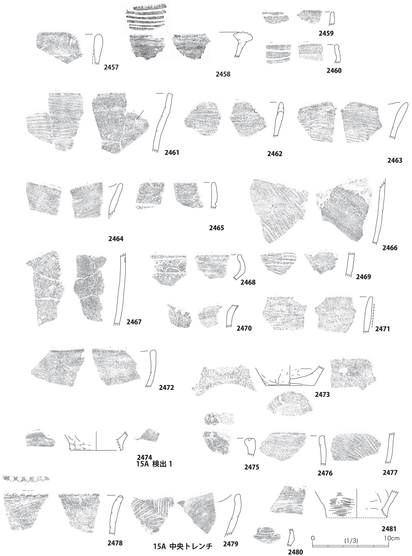
第 214 図 15A 区出土土器
