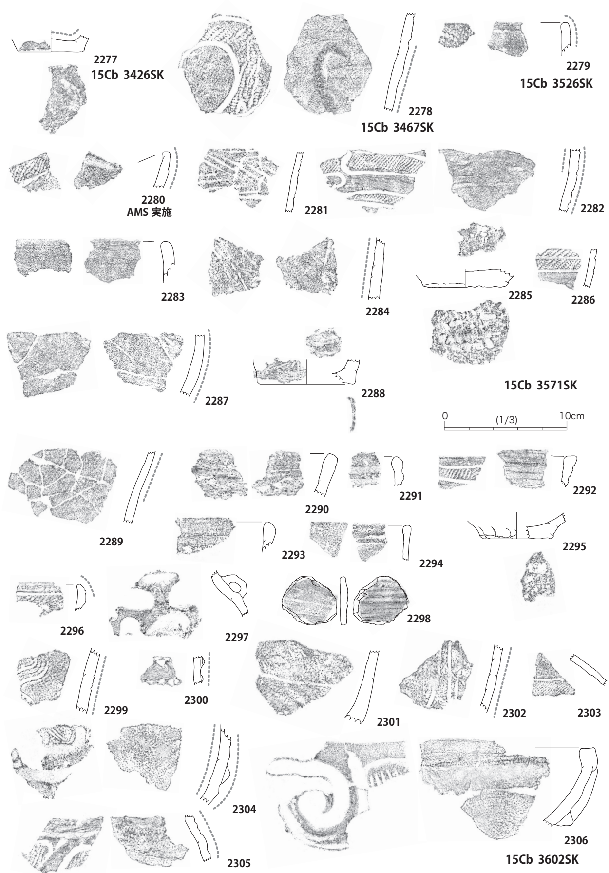
第 207 図 3602SK 他出土土器
