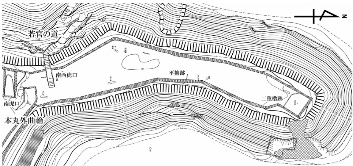
図23 北出丸測量図 (S=1/600)
