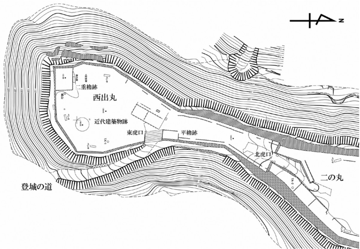
図20 西出丸測量図 (S=1/600)
