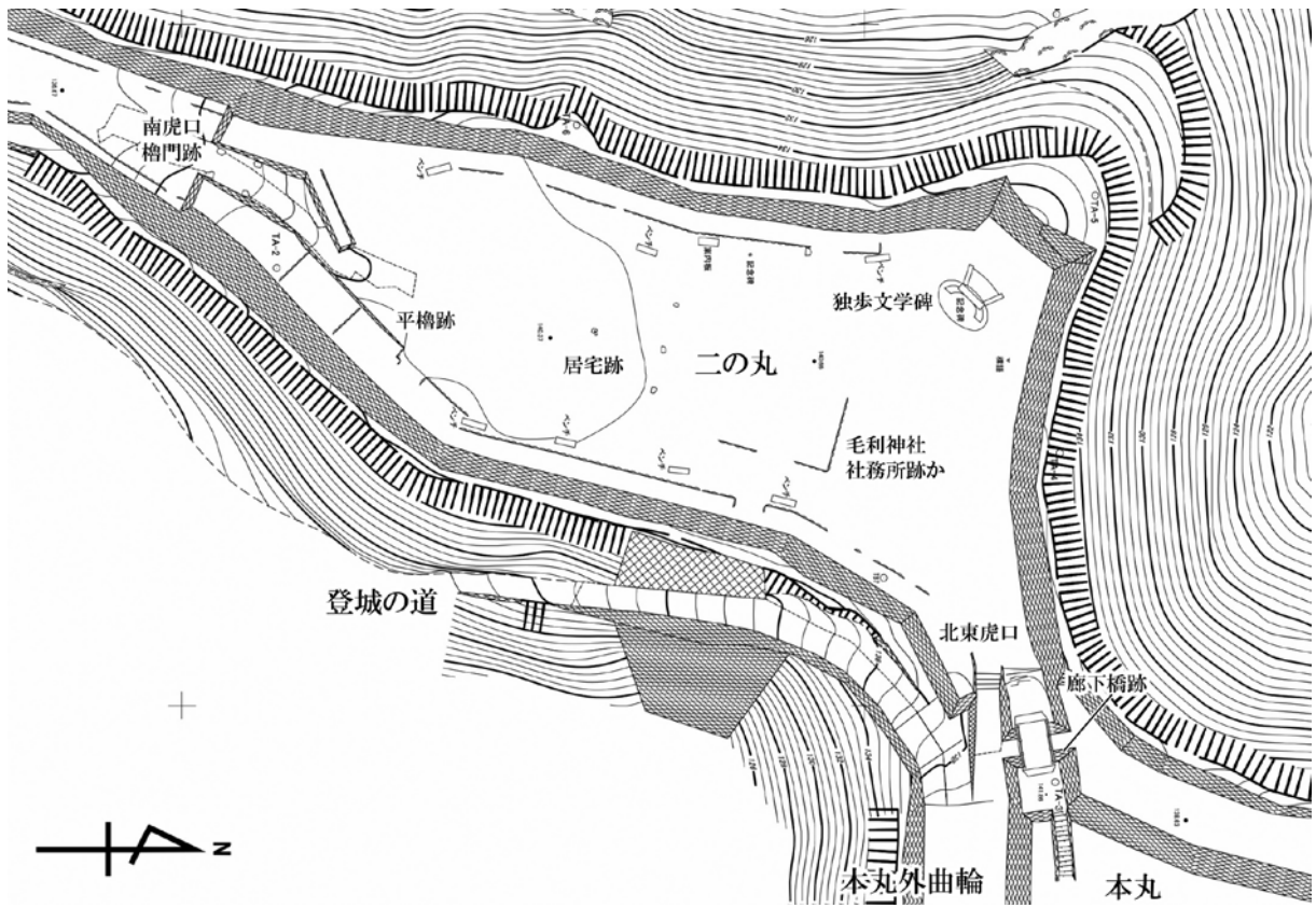
図17 二の丸測量図 (S=1/600)
