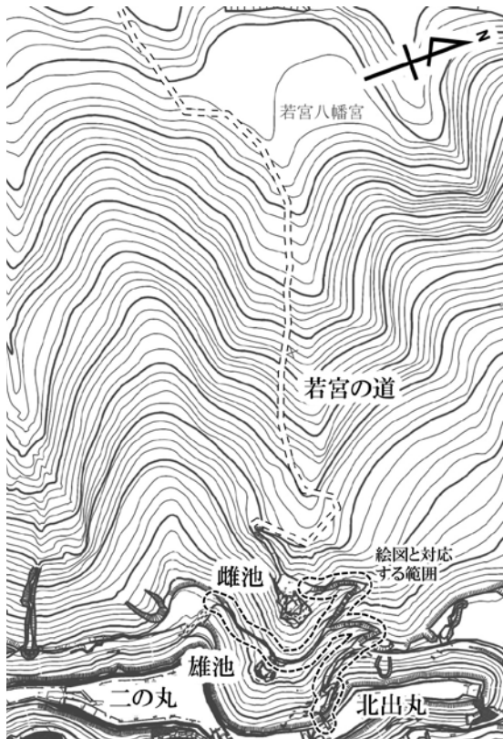
図39 若宮の道周辺測量図 (S=1/2,000)
