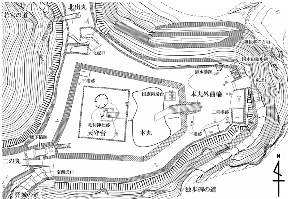
図15 本丸・本丸外曲輪測量図 (S=1/600)
