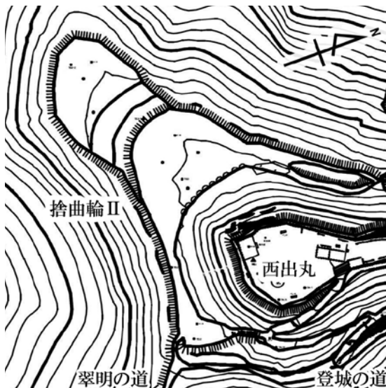
図27 捨曲輪 II 測量図 (S=1/1,500)
