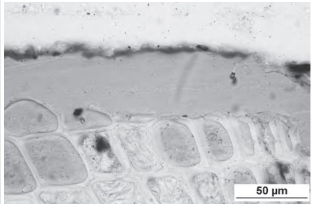
3 曲物底板 (16) 内面漆塗膜構造
