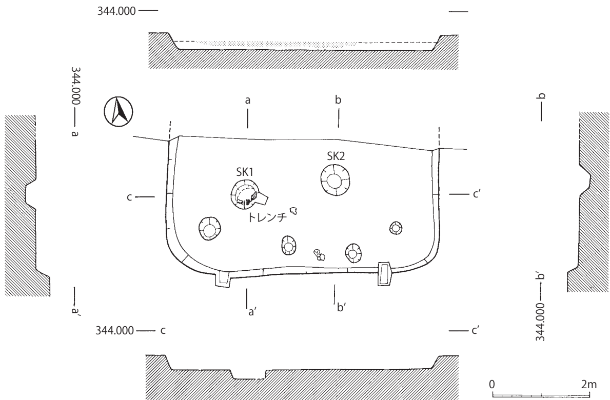
図12 2-SB4実測図（1：80）
