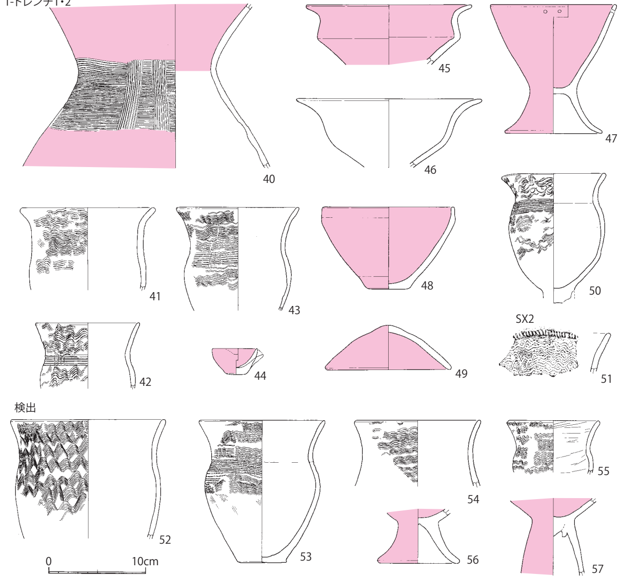
図15 土器実測図3 (1:4)
