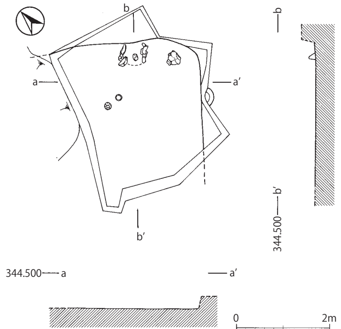
図6 1-SB1 実測図 (1:80)
