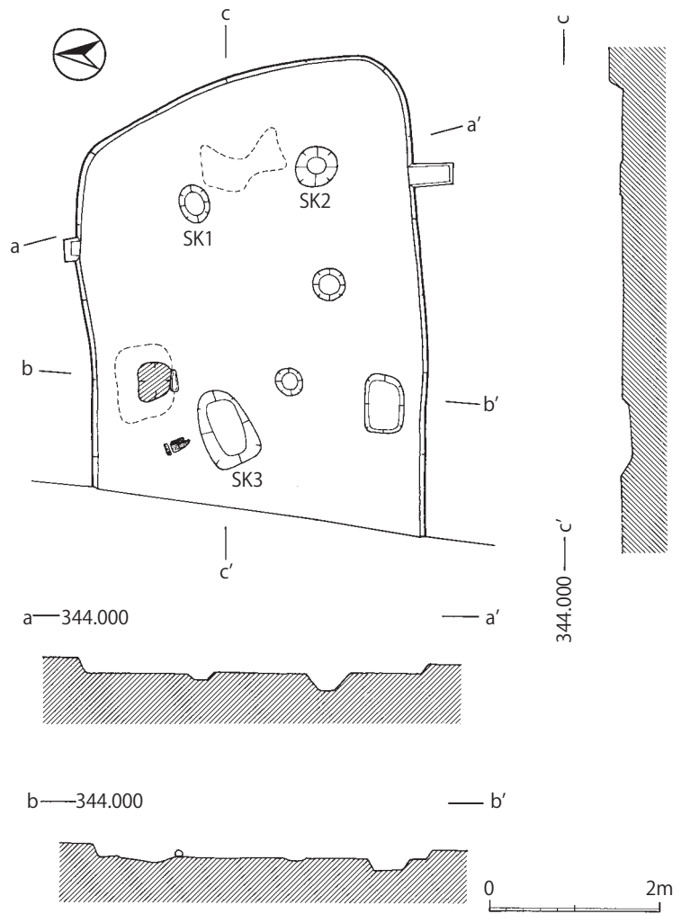
図11 2-SB3実測図（1：80）
