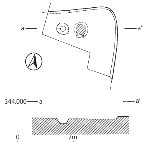
図9 2-SB1実測図(1:80)
