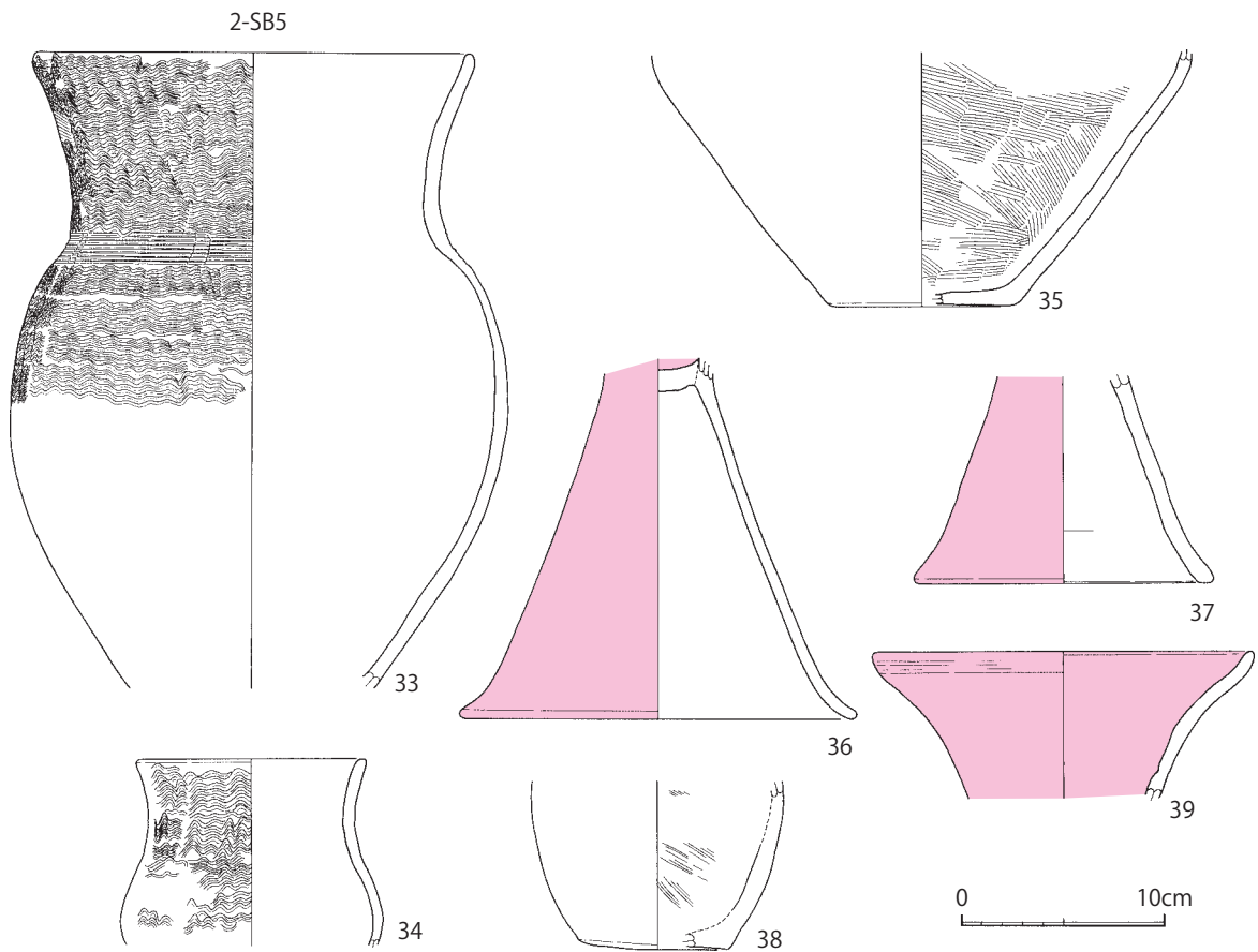
图14 土器实测图2 (1 : 4)
