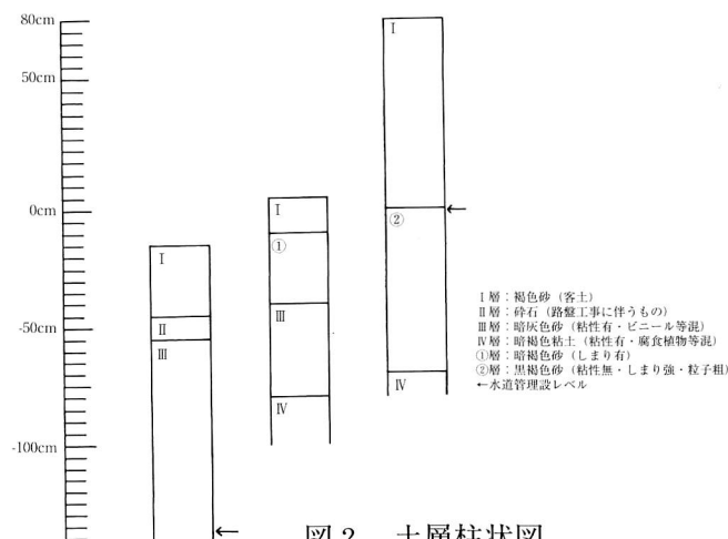
図 2 土層柱状図
