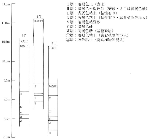
図2 土層柱状図
