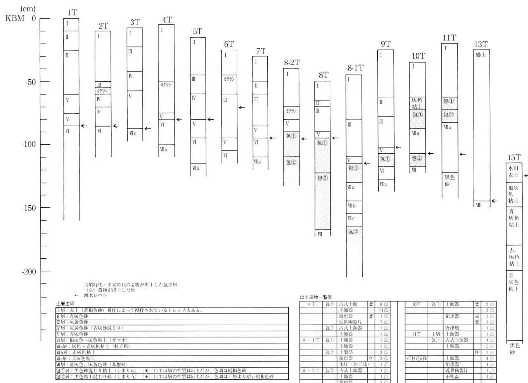
図3 土層柱状図
