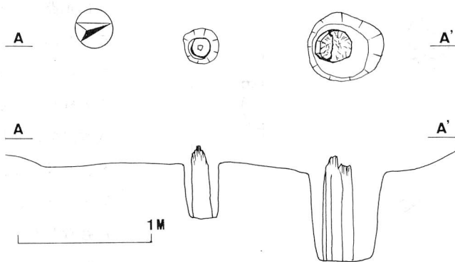
Fig. 8 柱列 平断面図
