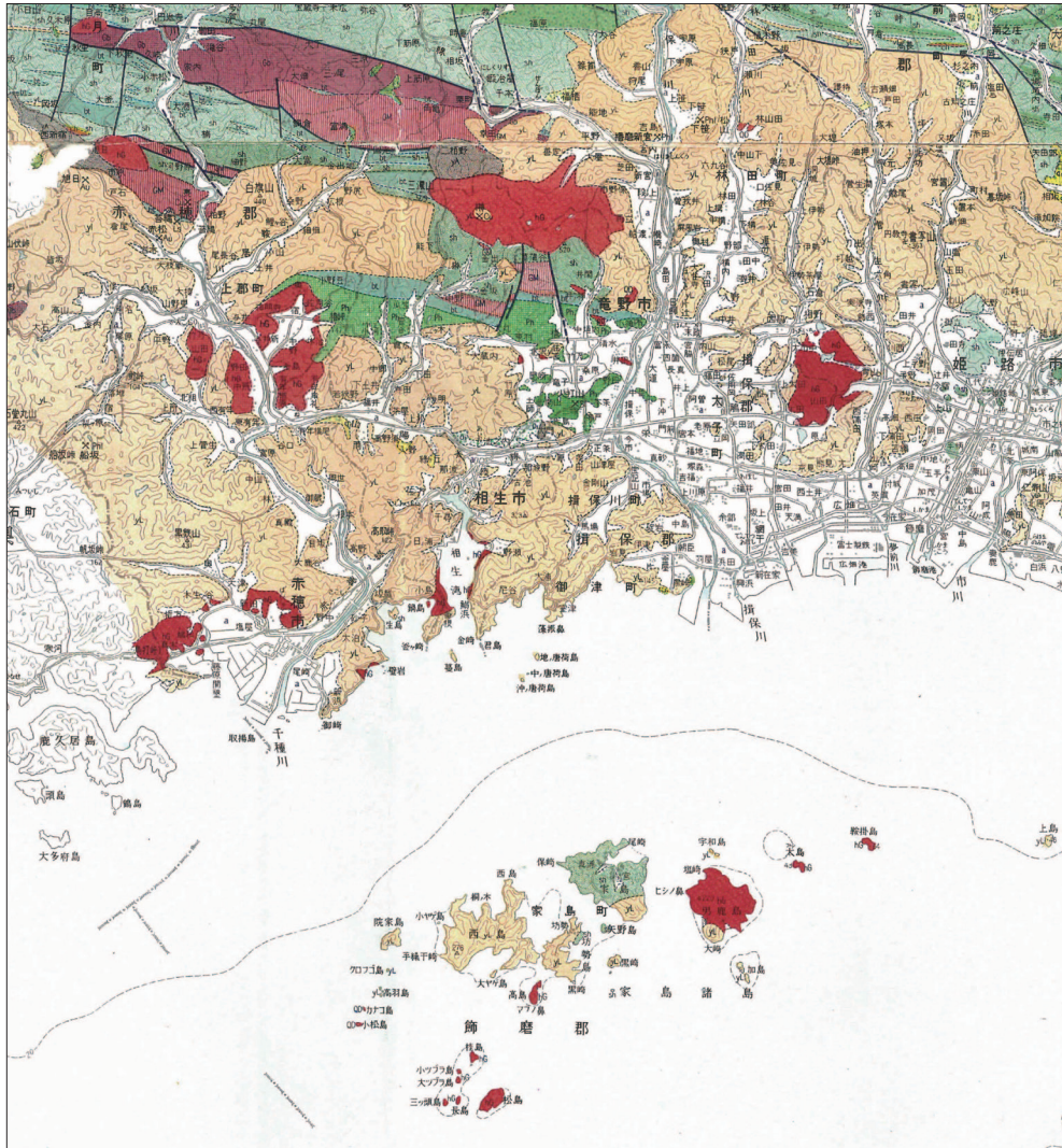
図2 西播磨の地質図
