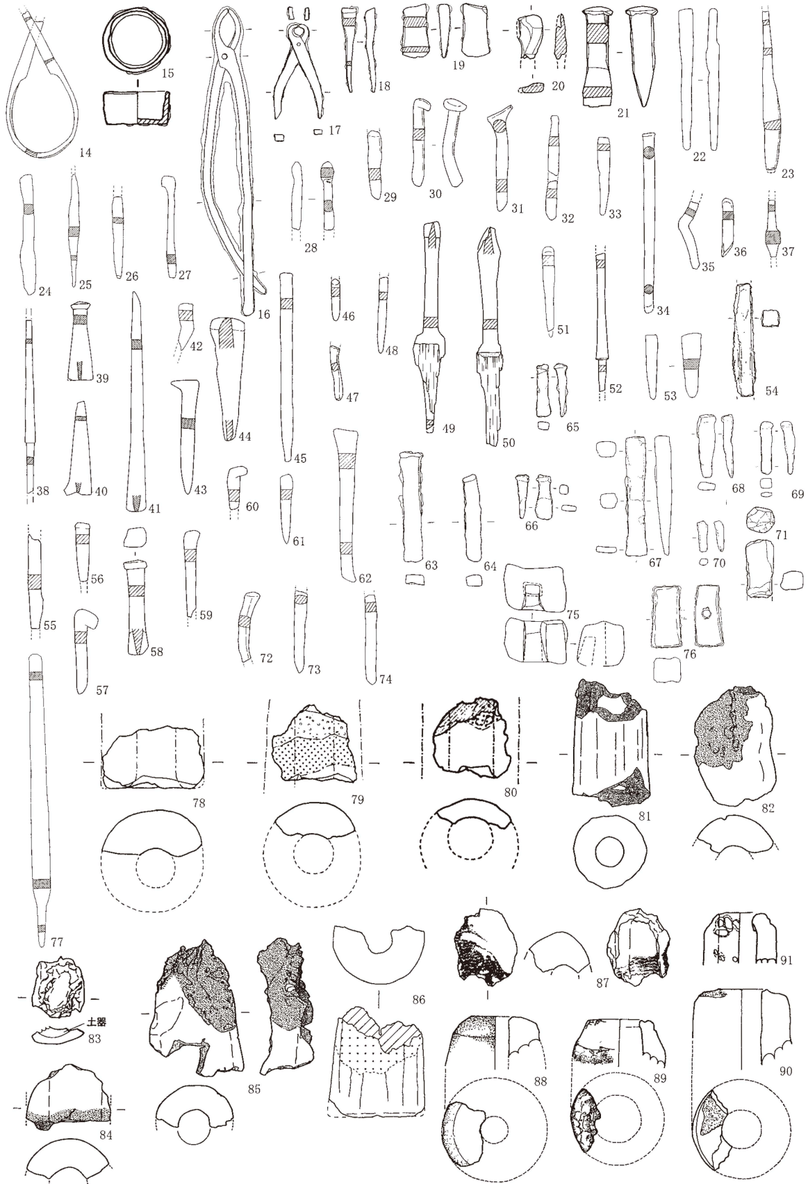
第2図 鉄生産関連遺物2
