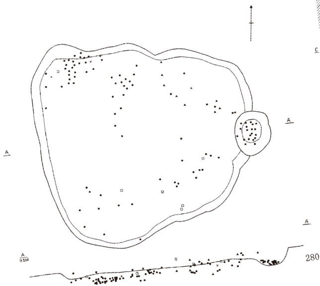
第6図 鉄生産関連遺構 1
