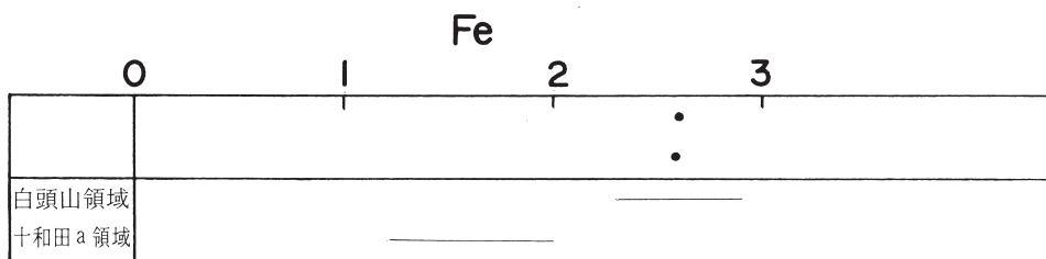
図168 Fe 因子の比較
