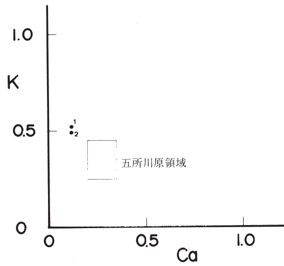
図169 K - Ca 分布図
