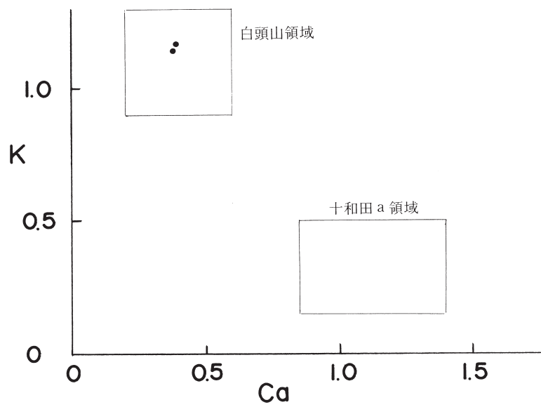
図166 K - Ca 分布図
