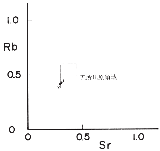
図170 Rb - Sr 分布図
