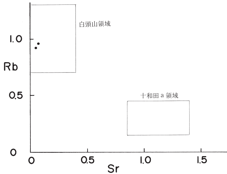
図167 Rb - Sr 分布図
