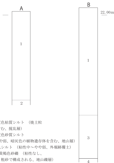
第5図 土層柱状図 (S=1/50)
