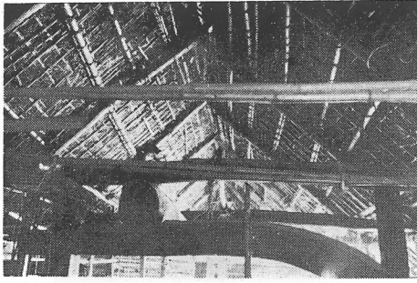
⑤ 森田半三郎家 相イ欠キのサスグミ
