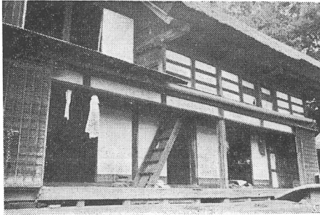
⑫ 諸田泰三家の軒セガイ・化粧ヌキと白カベ・エンガワにハシコダン
