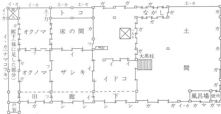
今井竹蔵家階下間取図(南牧村大仁田)
