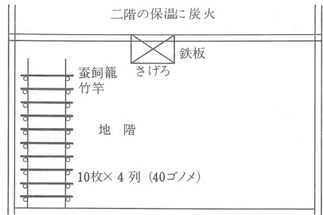
蚕室立面図 (塩沢、飯塚宇太郎家)
