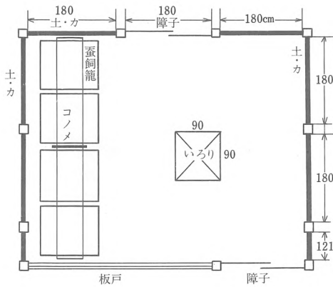
蚕室平面図 (塩沢・飯塚美治家)
