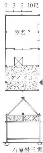
図1 1間取の民家（復原図）
