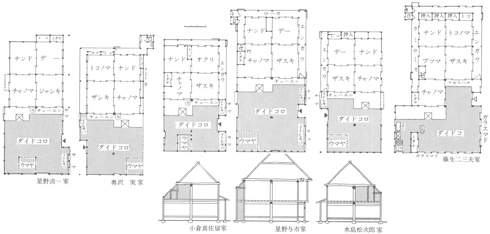
図8 整形田字平面の民家（平面・断面図）
