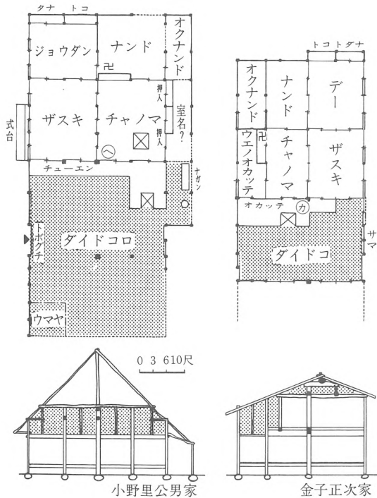
図9 多間取平面の民家（平面・断面図）
