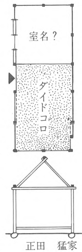
図1 1間取の民家（復原図）
