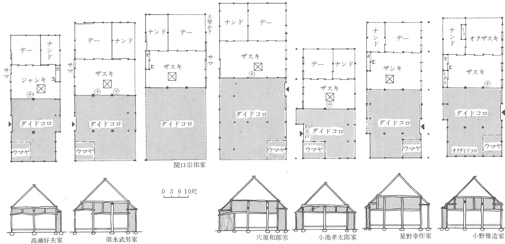
図3 広間型の民家（復原平面・断面図）
