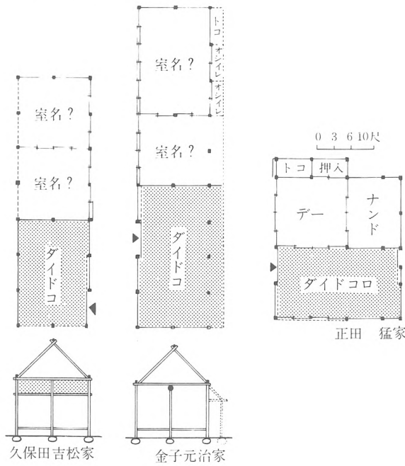
図2 二間取民家（復原図）
