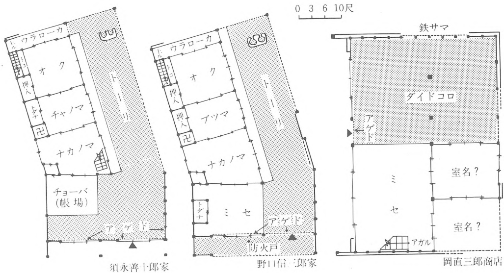
図10 町家（平面・断面図）
