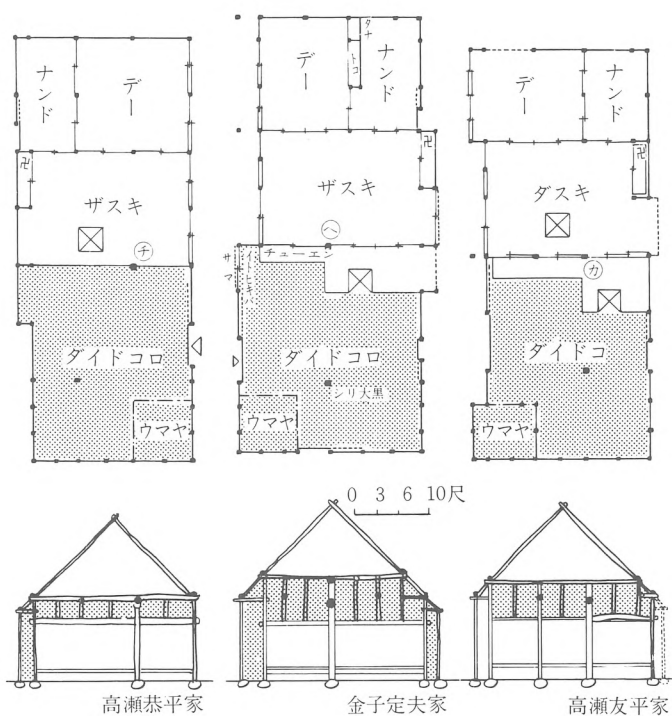
図4 広間型の民家（復原平面・断面図）
