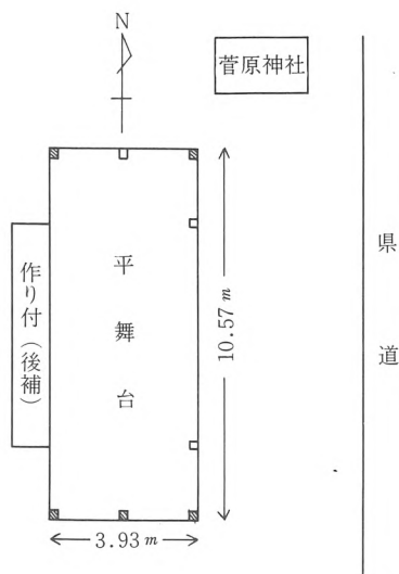
浅原舞台の平面図
