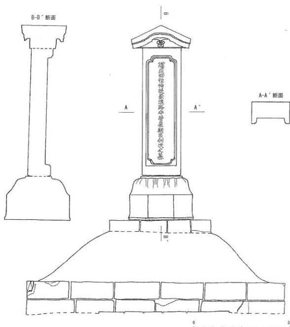
図3 初代藩主利次墓 【立面図】(1:80)
