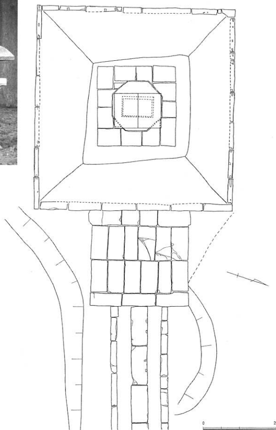
同左【平面図】(1:100)
