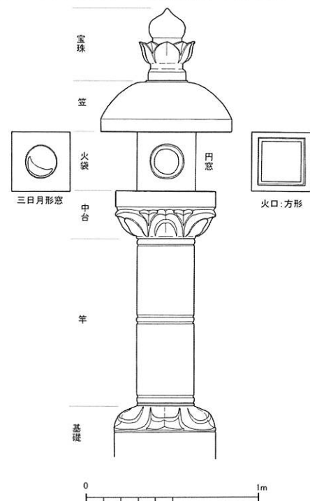
図 6 藩主墓前燈籠・初代利次墓 (1:30)
