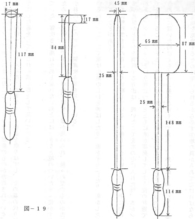
丸ごて キセル型丸ごて 平ごて
