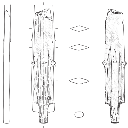
8 銅剣形石製品実測図 (S = 1/4)
