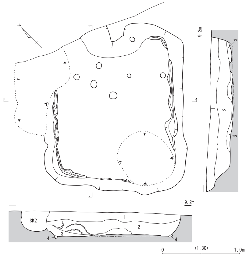
図7 SH6 炭・焼土検出状況平・立面図
