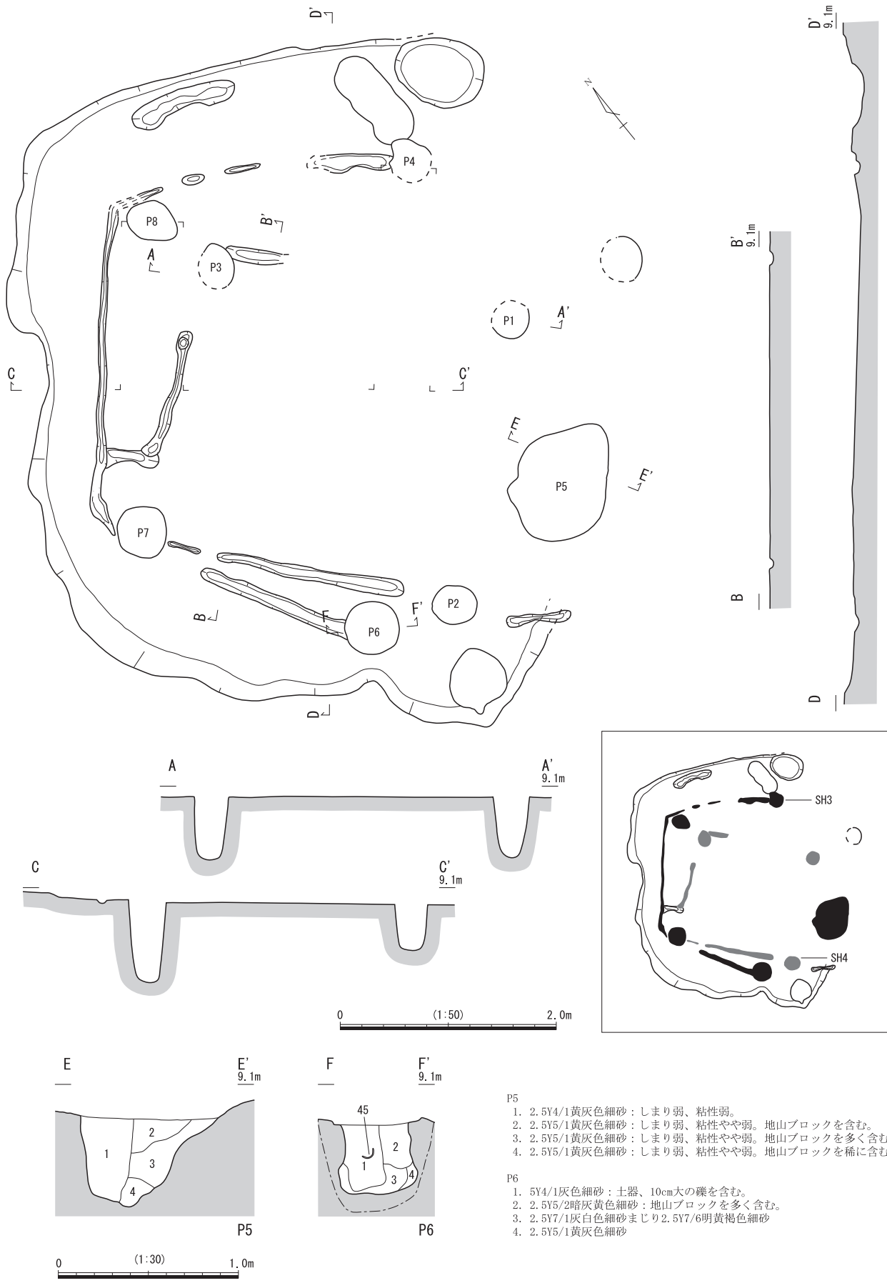
図12 SH3・4 平・断面図
