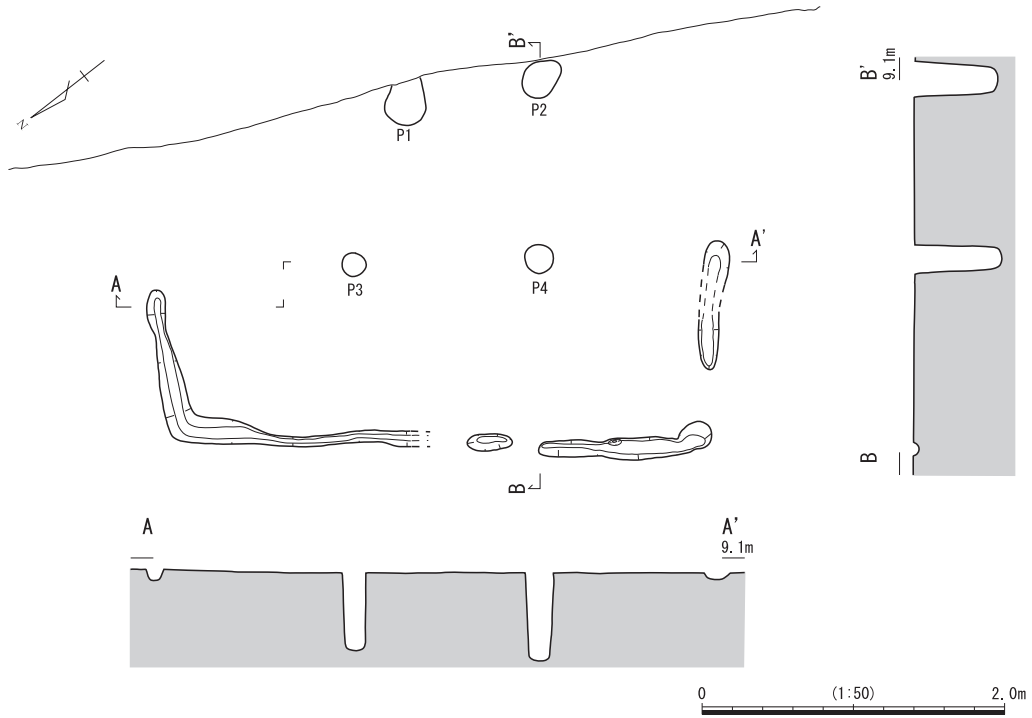
図14 SH1(古) 平・断面図
