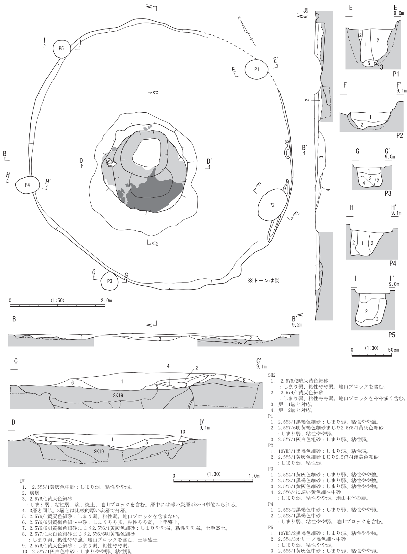
図13 SH2 平・断面図
