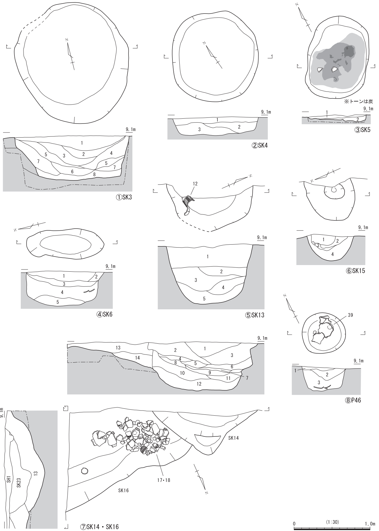
図5 遺構平・断面図
