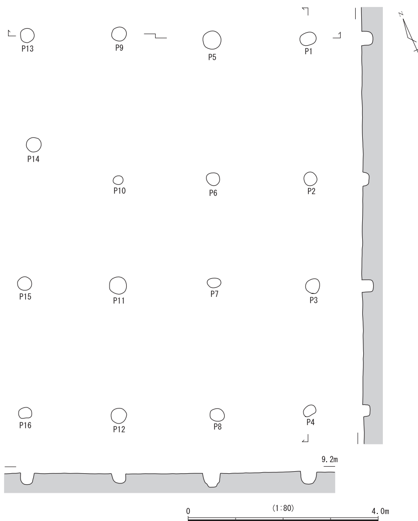
図18 SB1 平・断面図
