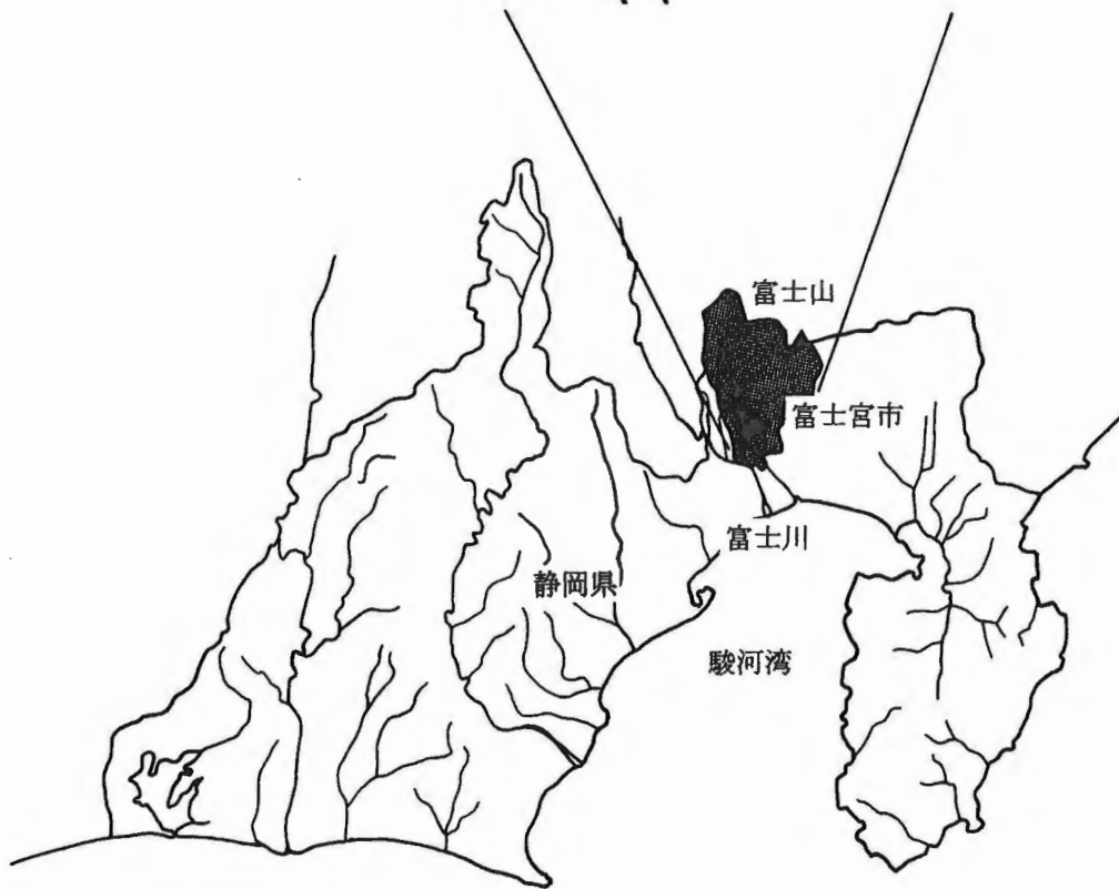
図2 遺跡周辺の地質図
