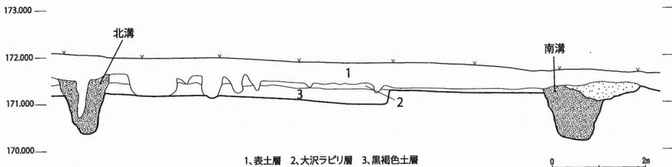
図10 方形周溝墓02東壁土層断面図
