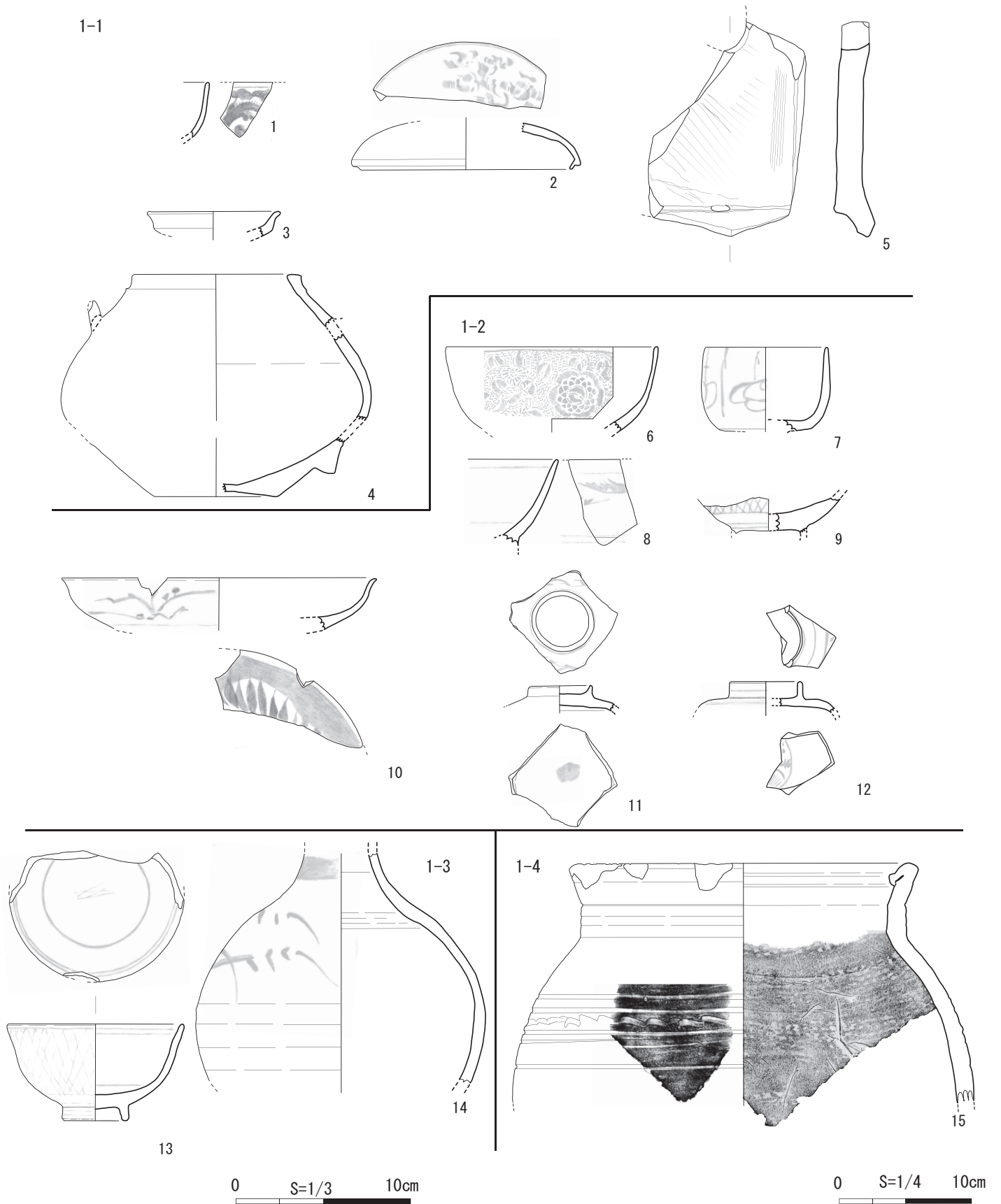
第50図 大渡野番所跡採集遺物実測図（1～14はS=1/3、15はS=1/4）
