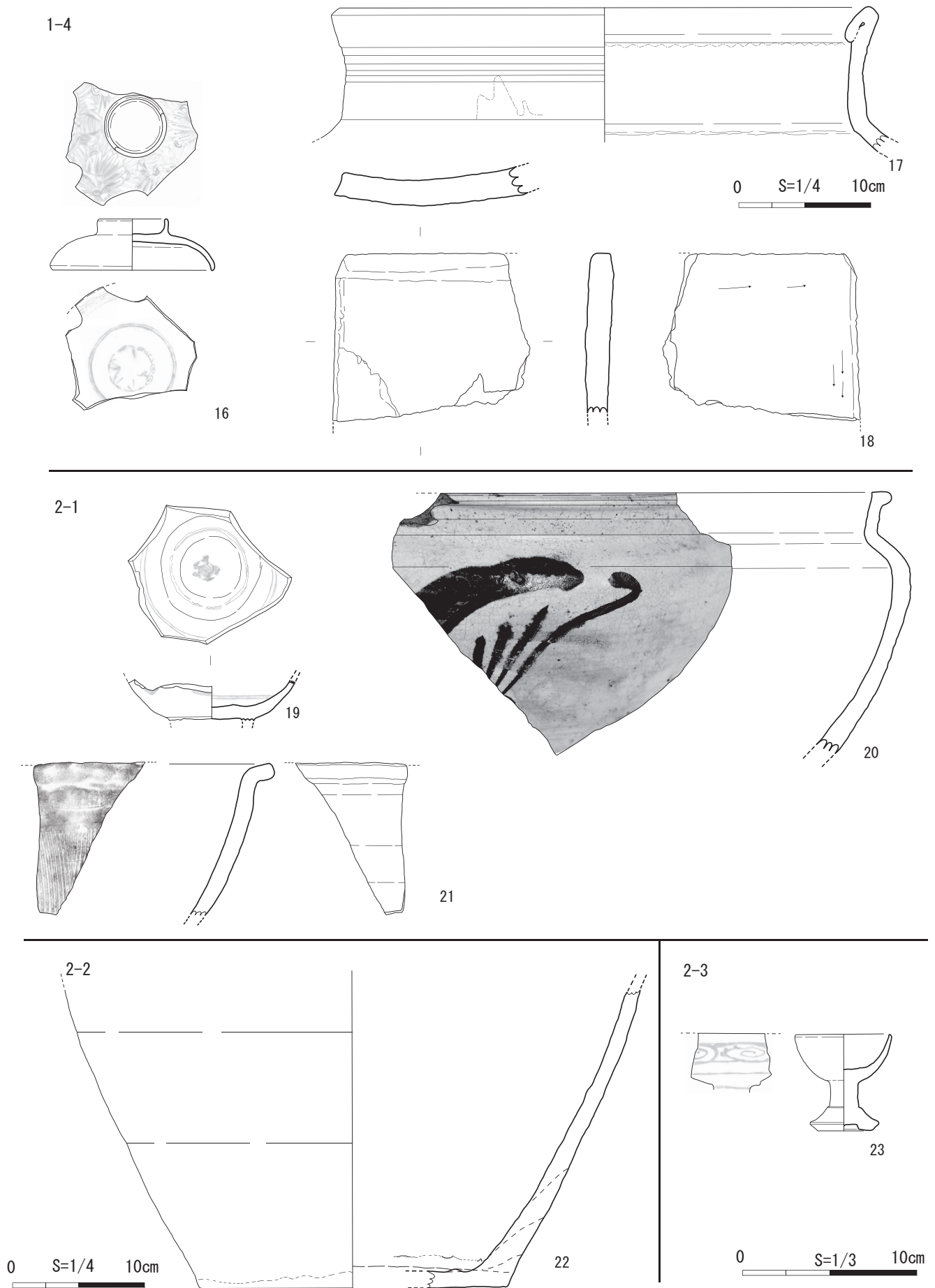
第51図 大渡野番所跡採集遺物実測図（18, 19~21, 23はS=1/3、17, 22はS=1/4）
