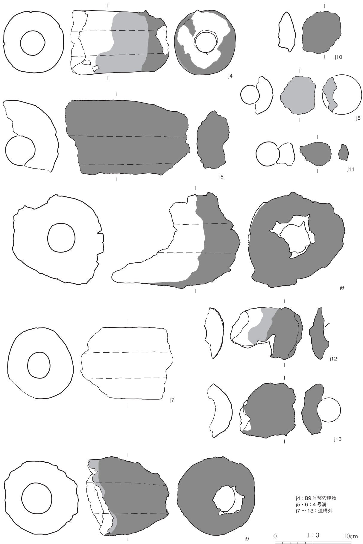
第 390 図 羽口 (2)
