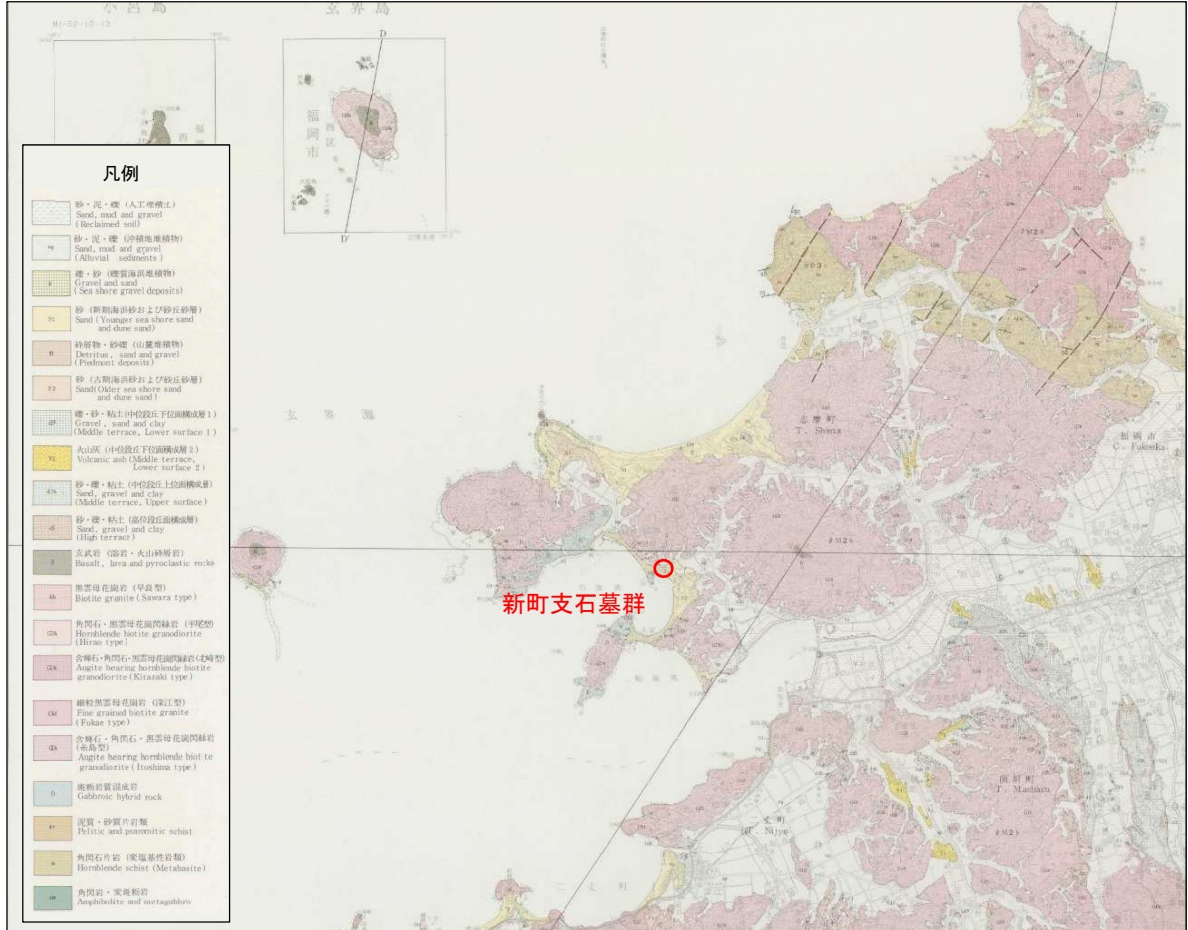
図 2-3 表層地質図
