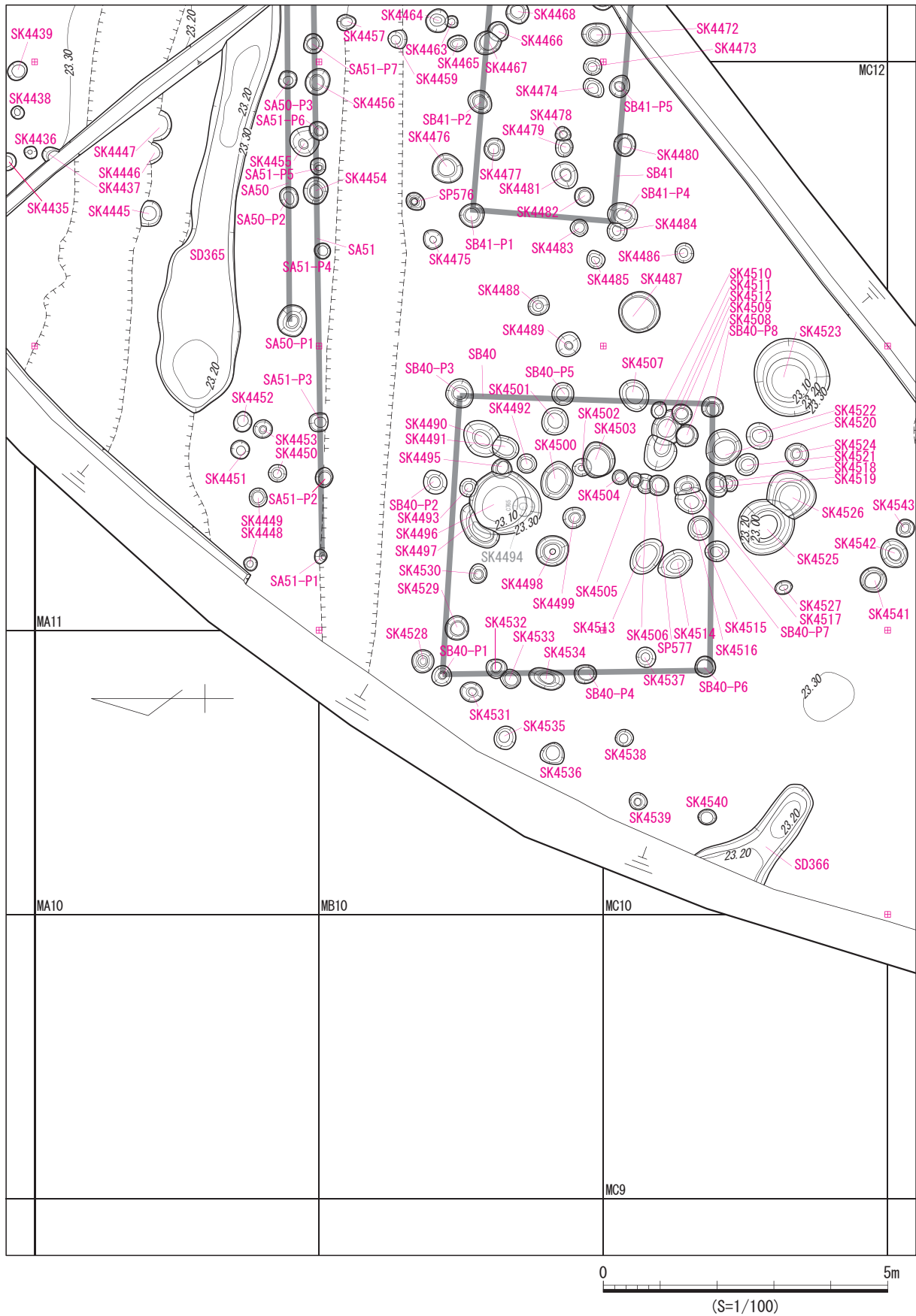
图 766 発掘区全域図 3・4 地点 分割図 3
