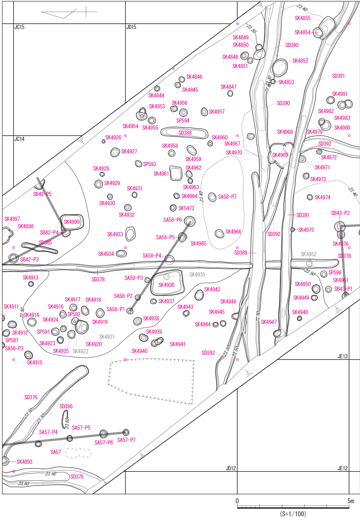
图 777 发掘区全域图 3·4 地点 分割图 14
