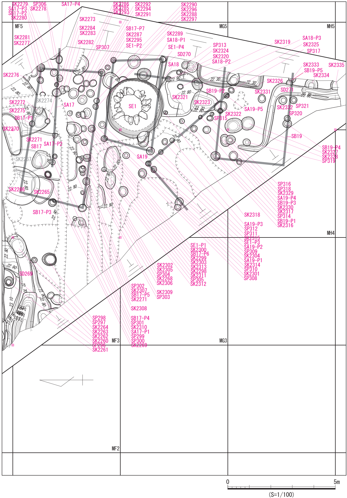
図 804 発掘区全域図 1・2・13・20・21 地点 分割図 10
