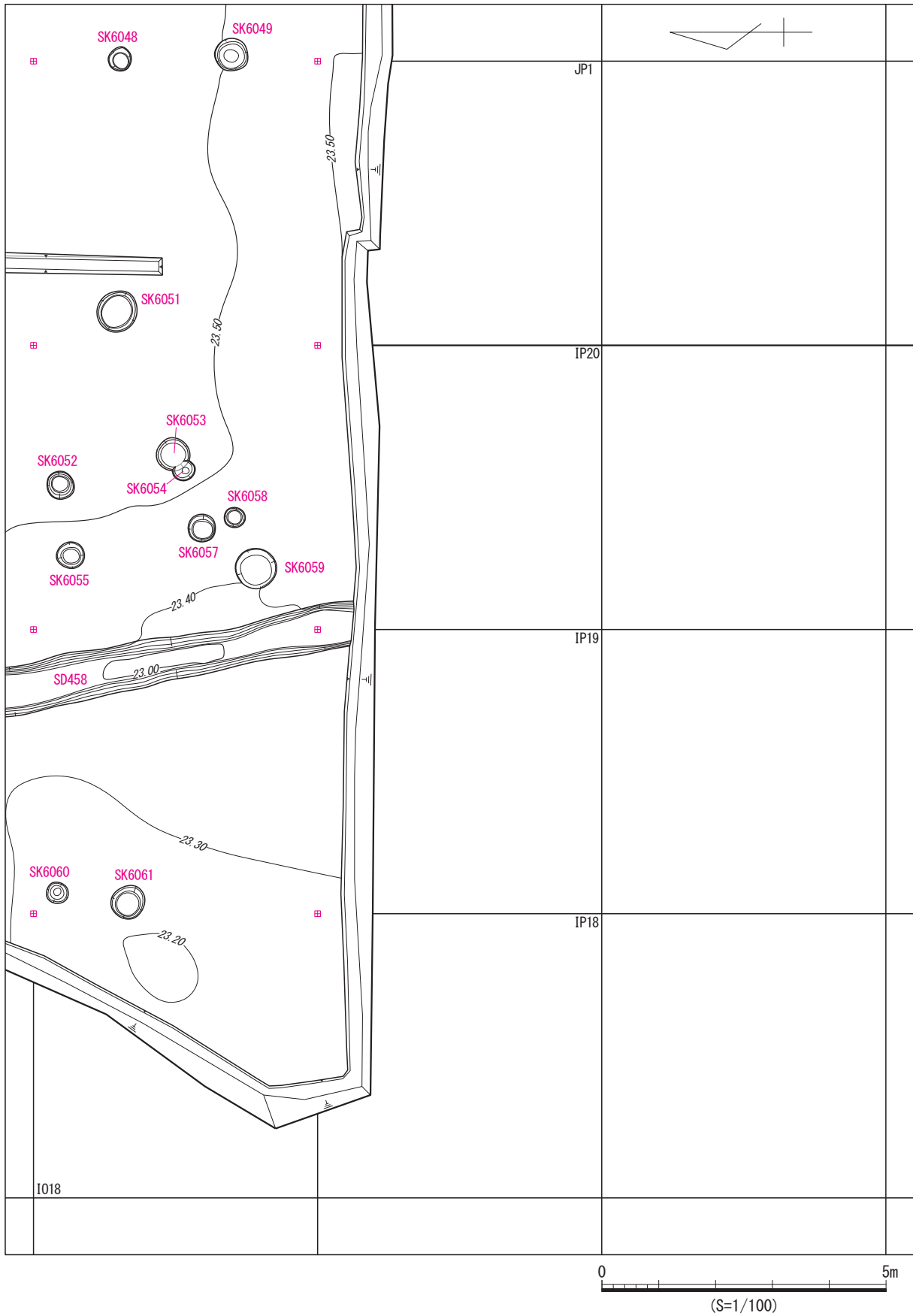
図 792 発掘区全域図 3・4地点 分割図 29
