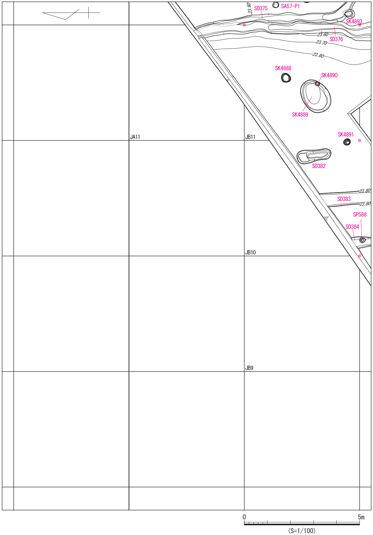
图 771 発掘区全域図 3・4地点 分割図 8
