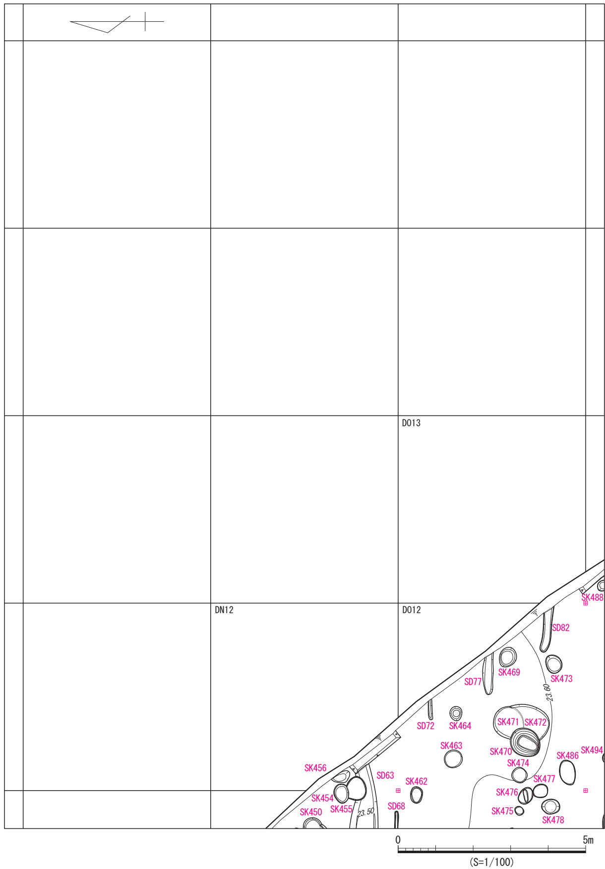
图 732 発掘区全域図 6～8・17・18 地点 分割図 3
