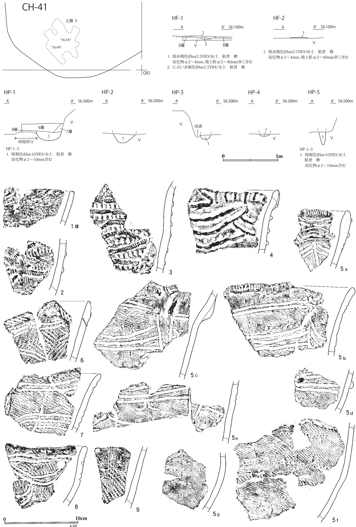
図 II-236 CH-41遺構図(2)・CH-41の遺物(1)
