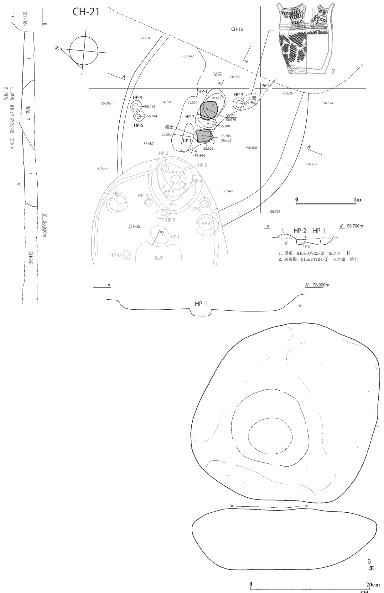
図 II-103 CH-21遺構図・CH-21の遺物(1)
