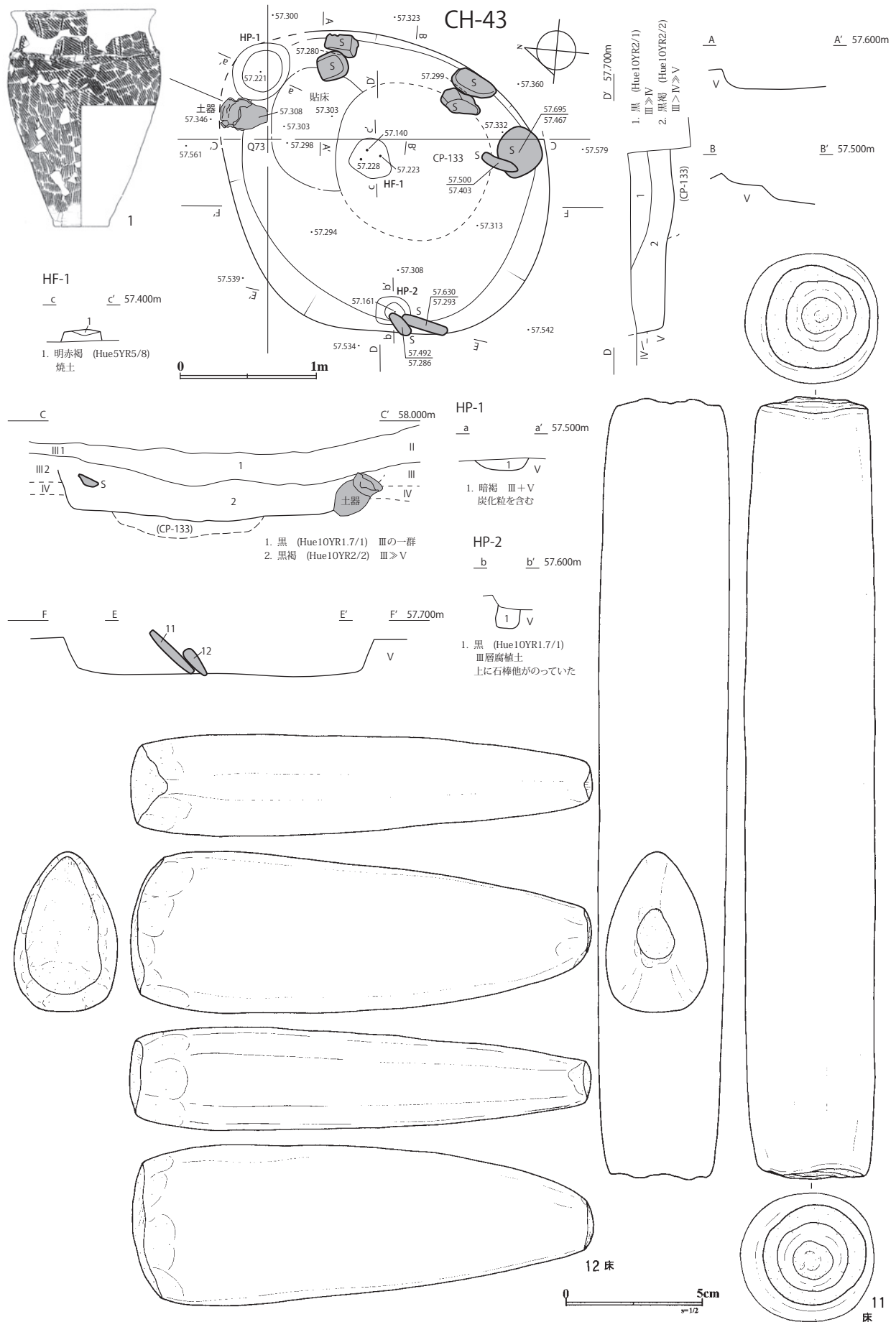
図II-238 CH-43遺構図・CH-43の遺物(1)
