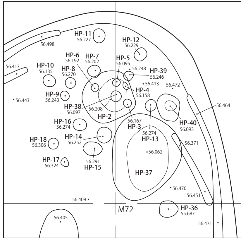
HP-2 周辺詳細図 (1/20)
