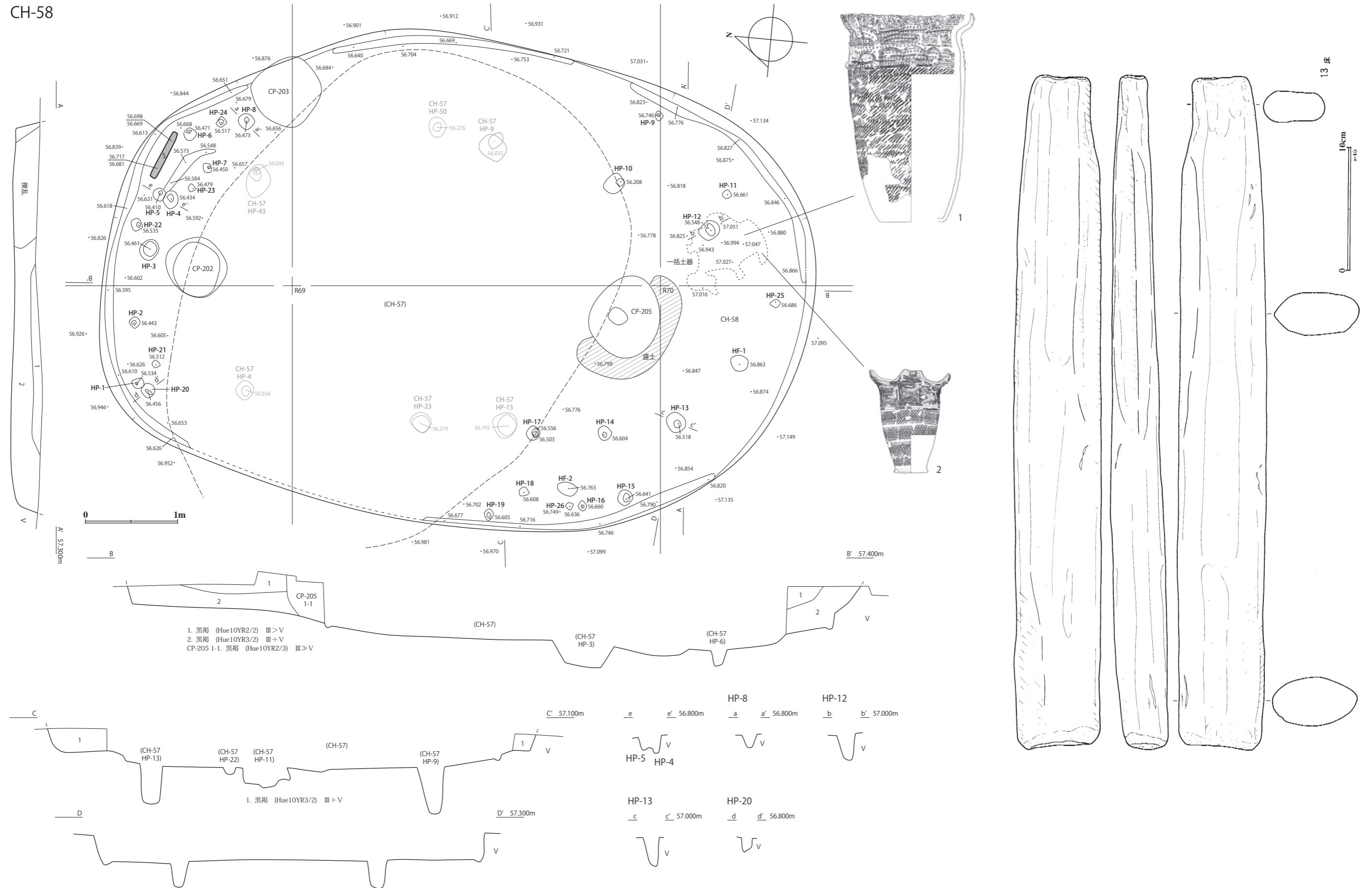
図 II-322 CH-58遺構図・CH-58の遺物(1)
