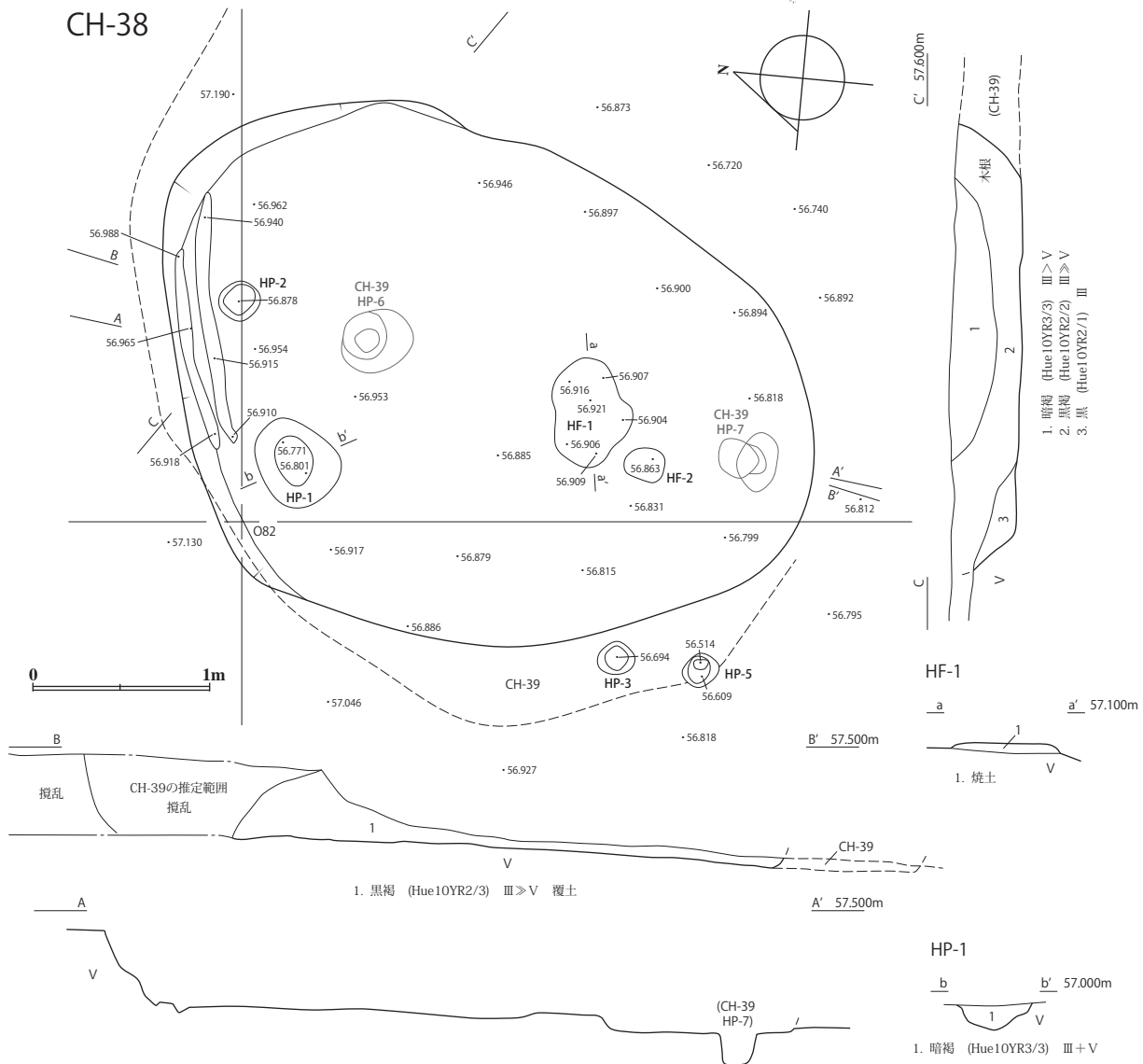
図 II-224 CH-38遺構図・CH-38の遺物
