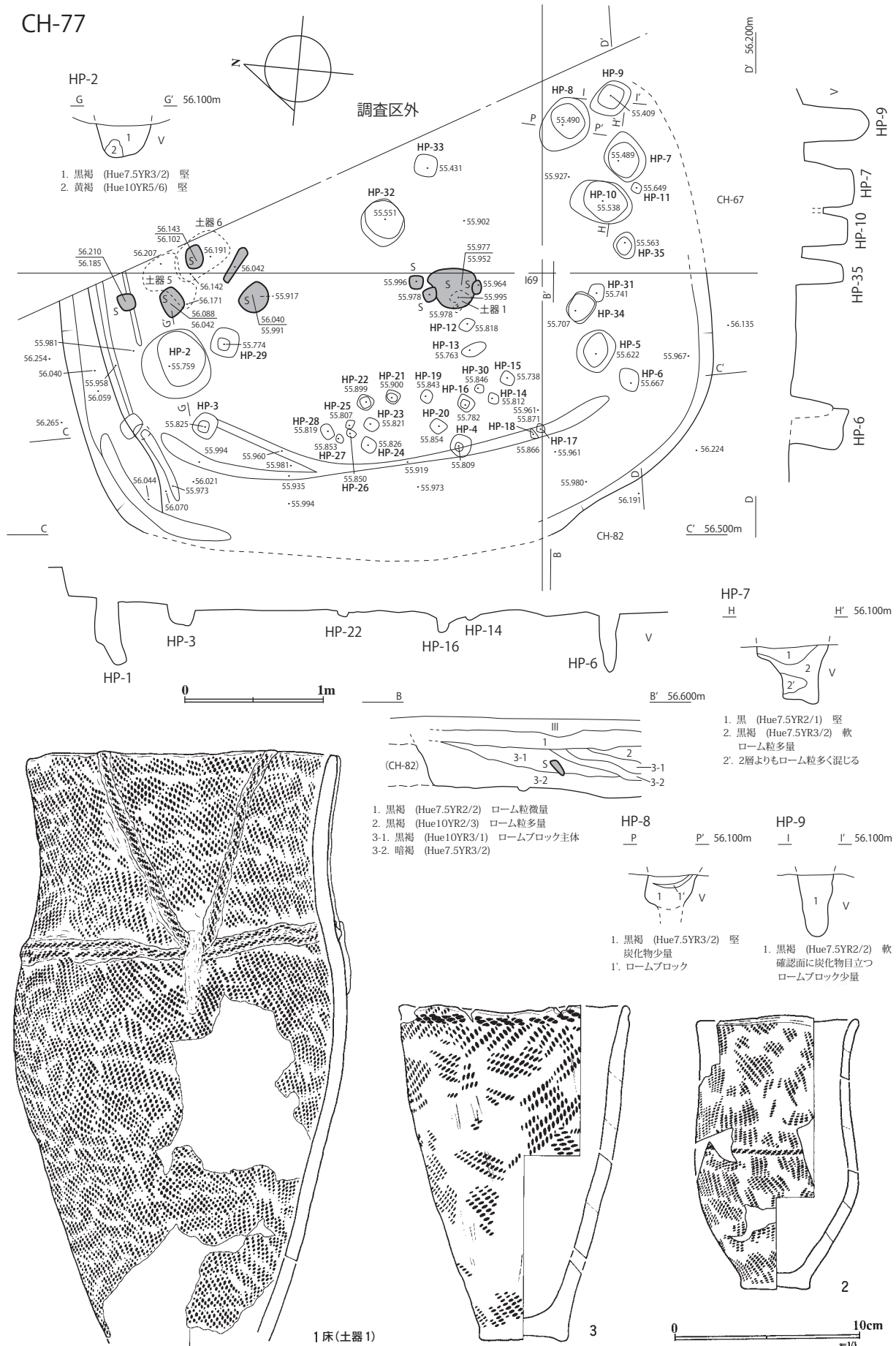
図II-388 CH-77遺構図・CH-77の遺物(1)
