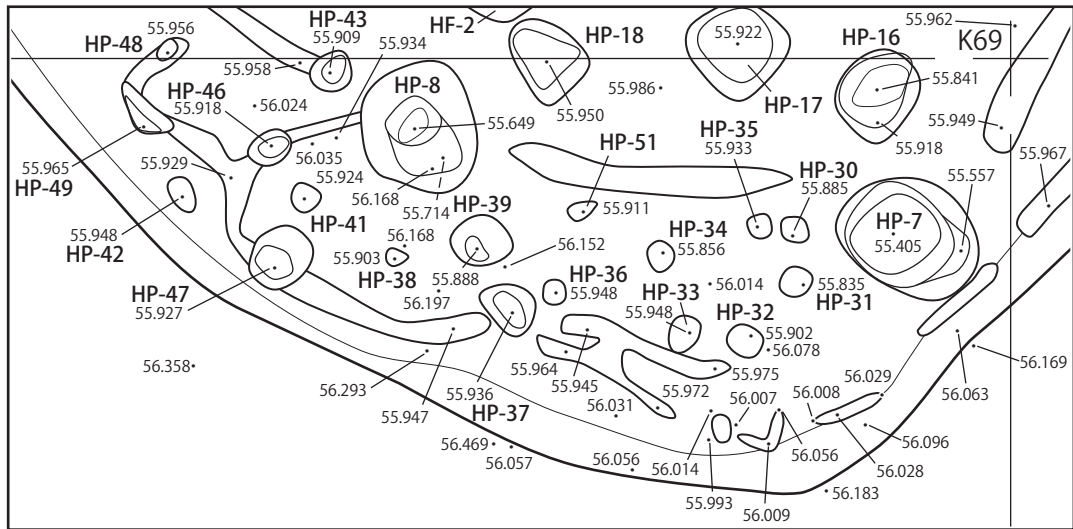
HF-1 周辺詳細図 (1/20)
