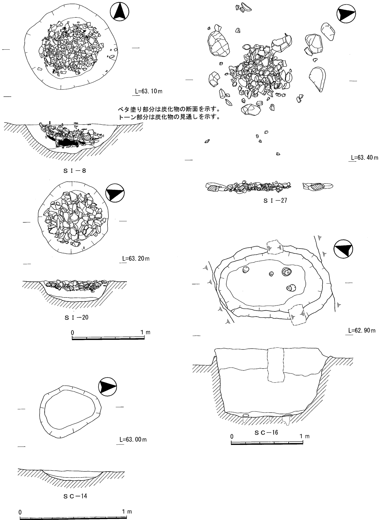
第12図 下猪ノ原遺跡SI-8. 20. 27. SC-14. 16実測図 (S=1/30・1/20)
