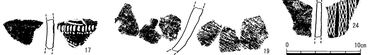
第13図 下猪ノ原遺跡出土縄文時代早期遺物実測図 (S = 2/3 · 1/3)
