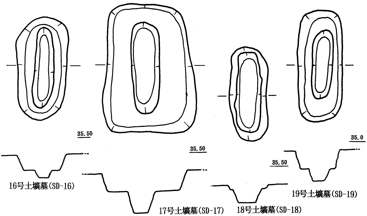
第84图 東原F地点 土墳墓实测图(3) (S=1/50)
