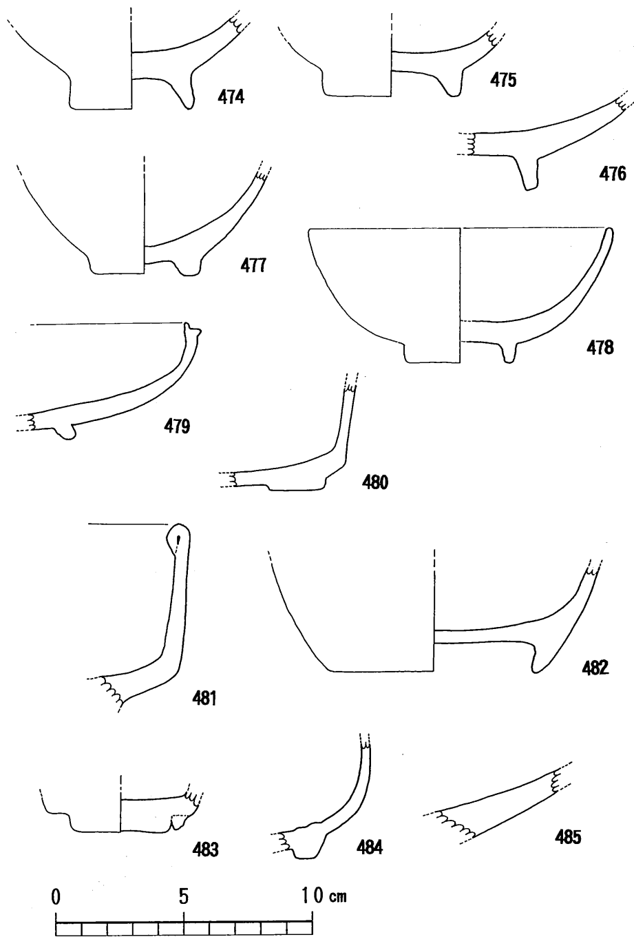
第99図 東京F地点 遺構に伴わない陶磁器片実測図(2)
