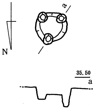
第60图 2号土壇(SC-2)実測図 (S=1/50)
