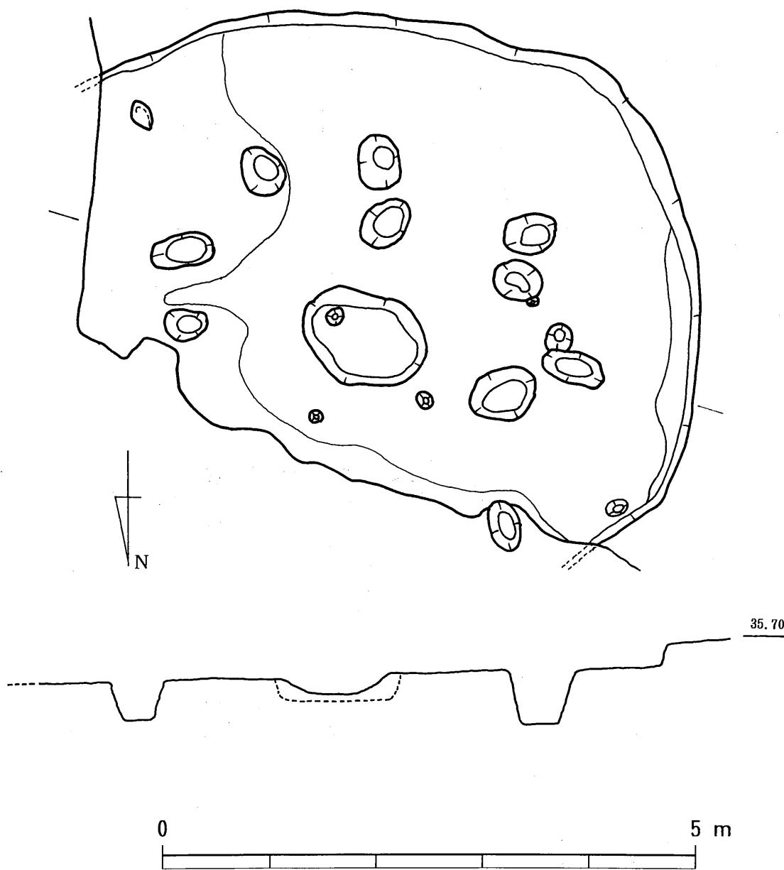
第18図 東原F地点 6号竪穴式住居 (SA-6) 実測図 (S=1/50)
