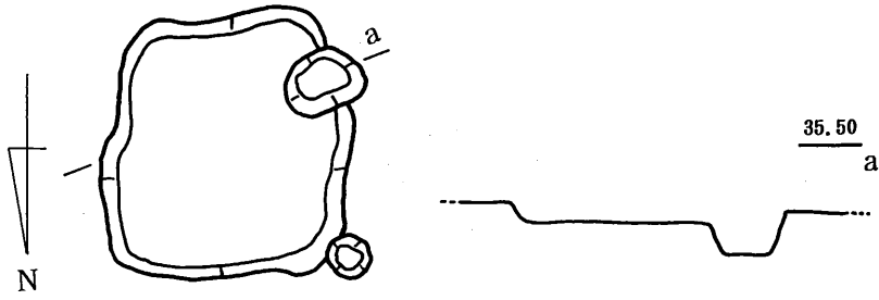
第62图 東京F地点 4号土壙(SC-3)実測図 (S=1/50)
