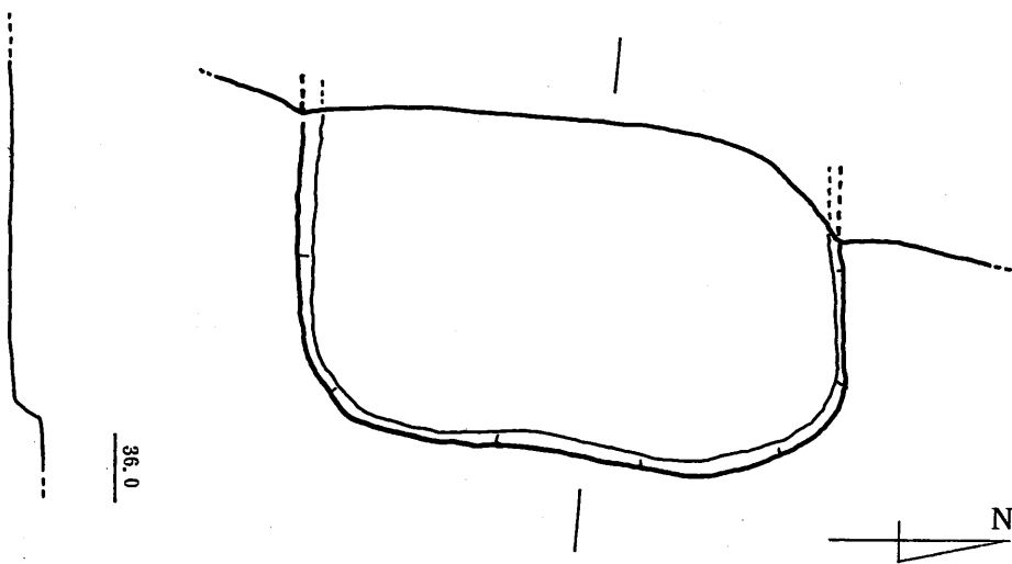
第48図 東原F地点 15号竪穴式住居 (SA-15) 実測図 (S=1/50)
