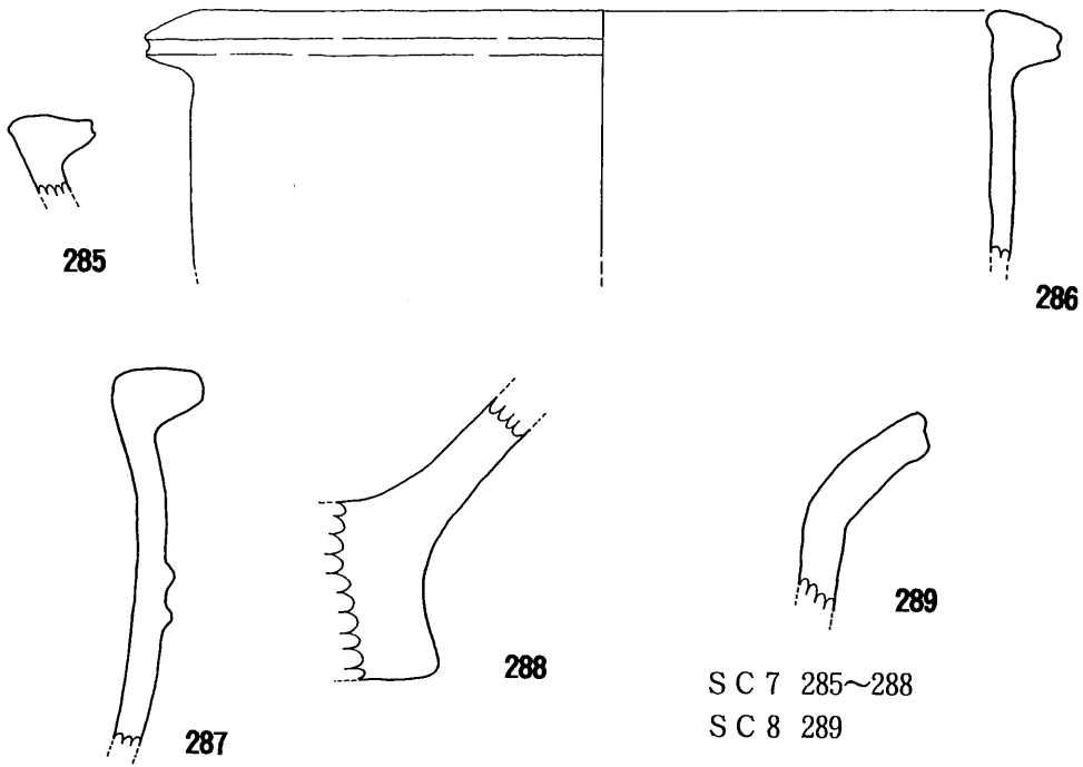
第78图 東原F地点 7・8号土壇実測出土土器片実測図
