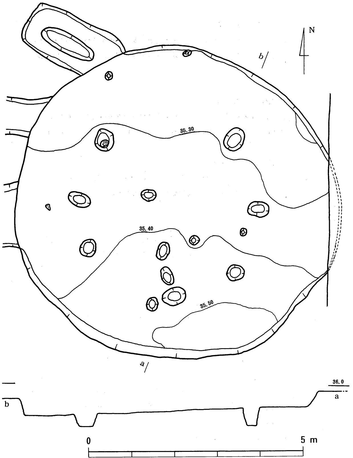
第45图 東原F地点 14号竪穴式住居 (SA-14) 実測図 (S=1/50)
