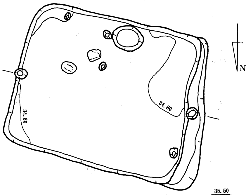
第48図 東原F地点 15号竪穴式住居 (SA-15) 実測図 (S=1/50)
