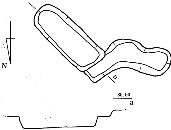
第59图 東原F地点 1号土壇(SC-1)実測図 (S=1/50)
