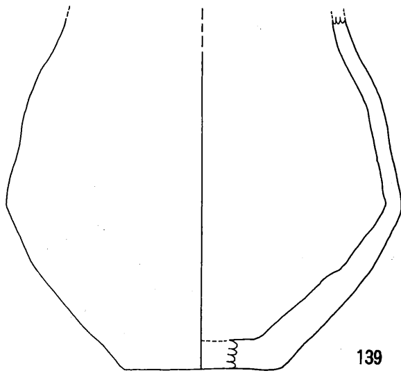
第32图 東原F地点 9号竪穴式住居出土土器片实测图(2)
