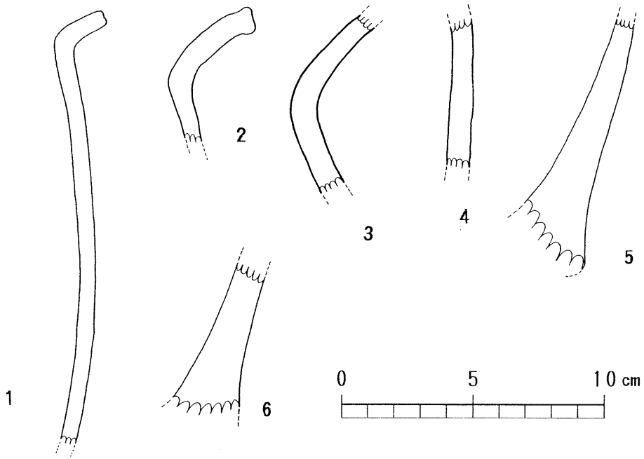
第7图 東原F地点 1号竖穴式住居出土土器片実測图
