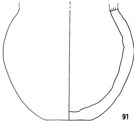
第25图 東原F地点 7号竖穴式住居出土土器片实测图(2)
