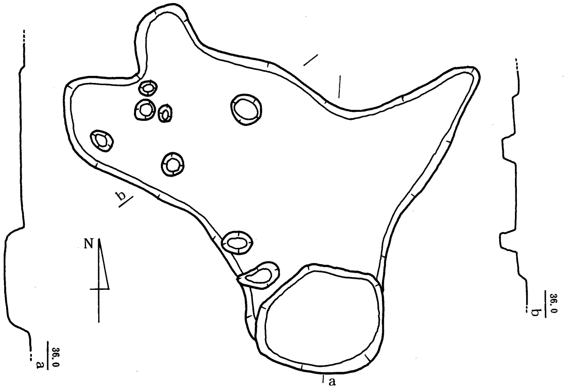
第69図 東原F地点 11号土壇(SC-3)実測図 (S=1/50)
