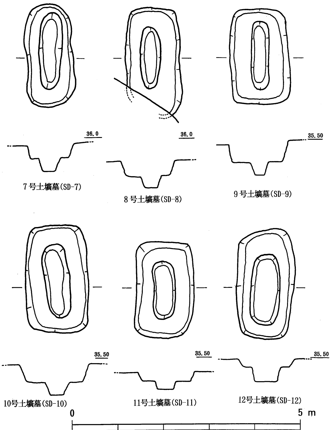
第83图 東原F地点 土墳墓実測図(2) (S=1/50)
