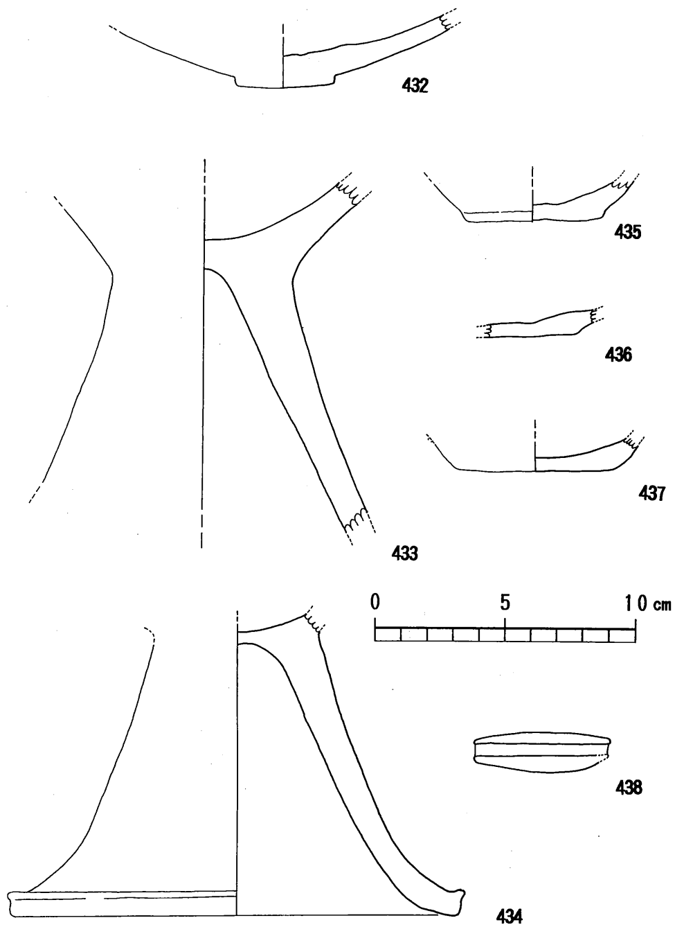
第94図 東原F地点 遺構に伴わない土器片実測図(7)
