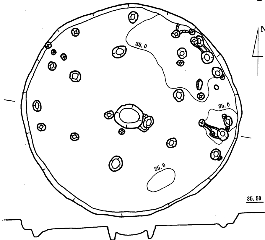
第54図 東原F地点 18号竪穴式住居 (SA-18) 実測図 (S=1/50)
