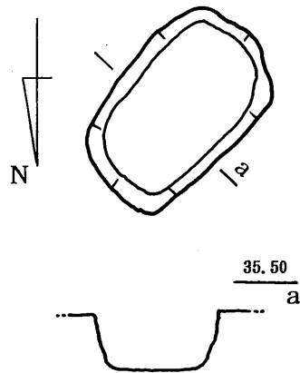
第61图 3号土壇(SC-3)実測図 (S=1/50)
