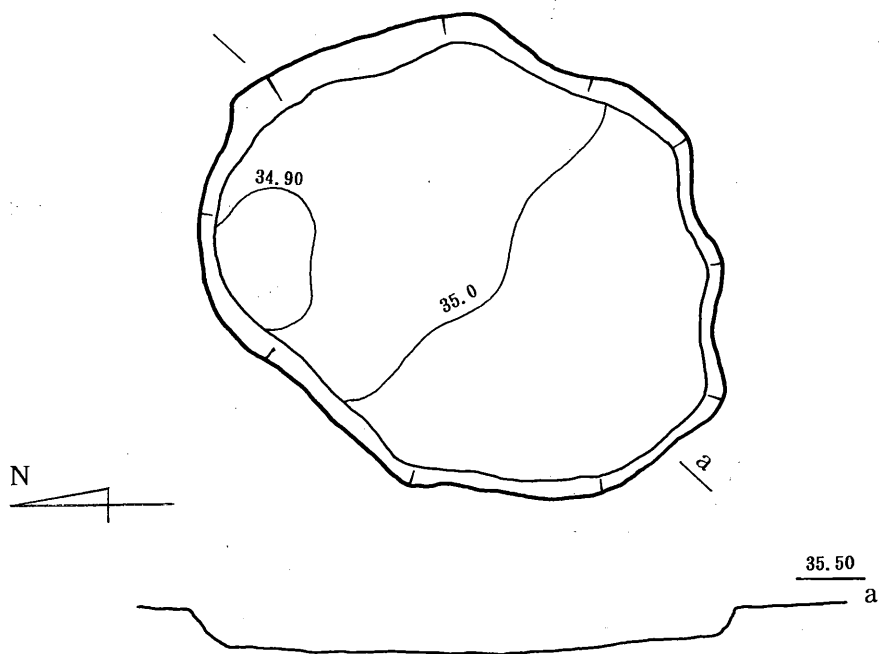
第30图 東原F地点 10号竪穴式住居 (SA-10) 実測図 (S=1/50)
