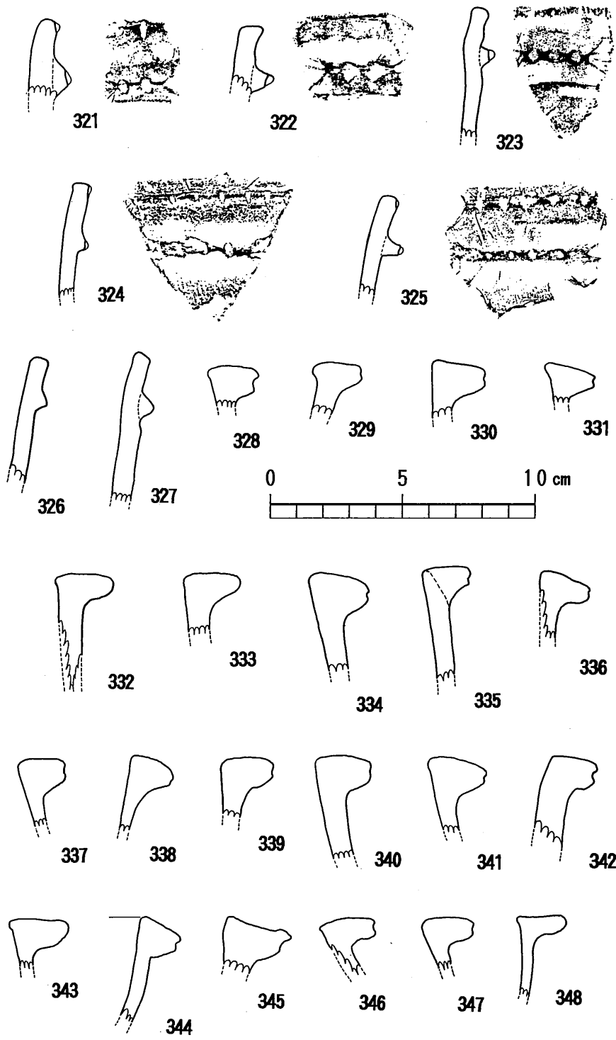
第88図 東原F地点 遺構に伴わない土器片実測図(1)
