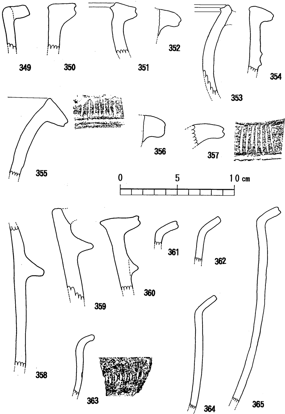
第89図 東原F地点 遺構に伴わない土器片実測図(2)
