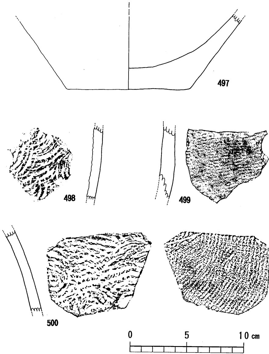
第101図 東原F地点 遺構に伴わない陶磁器片実測図(4)
