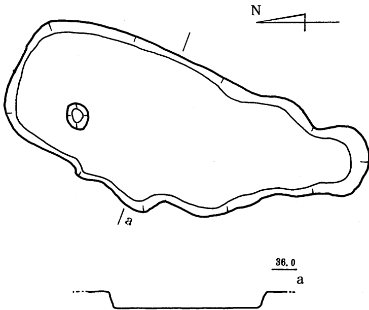
第68图 東原F地点 10号土壤(SC-3)実測図 (S=1/50)
