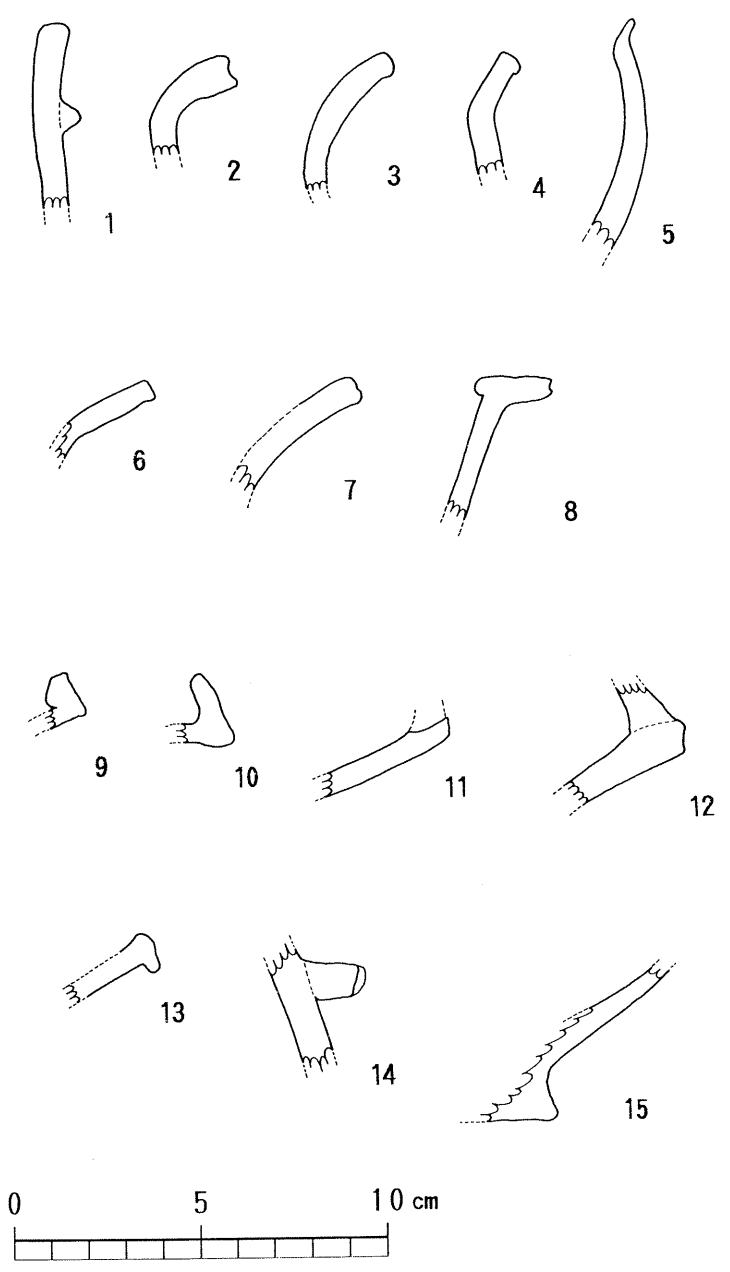
第4图 東原E地点 出土土器片实测图
