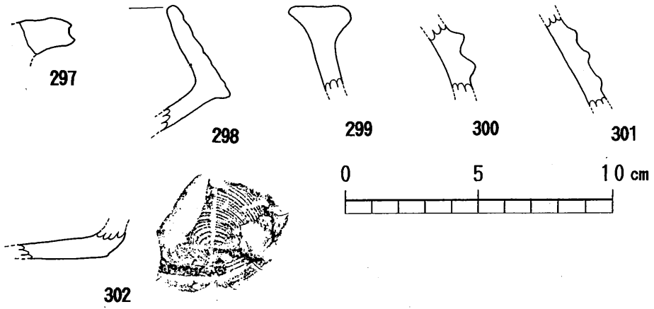
第80图 東原F地点 12号土壤实测出土土器片实测图
