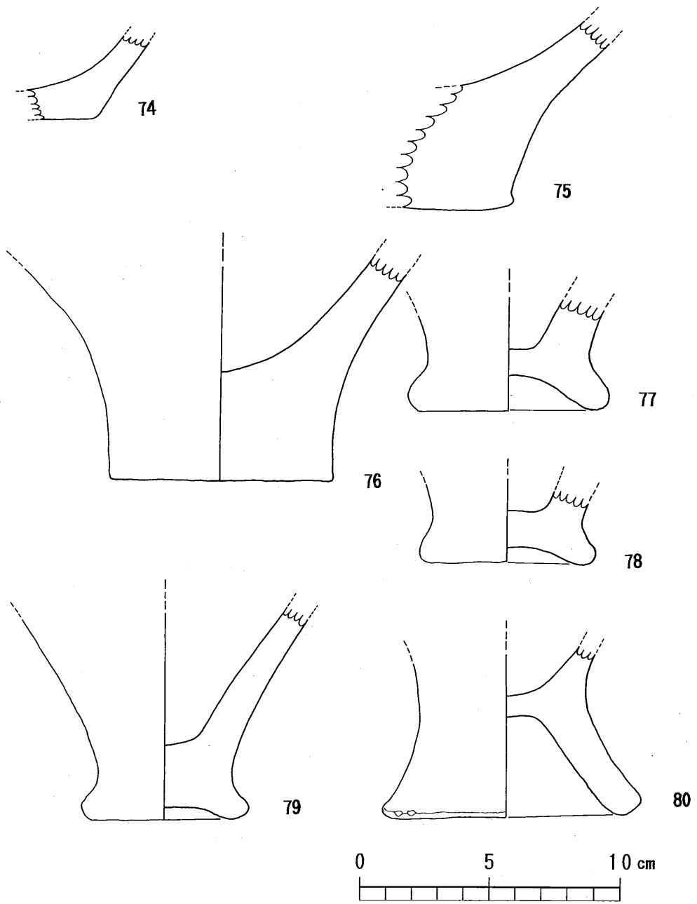
第21图 東原F地点 6号竪穴式住居出土土器片实测图(4)
