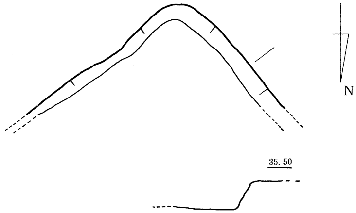
第5图 東原F地点 1号竖穴式住居 (SA-1) 实测图 (S=1/50)
