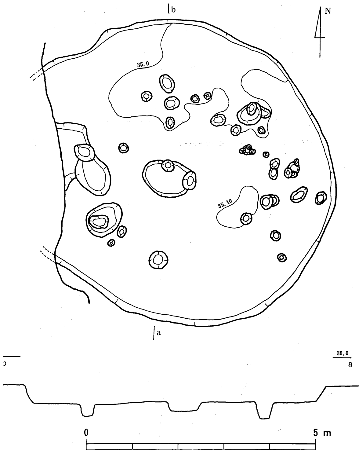
第35図 東原F地点 11号竪穴式住居 (SA-11) 実測図 (S=1/50)
