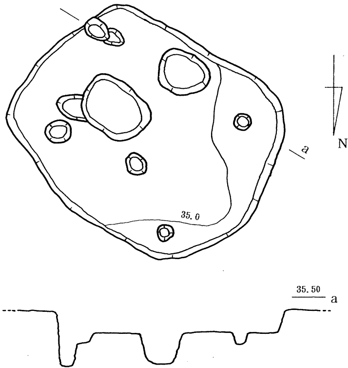
第6图 東原F地点 2号竖穴式住居 (SA-2) 实测图 (S=1/50)
