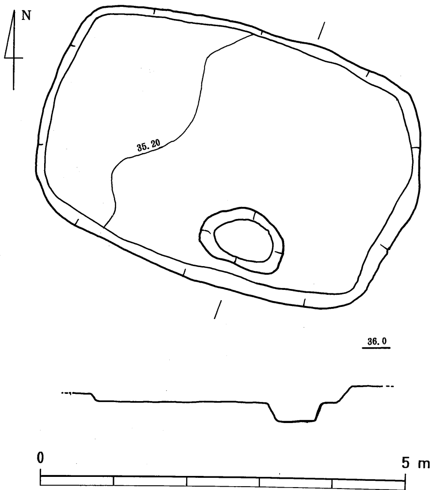
第41图 東原F地点 12号竪穴式住居 (SA-12) 実測図 (S=1/50)
