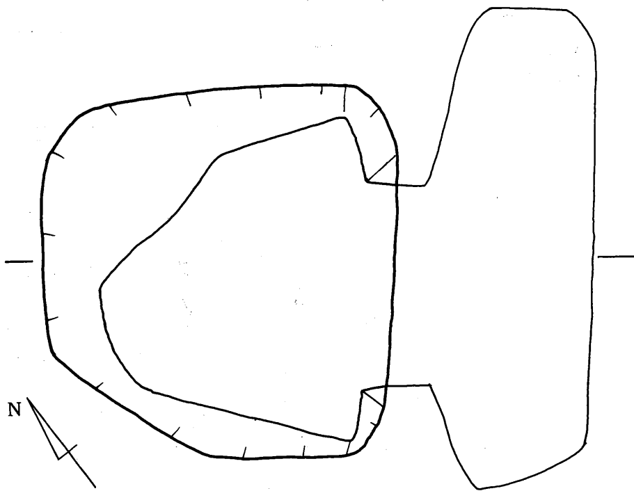
第85図 東原F地点 地下式横穴墓 (C2グリッド) 実測図
