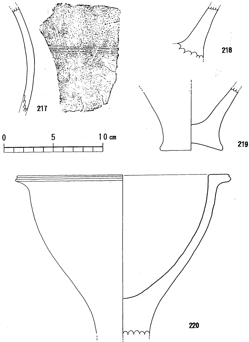
第52图 東原F地点 16号竪穴式住居出土土器片実測图(2)
