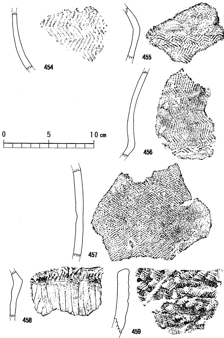
第96図 東原F地点 遺構に伴わない縄文土器片実測図(2)
