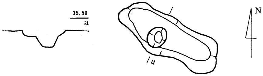
第65图 東原F地点 7号土壇(SC-3)実測図 (S=1/50)
