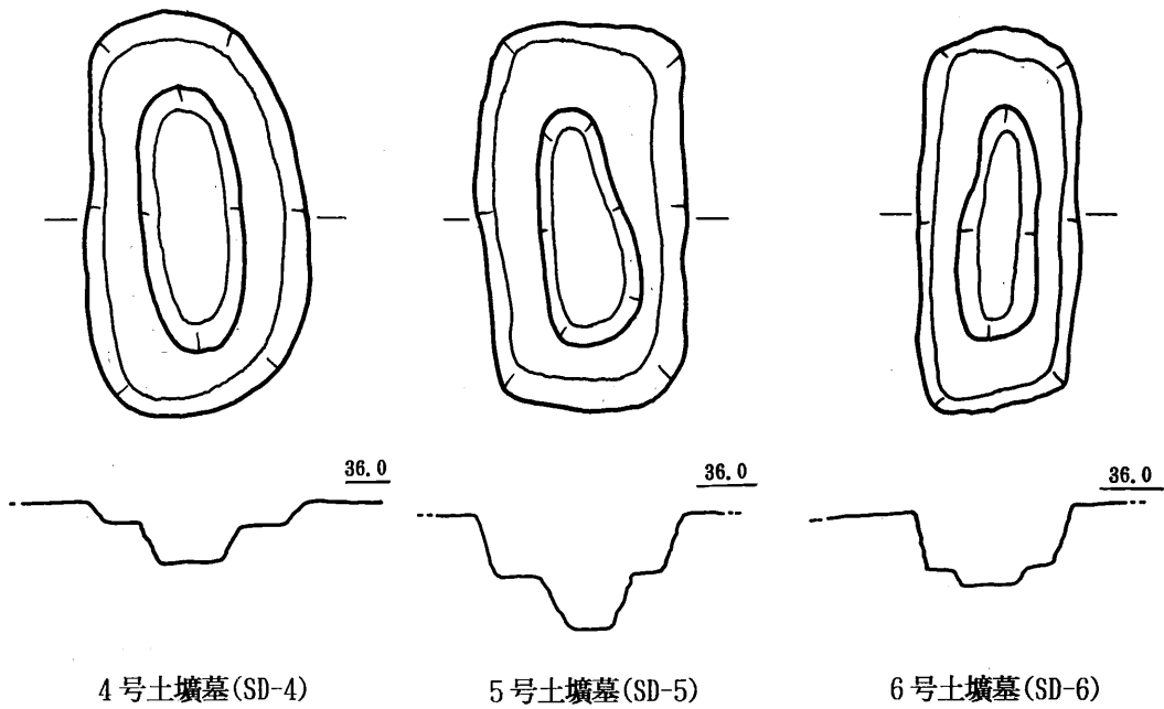
第82图 東原F地点 土墳墓实测图(1) (S=1/50)
