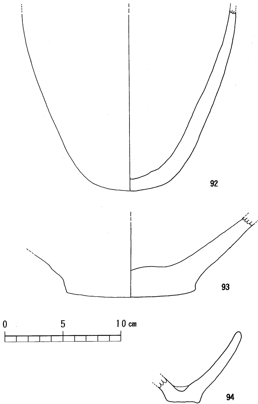
第26图 東原F地点 7号竪穴式住居出土土器片実測図(3)
