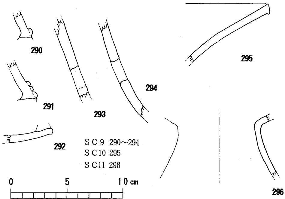
第79图 東原F地点 9・10・11号土壇実測出土土器片実測図
