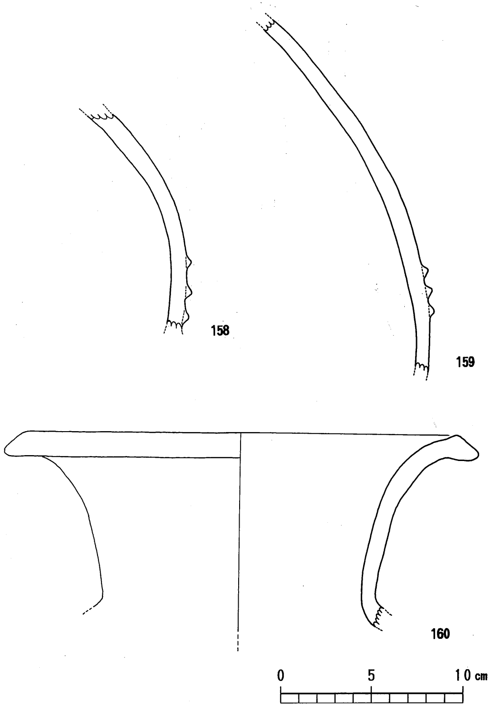
第37图 東原F地点 11号竪穴式住居出土土器片実測图(3)
