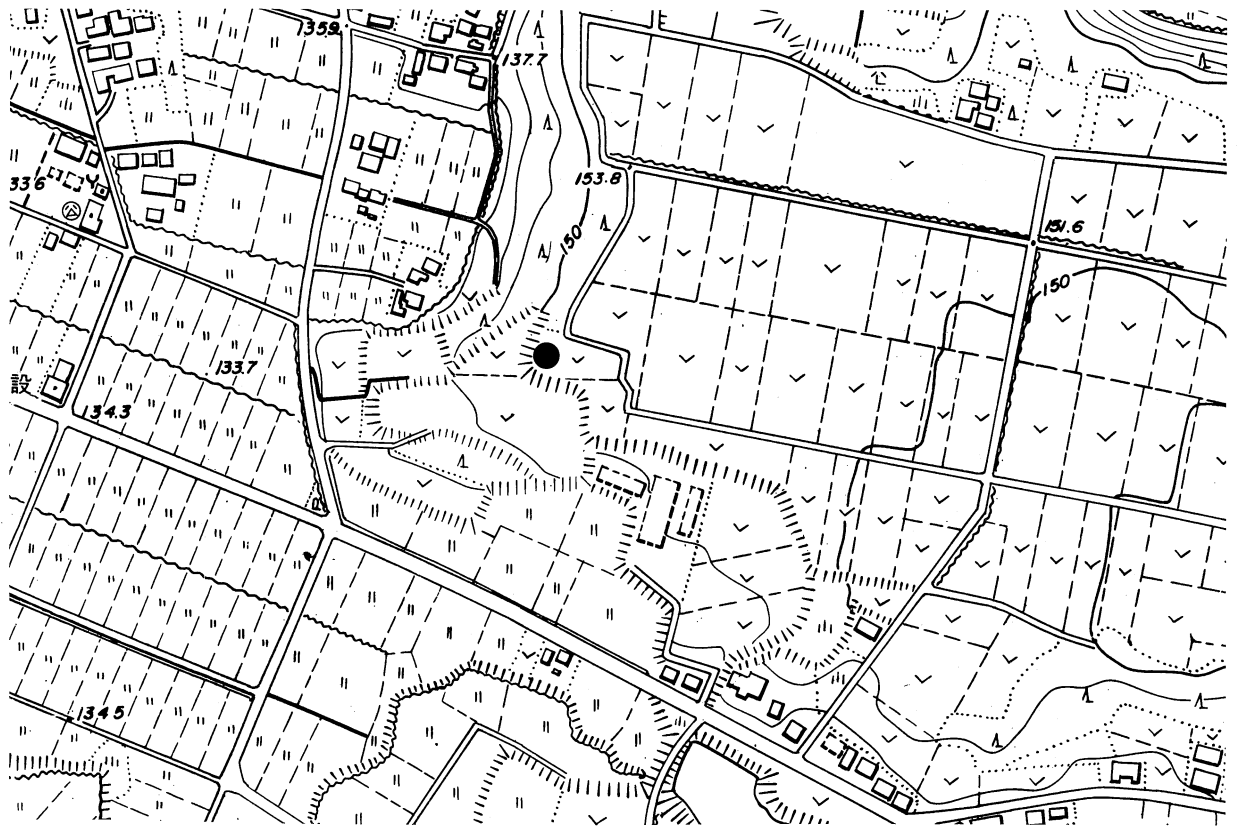
第11図 石山高取原地下式横穴墓地形図(1/5,000)
