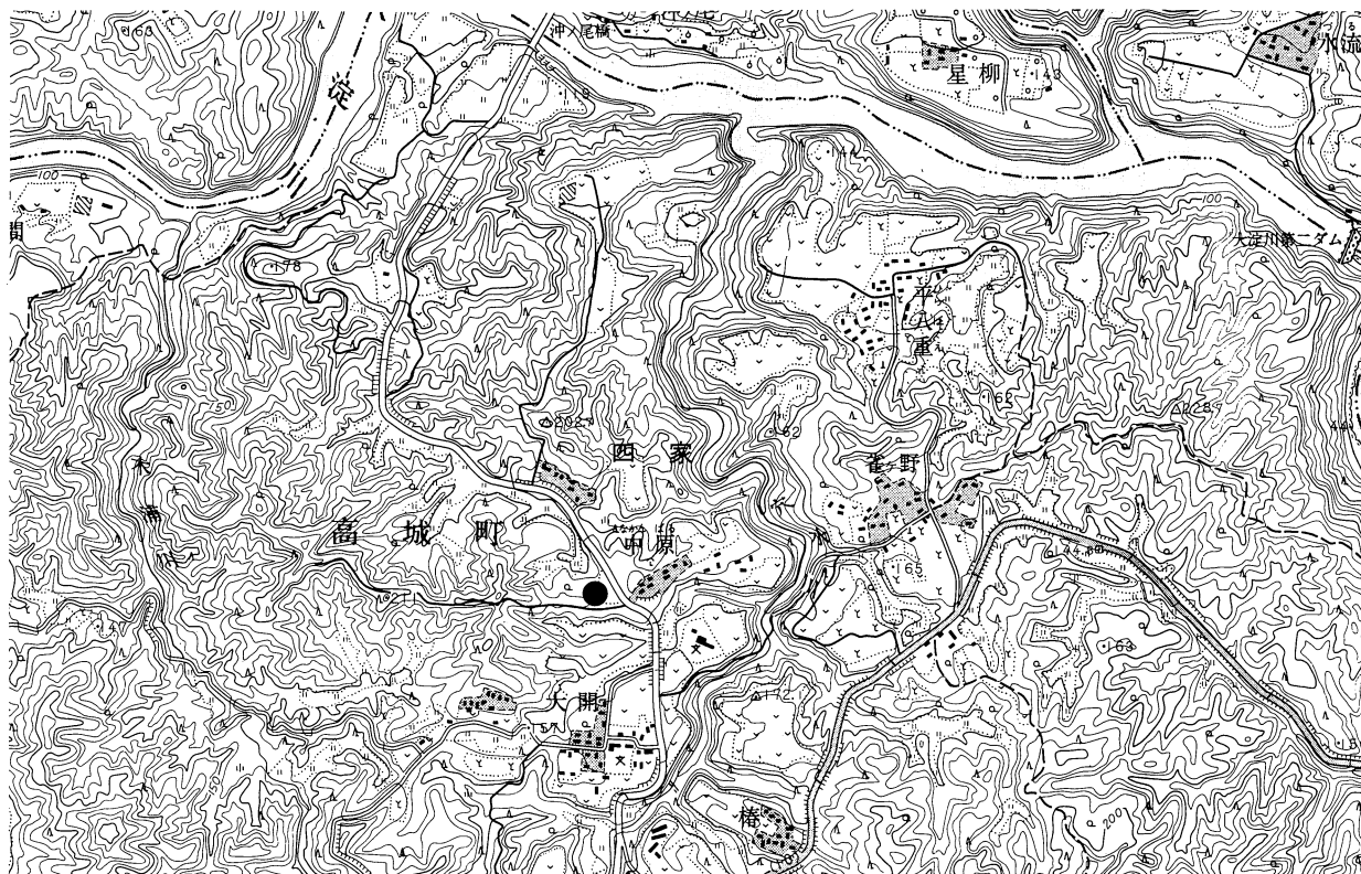
第2図 株イー・アール・シー高城産業廃棄物最終処分場建設予定地位置図(1/25,000)
