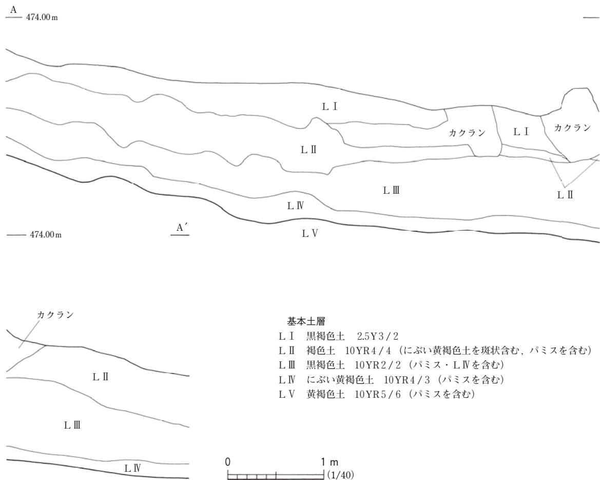
図3 基本土層図
